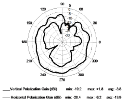
SN01—EUT vertical
