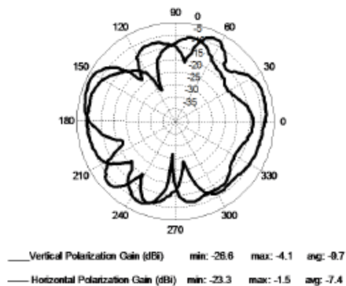
SN01—EUT vertical
