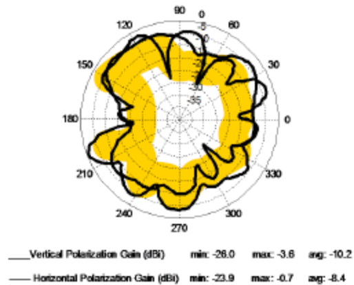
SN01—EUT side
