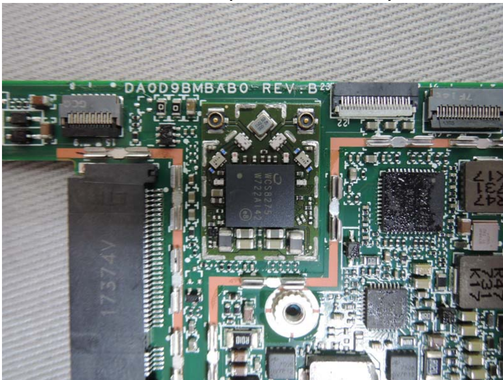
WLAN (Main) / BT / WLAN (Aux) Antenna
