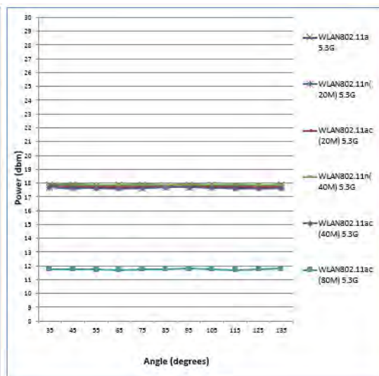
5.3GHz Aux(SISO)
