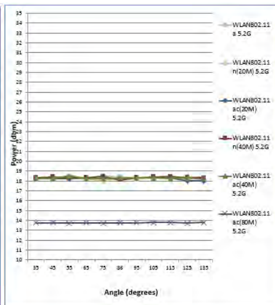
5.2GHz Aux(SISO)
