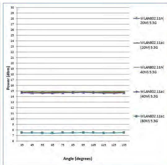
5.3GHz Aux(MIMO)
