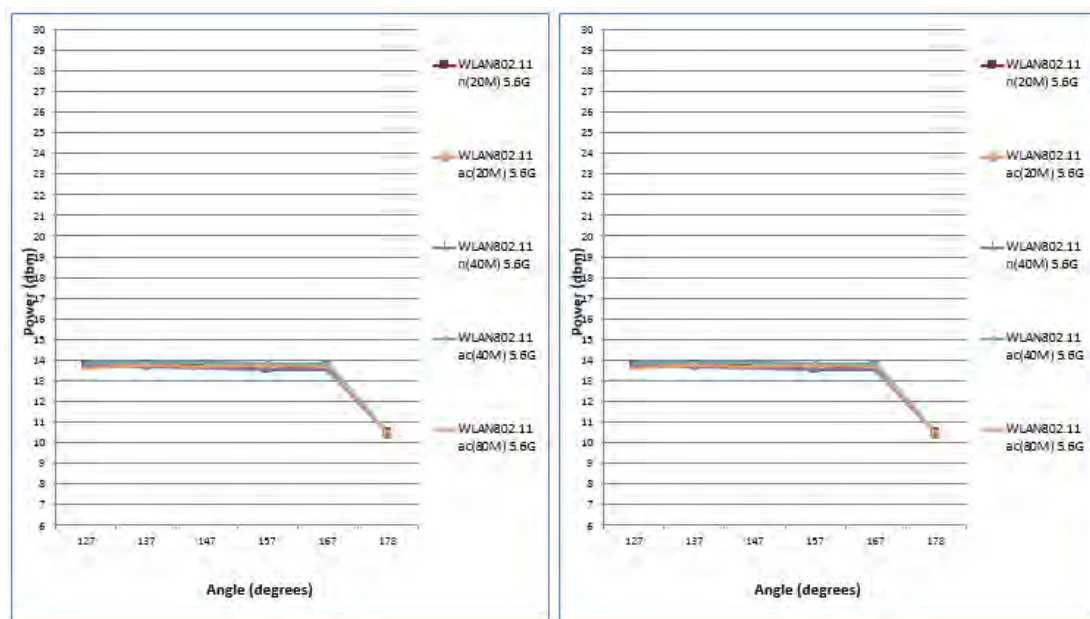
5.6GHz Main(MIMO)
