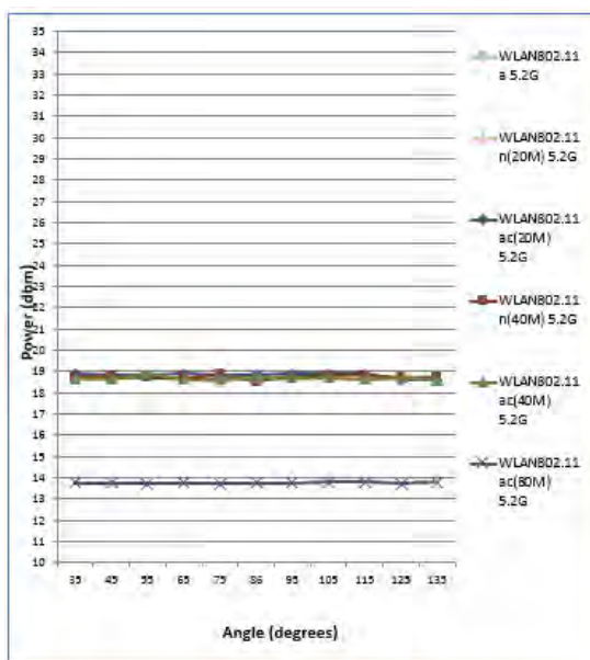
5.2GHz Main(SISO)
