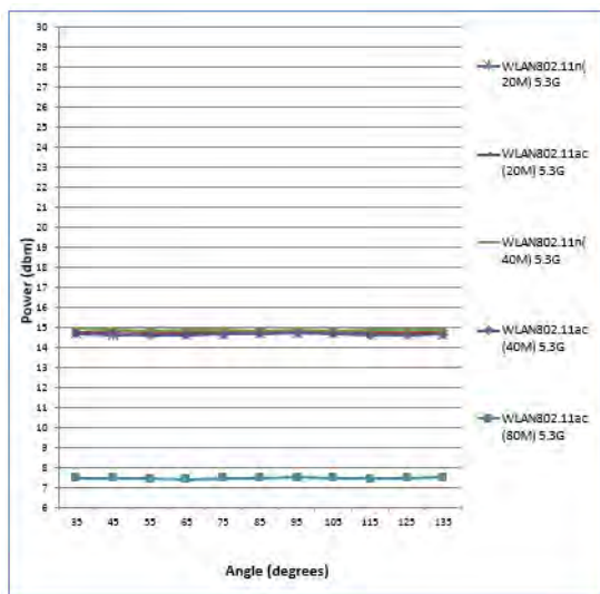
5.3GHz Main(MIMO)
