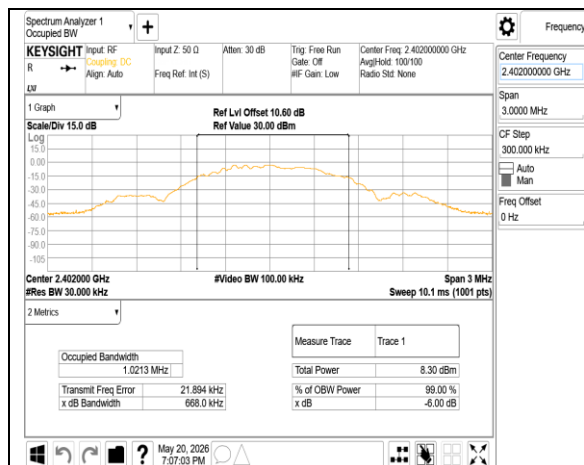
IC OBW_BLE 1M_LowCH00-2402MHz
