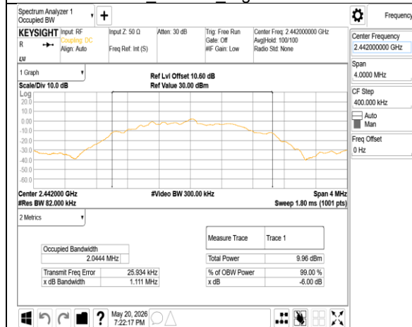
IC OBW_BLE 2M_MidCH20-2442MHz
