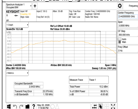
OBW_BLE 2M_MidCH20-2442MHz
