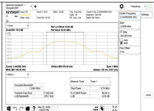
OBW_BLE 1M_MidCH20-2442MHz
