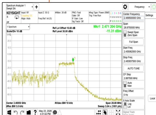
802.11be_20MHz_Chain0_2462MHz_RU52_40
