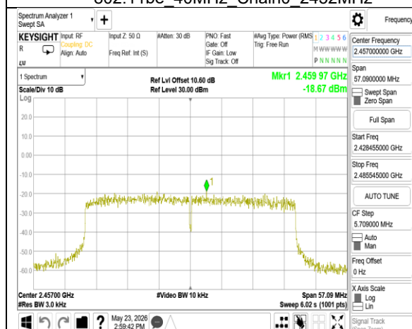
802.11be 40MHz Chain0 2457MHz
