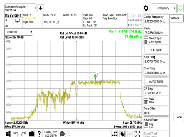
802.11be 20MHz Chain1 2472MHz 106+26 MRU2
