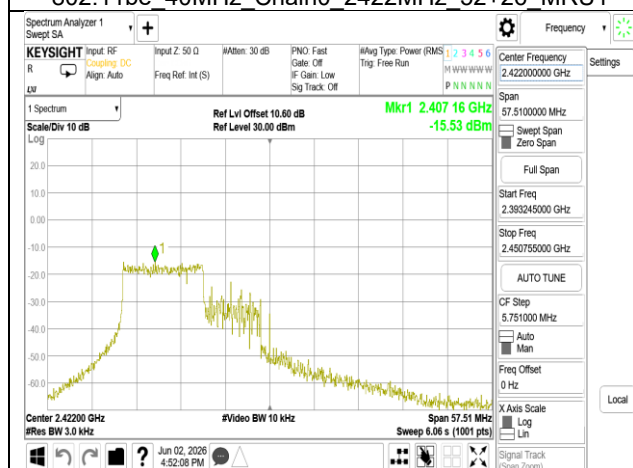
802.11be 40MHz Chain0 2422MHz 106+26 MRU1
