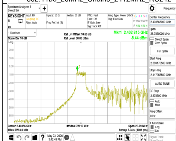
802.11be 20MHz Chain0 2412MHz RU26_0
