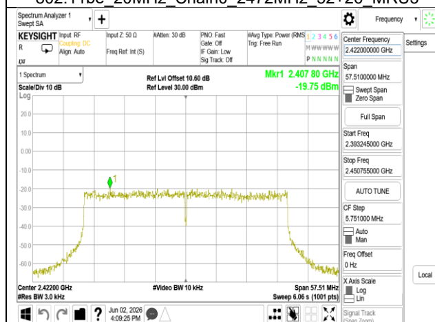
802.11be 40MHz Chain0 2422MHz RU484
