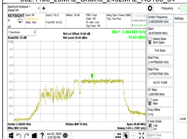
802.11be_20MHz_Chain0_2462MHz_106+26_MRU2
