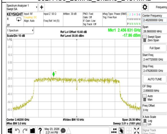
802.11be 20MHz Chain0 2462MHz
