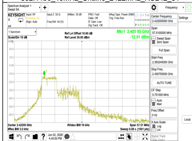
802.11be 40MHz Chain0 2422MHz 52+26 MRU1
