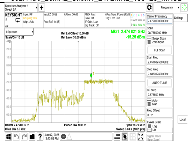
802.11be 20MHz Chain1 2472MHz 52+26 MRU3
