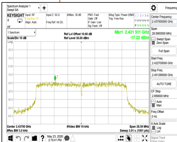
802.11be 20MHz Chain0 2437MHz
