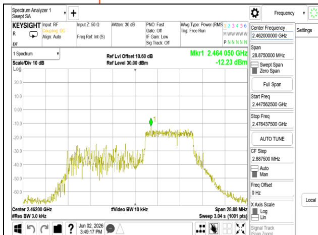
802.11be 20MHz Chain0 2462MHz 52+26 MRU3
