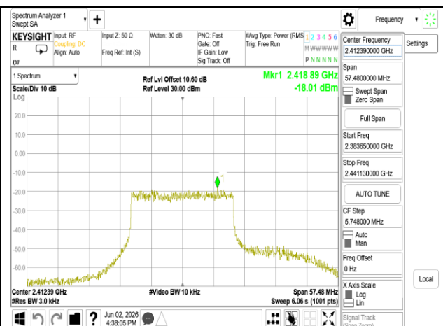
802.11be 40MHz Chain1 2422MHz RU242 61
