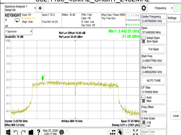
802.11be 40MHz Chain1 2457MHz
