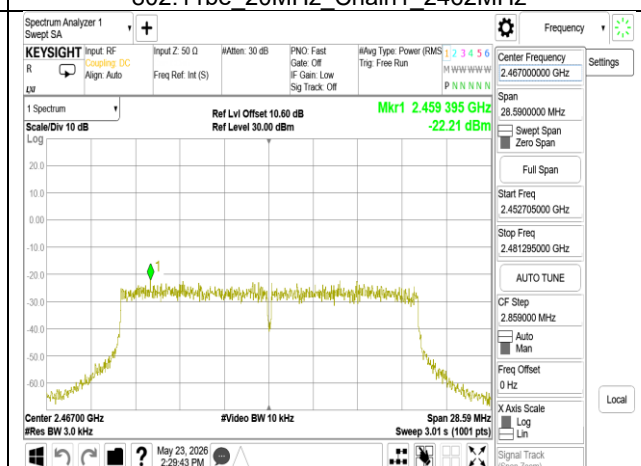
802.11be 20MHz Chain1 2467MHz
