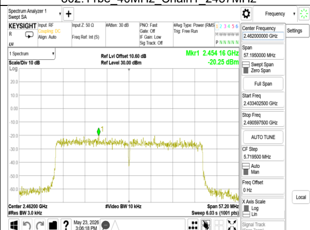
802.11be 40MHz Chain1 2462MHz
