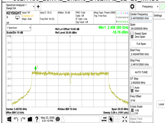
802.11be 20MHz Chain0 2467MHz RU242
