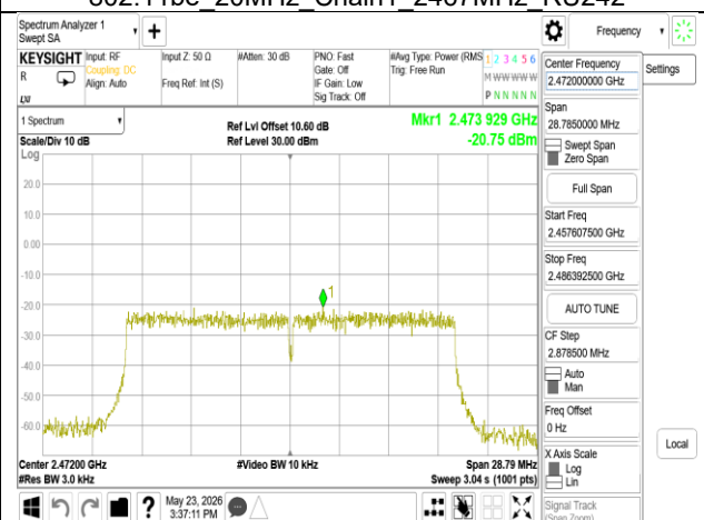
802.11be 20MHz Chain1 2472MHz RU242
