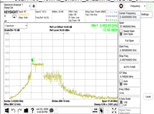
802.11be 40MHz Chain1 2422MHz 52+26 MRU1
