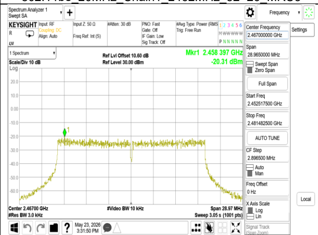
802.11be 20MHz Chain1 2467MHz RU242
