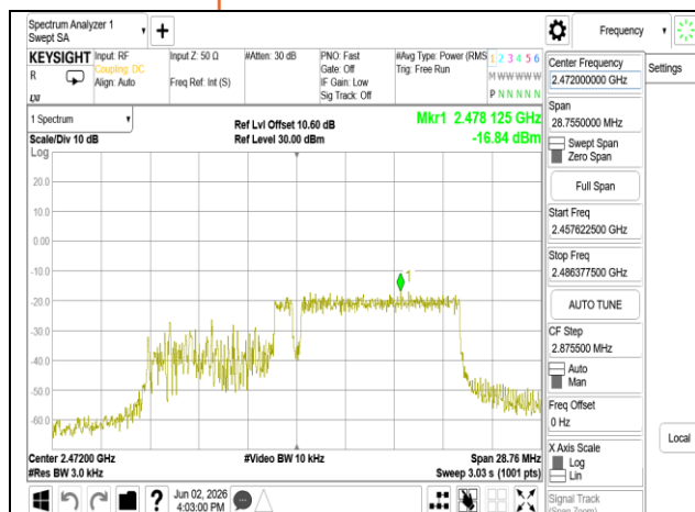
802.11be 20MHz Chain0 2472MHz 106+26 MRU2
