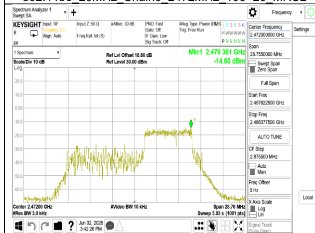
802.11be 20MHz Chain0 2472MHz 52+26 MRU3
