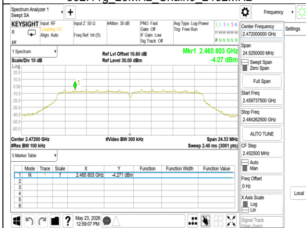
802.11g_20MHz_Chain0_2472MHz
