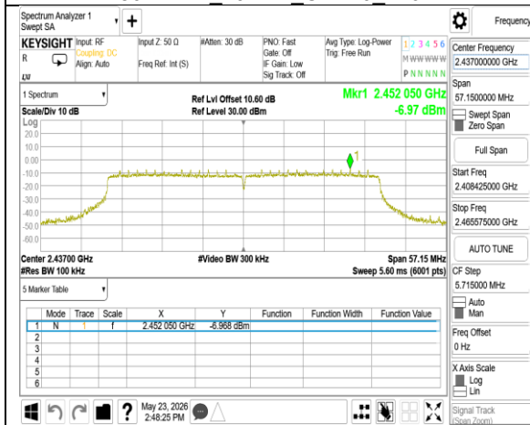
802.11be 40MHz Chain1 2437MHz
