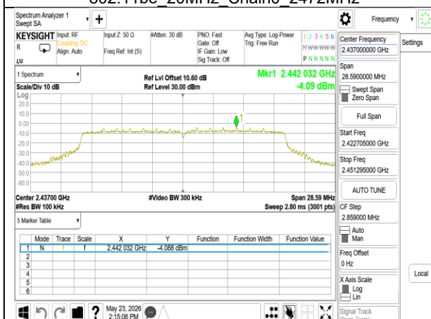
802.11be 20MHz Chain1 2437MHz
