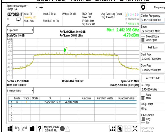
802.11be 40MHz Chain1 2457MHz
