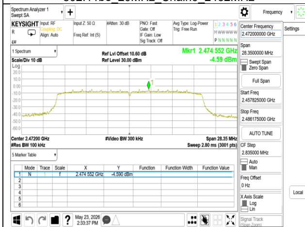
802.11be 20MHz Chain0 2472MHz
