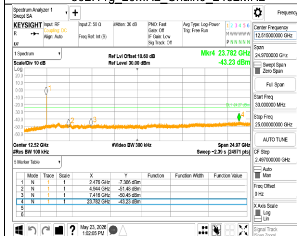
802.11g_20MHz_Chain0_2472MHz
