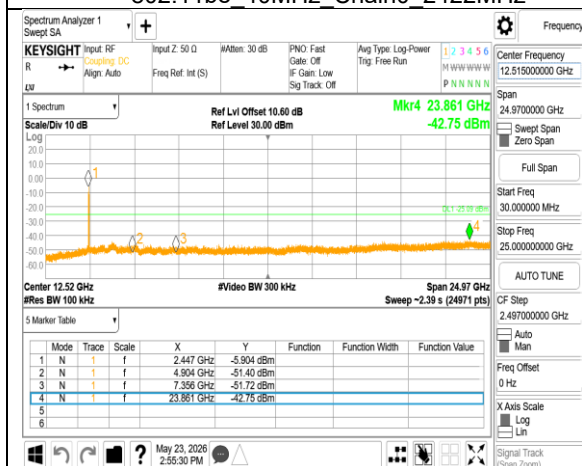
802.11be_40MHz_Chain0_2452MHz
