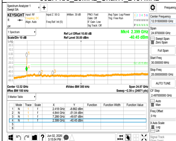
802.11be_40MHz_Chain0_2422MHz
