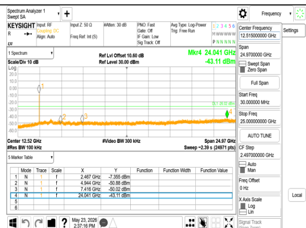
802.11be_20MHz_Chain1_2472MHz
