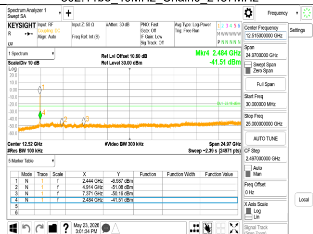
802.11be_40MHz_Chain0_2457MHz
