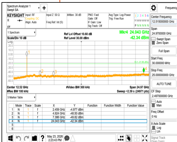
802.11be_20MHz_Chain0_2462MHz
