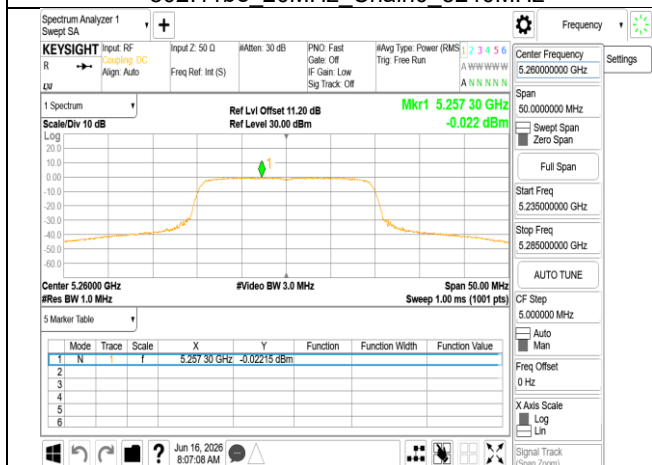
802.11be_20MHz_Chain0_5260MHz
