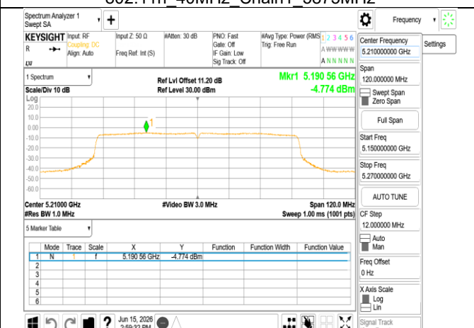
802.11ac_80MHz_Chain1_5210MHz
