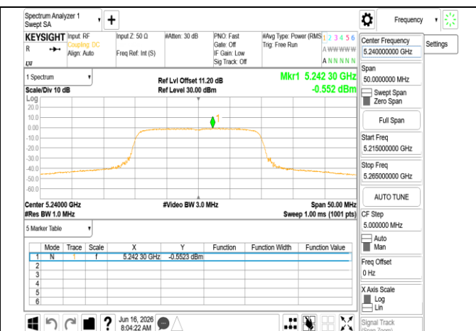
802.11be_20MHz_Chain1_5240MHz
