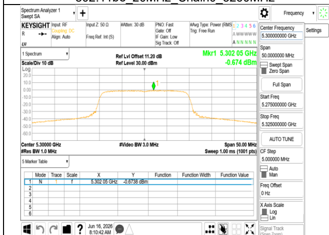
802.11be_20MHz_Chain0_5300MHz
