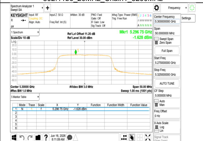
802.11be_20MHz_Chain1_5300MHz
