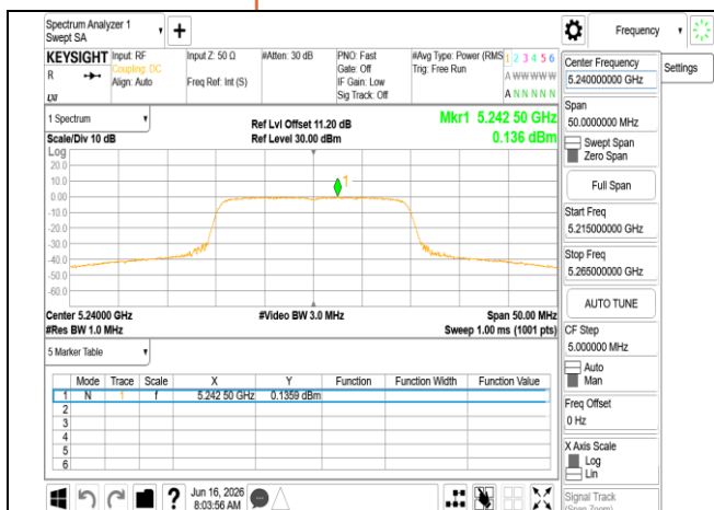
802.11be_20MHz_Chain0_5240MHz
