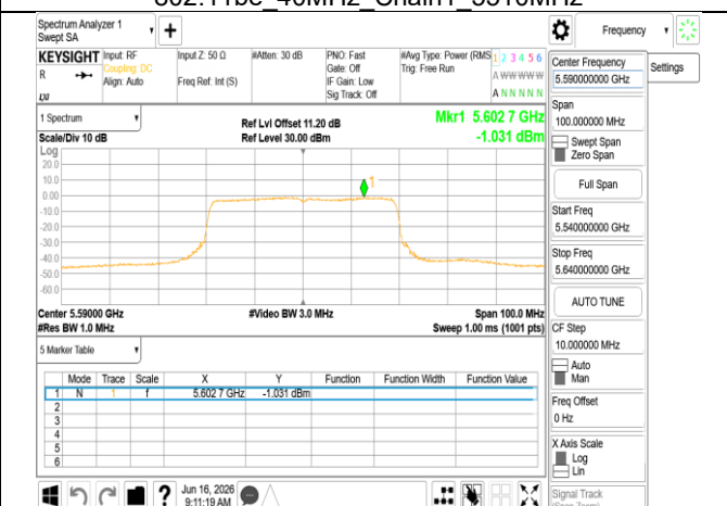
802.11be 40MHz Chain1 5590MHz
