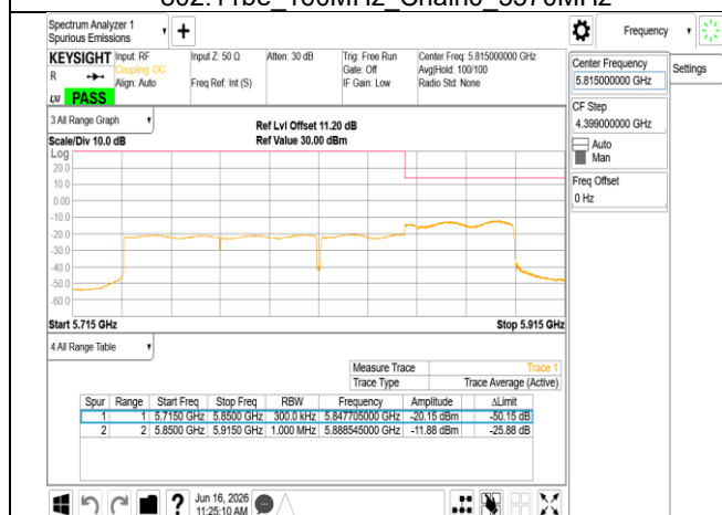
802.11be_160MHz_Chain0_5815MHz_UNII 4
