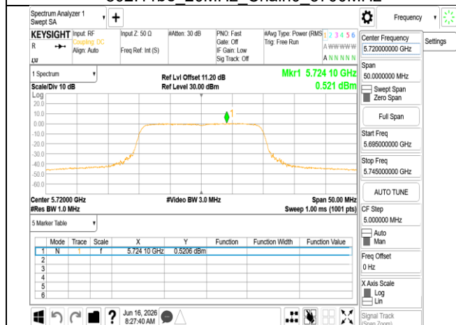
802.11be_20MHz_Chain0_5720MHz_UNII 2C
