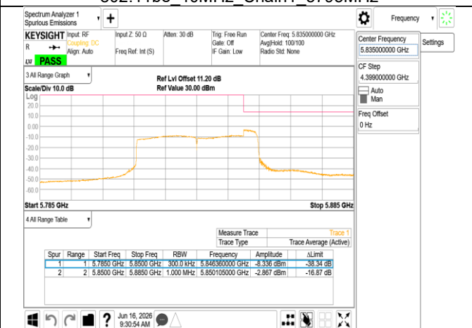
802.11be 40MHz Chain1_5835MHz_UNII 4
