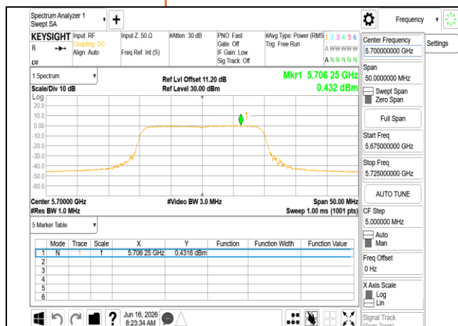
802.11be_20MHz_Chain0_5700MHz
