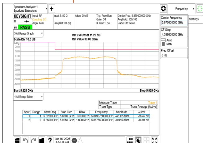
802.11be_40MHz_Chain0_5875MHz
