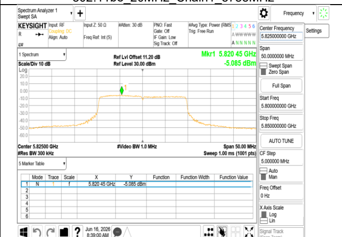
802.11be_20MHz_Chain1_5825MHz
