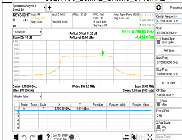
802.11be_20MHz_Chain0_5785MHz
