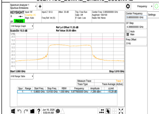
802.11be 20MHz Chain0 5885MHz
