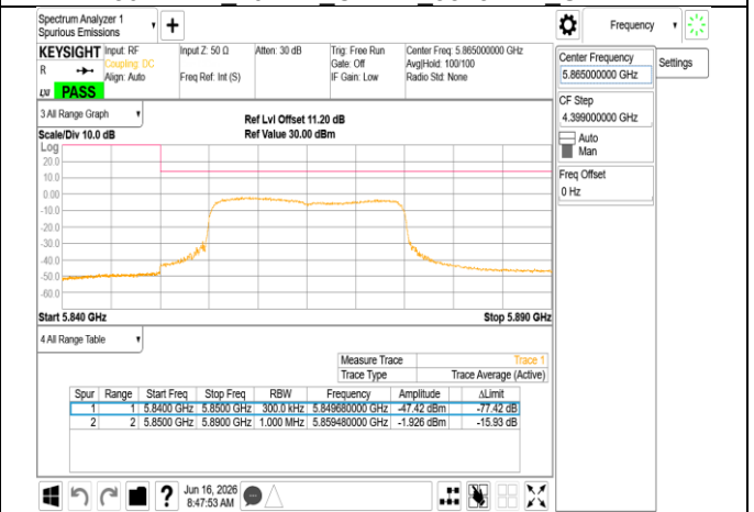
802.11be 20MHz Chain1 5865MHz
