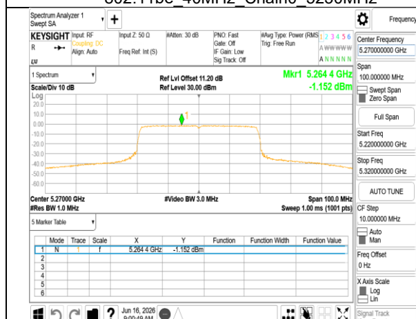
802.11be 40MHz Chain0_5270MHz
