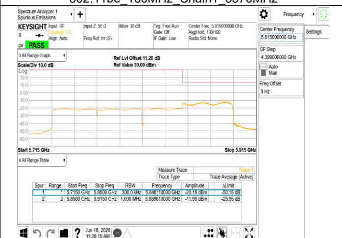
802.11be_160MHz_Chain1_5815MHz_UNII 4
