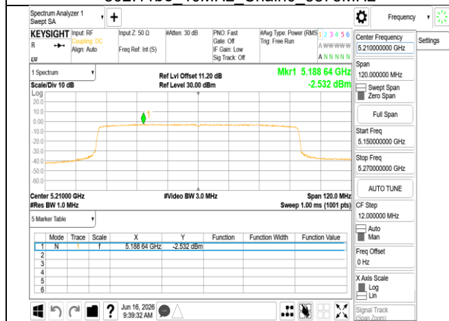
802.11be_80MHz_Chain0_5210MHz
