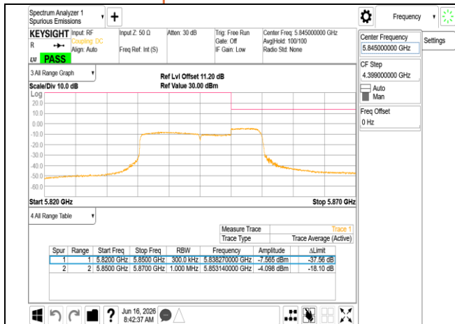
802.11be 20MHz Chain0 5845MHz UNII 4
