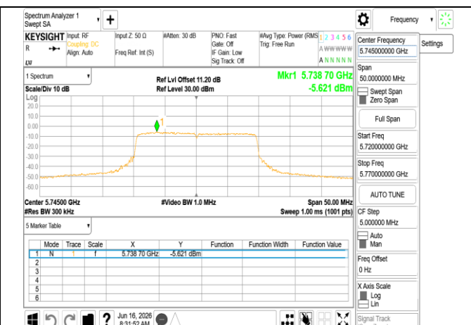
802.11be_20MHz_Chain1_5745MHz
