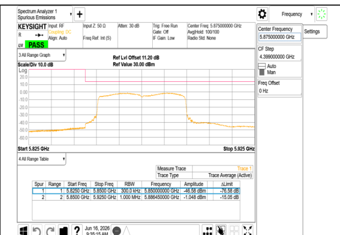
802.11be_40MHz_Chain1_5875MHz
