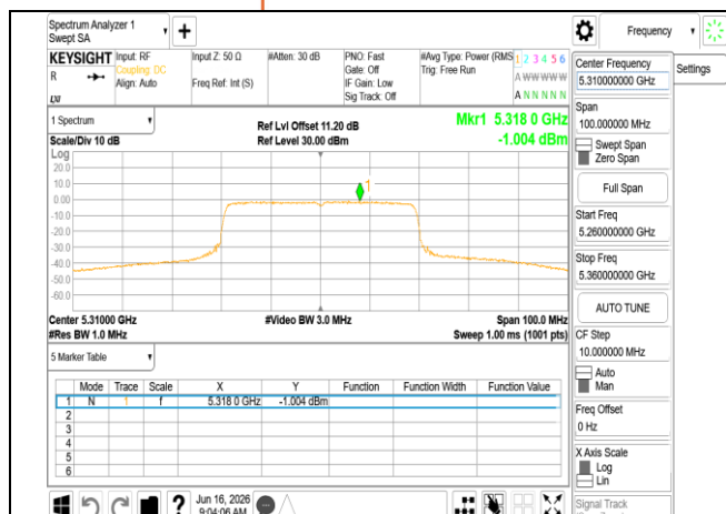
802.11be 40MHz Chain0 5310MHz
