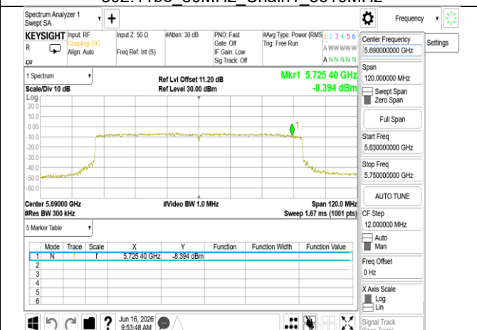
802.11be_80MHz_Chain0_5690MHz_UNII 3
