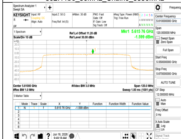
802.11be_80MHz_Chain0_5610MHz
