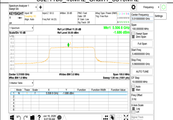
802.11be 40MHz Chain1 5510MHz
