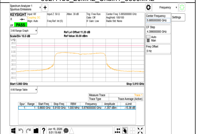
802.11be 20MHz Chain1 5885MHz
