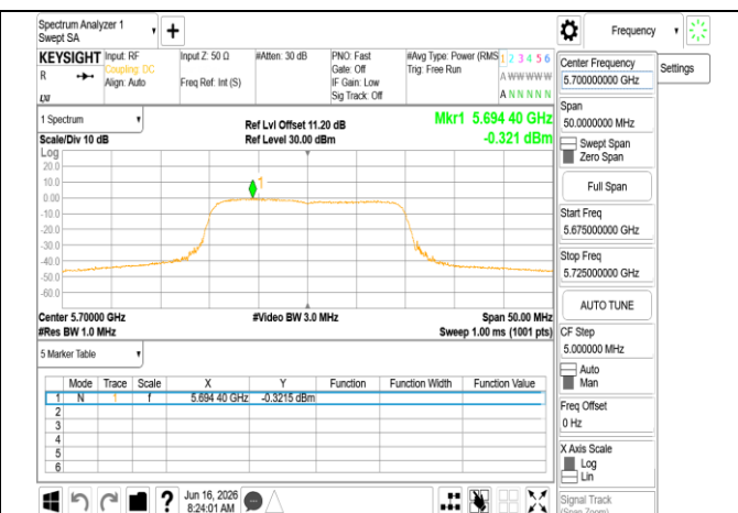
802.11be_20MHz_Chain1_5700MHz
