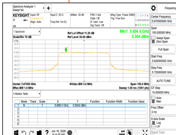
802.11be 40MHz Chain0_5670MHz
