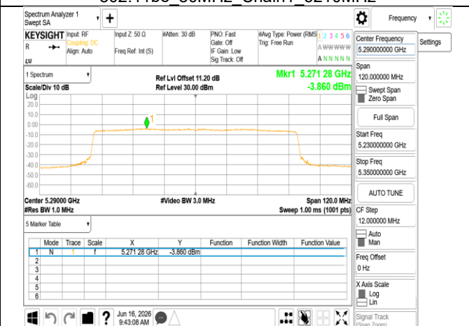
802.11be_80MHz_Chain1_5290MHz
