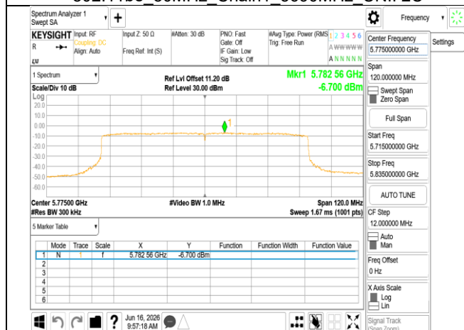
802.11be 80MHz Chain0 5775MHz
