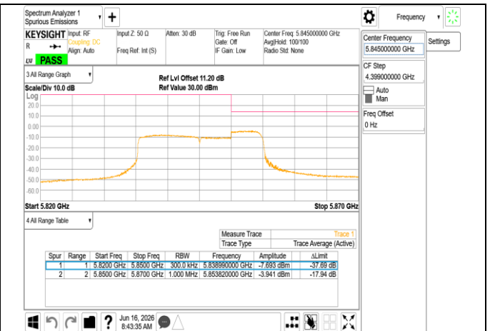
802.11be 20MHz Chain1 5845MHz UNII 4
