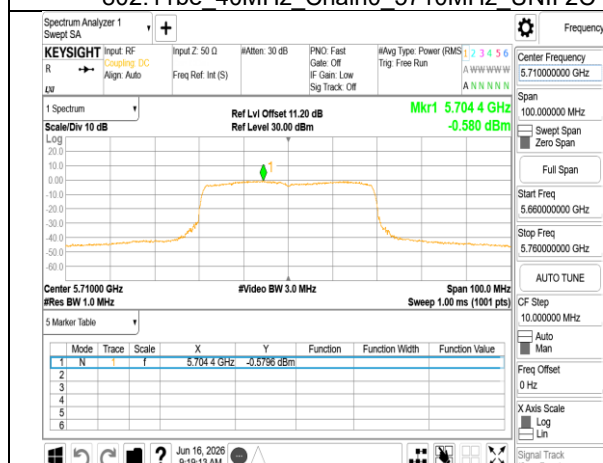
802.11be 40MHz Chain1_5710MHz UNII 2C
