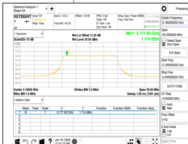
802.11be 20MHz Chain0 5180MHz RU242
