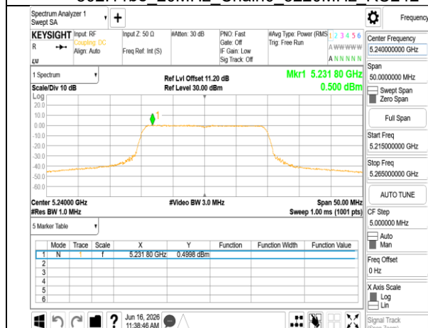
802.11be 20MHz Chain0 5240MHz RU242
