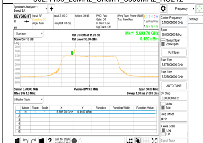
802.11be_20MHz_Chain1_5700MHz_RU242
