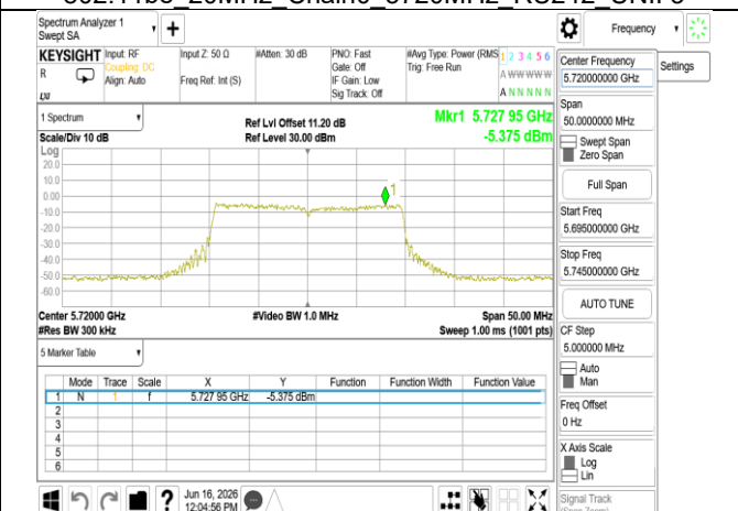
802.11be_20MHz_Chain1_5720MHz_RU242_UNII 3
