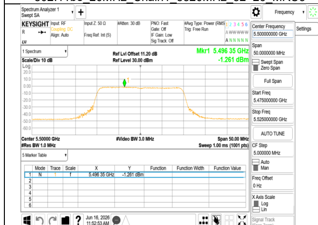
802.11be_20MHz_Chain1_5500MHz_RU242
