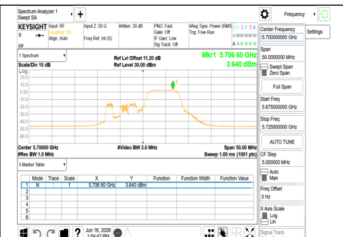
802.11be_20MHz_Chain1_5700MHz_52+26_MRU3
