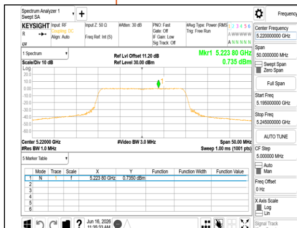
802.11be 20MHz Chain0 5220MHz RU242
