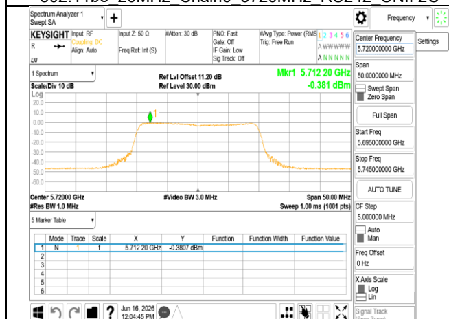
802.11be_20MHz_Chain1_5720MHz_RU242_UNII 2C
