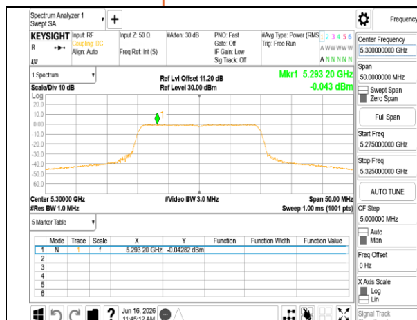
802.11be 20MHz Chain0 5300MHz RU242
