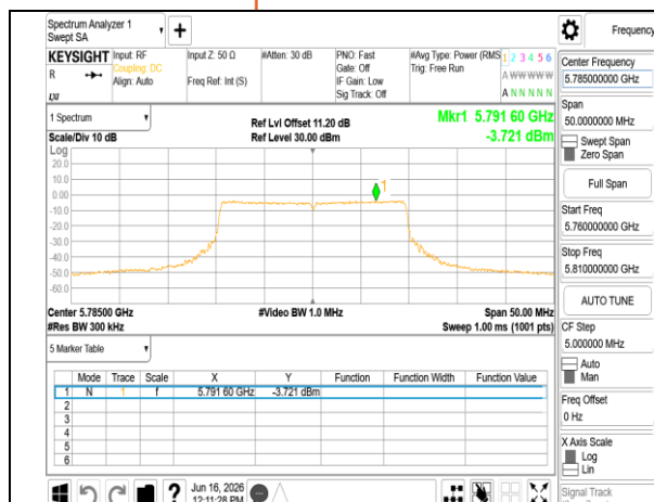
802.11be_20MHz_Chain0_5785MHz_RU242
