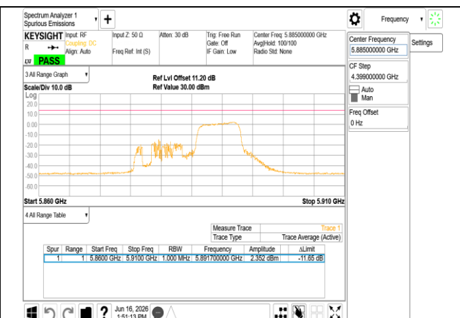
802.11be_20MHz_Chain1_5885MHz_52+26_MRU3
