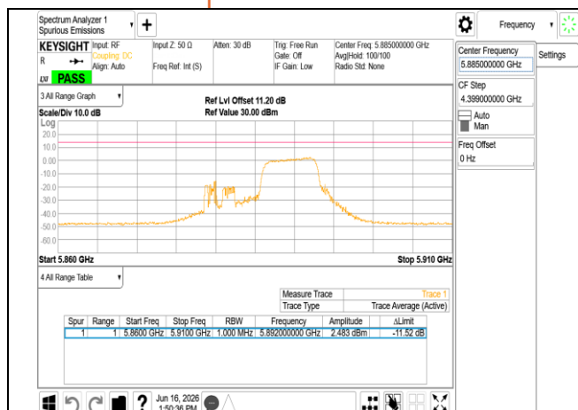
802.11be_20MHz_Chain0_5885MHz_52+26_MRU3
