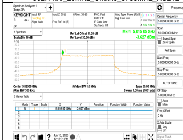
802.11be_20MHz_Chain0_5825MHz_RU242
