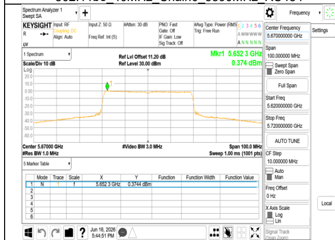
802.11be 40MHz Chain0 5670MHz RU484
