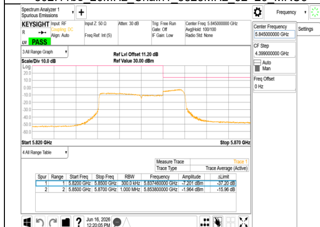
802.11be_20MHz_Chain1_5845MHz_RU242_UNII 4
