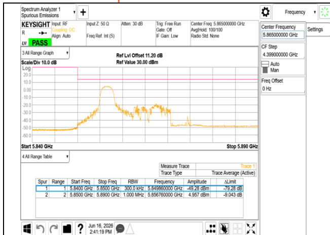
802.11be 20MHz Chain1 5865MHz RU26_0
