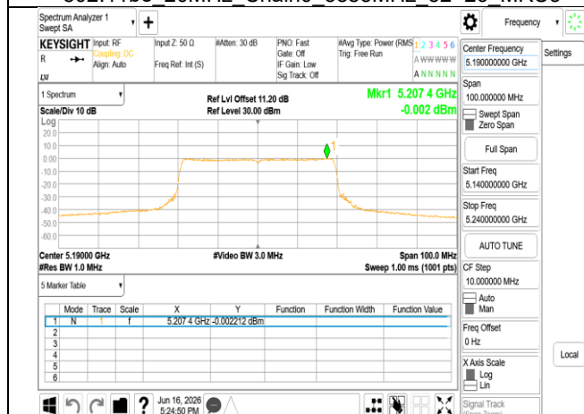
802.11be_40MHz_Chain0_5190MHz_RU484
