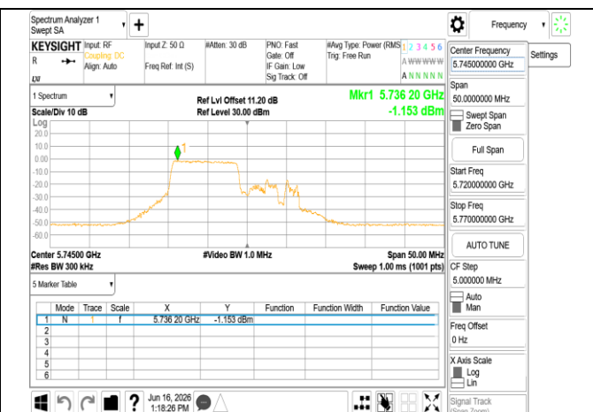
802.11be 20MHz Chain1 5745MHz RU106_53
