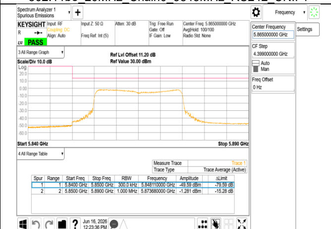
802.11be_20MHz_Chain0_5865MHz_RU242
