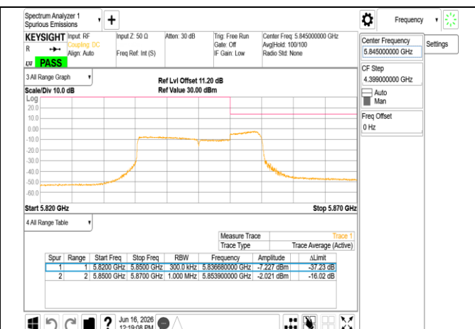
802.11be_20MHz_Chain0_5845MHz_RU242_UNII 4
