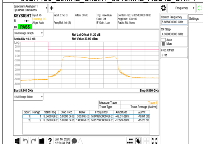
802.11be_20MHz_Chain1_5865MHz_RU242
