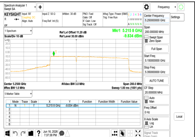
802.11be_160MHz_Chain0_5250MHz_996+484_MRU1
