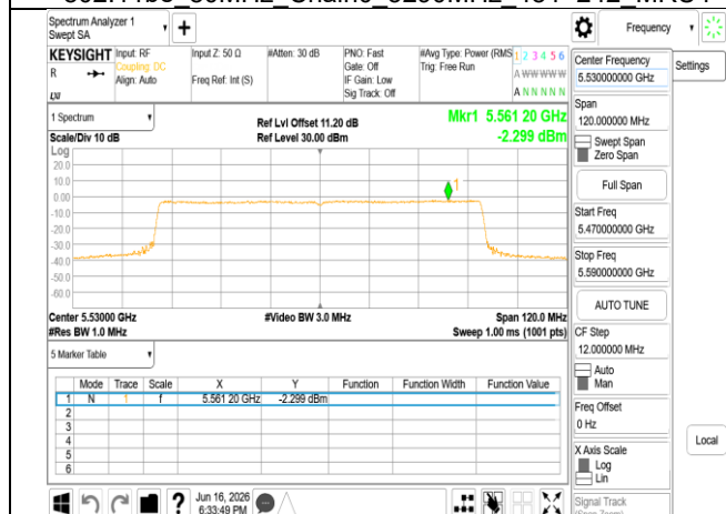
802.11be_80MHz_Chain0_5530MHz_RU996
