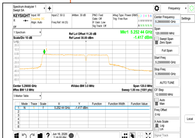
802.11be_80MHz_Chain0_5290MHz_484+242_MRU4
