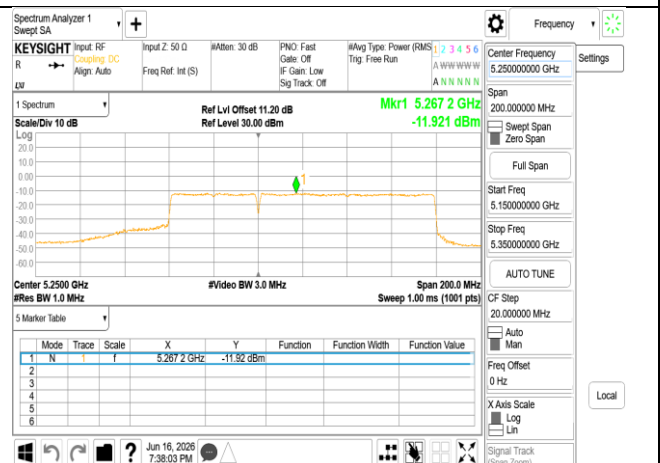
802.11be_160MHz_Chain1_5250MHz_996+484_MRU1
