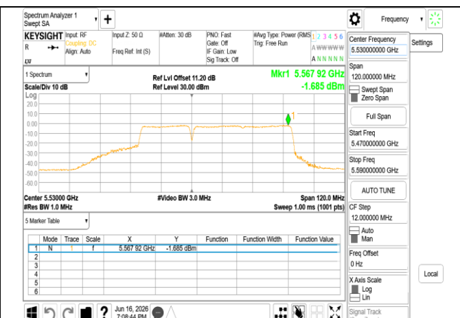
802.11be_80MHz_Chain1_5530MHz_484+242_MRU1
