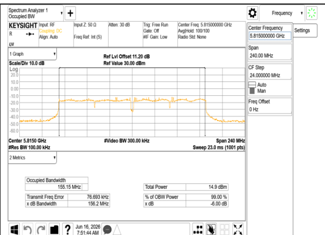
802.11ac 160MHz Chain1 5815MHz
