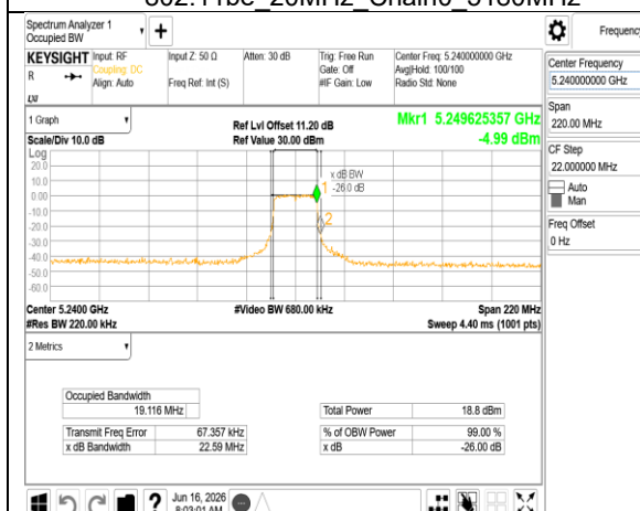
802.11be 20MHz Chain0 5240MHz
