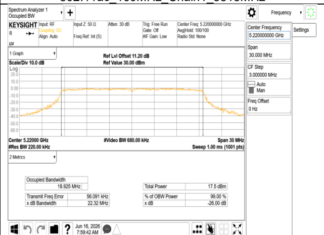
802.11be 20MHz Chain0 5220MHz
