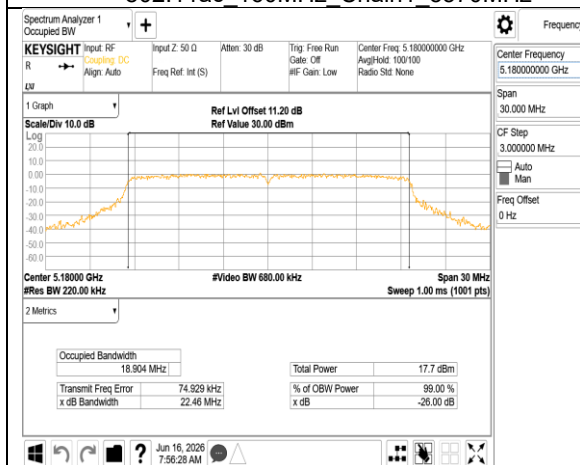
802.11be 20MHz Chain0 5180MHz
