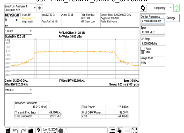
802.11be 20MHz Chain0 5260MHz
