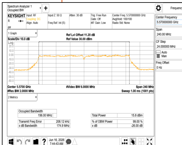
802.11ac 160MHz Chain1 5570MHz
