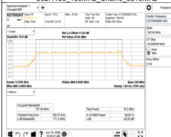
802.11be_160MHz_Chain1_5570MHz
