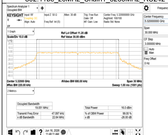
802.11be 20MHz Chain1 5320MHz RU242
