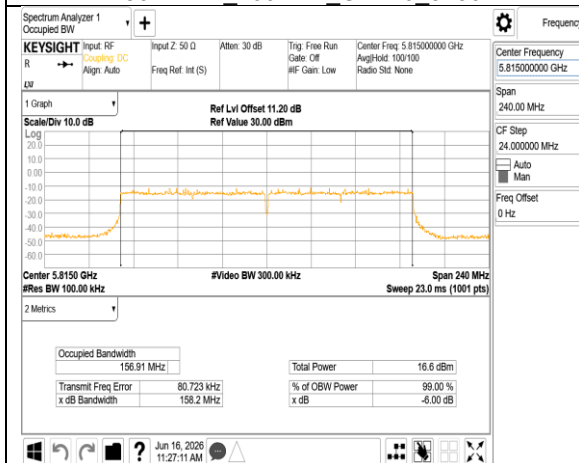
802.11be_160MHz_Chain0_5815MHz
