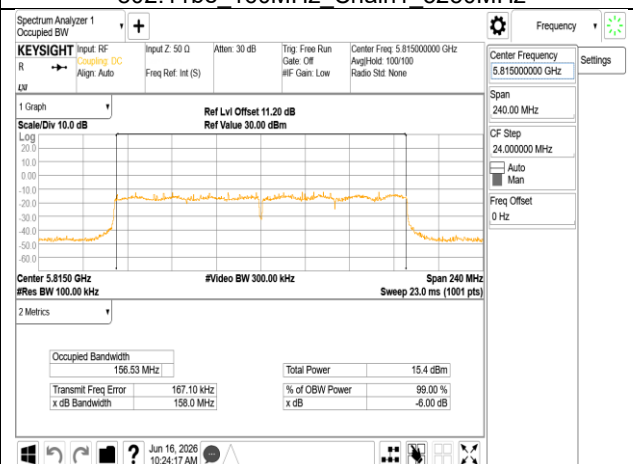
802.11be_160MHz_Chain1_5815MHz
