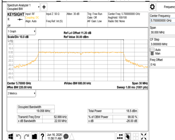
802.11be_20MHz_Chain0_5700MHz_RU242
