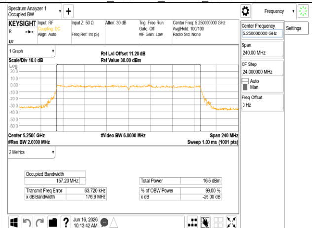
802.11be_160MHz_Chain1_5250MHz
