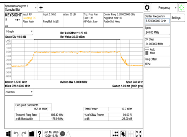
802.11be_160MHz_Chain0_5570MHz
