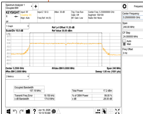
802.11be_160MHz_Chain0_5250MHz
