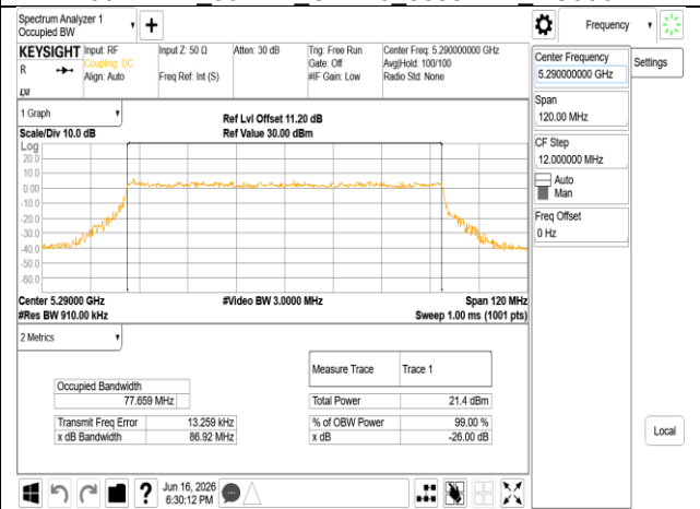
802.11be 80MHz Chain1 5290MHz RU996
