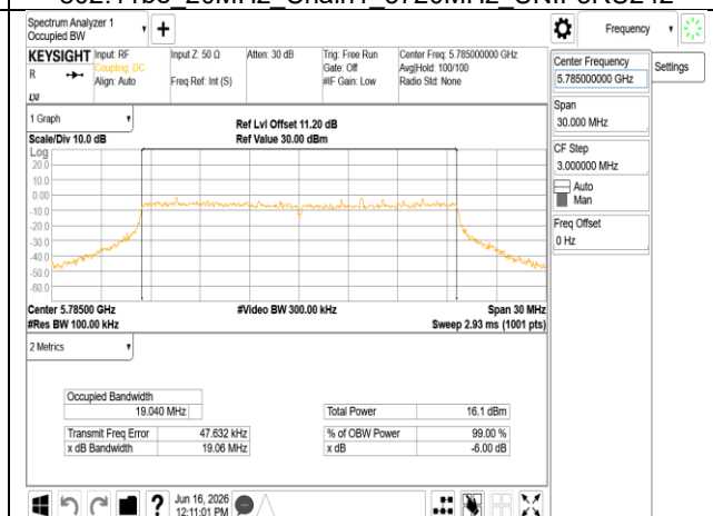
802.11be 20MHz Chain1 5785MHz RU242
