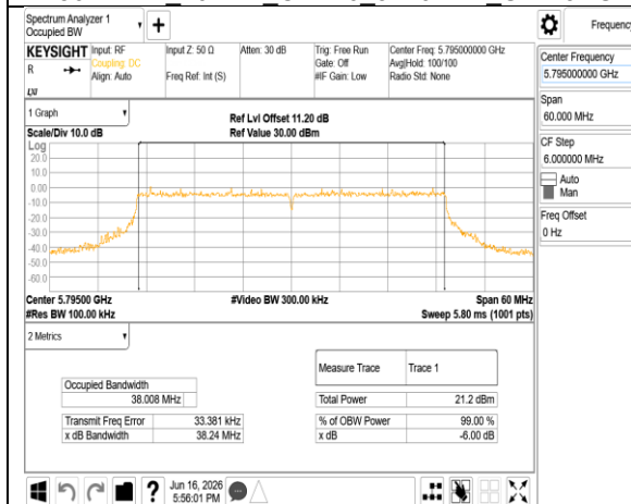
802.11be 40MHz Chain0 5795MHz RU484
