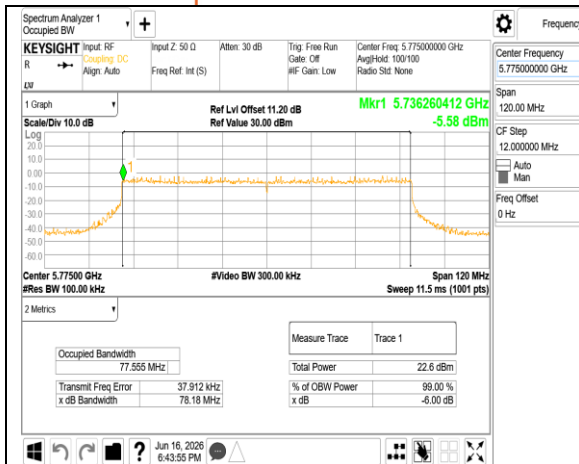
802.11be 80MHz Chain0 5775MHz RU996
