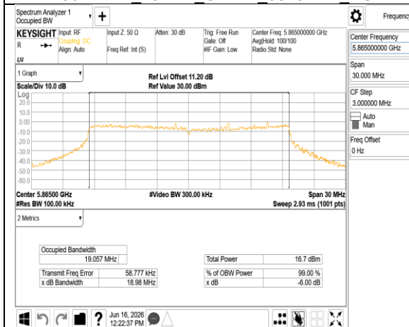
802.11be 20MHz Chain1 5865MHz RU242
