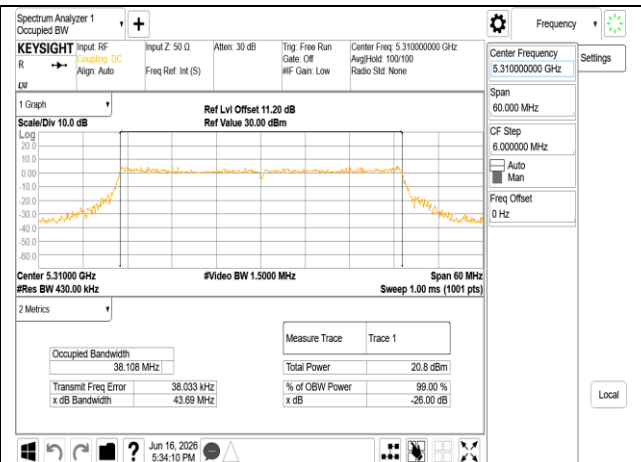
802.11be 40MHz Chain0 5310MHz RU484
