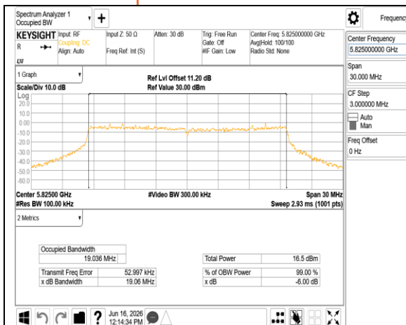
802.11be 20MHz Chain1 5825MHz RU242
