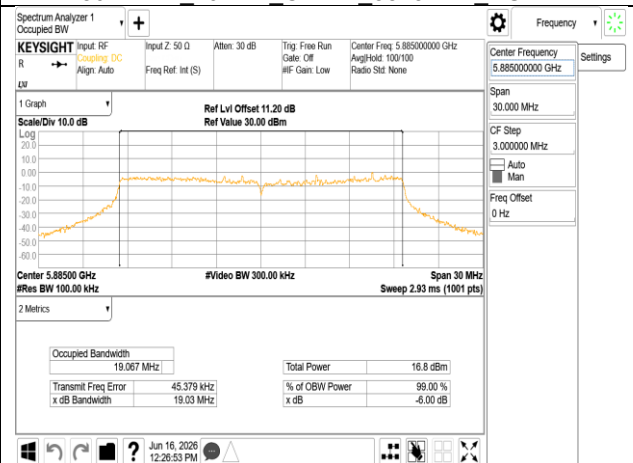
802.11be 20MHz Chain1 5885MHz RU242
