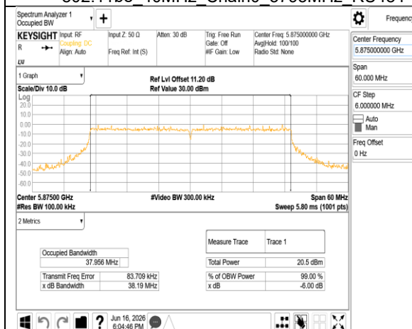
802.11be 40MHz Chain0 5875MHz RU484
