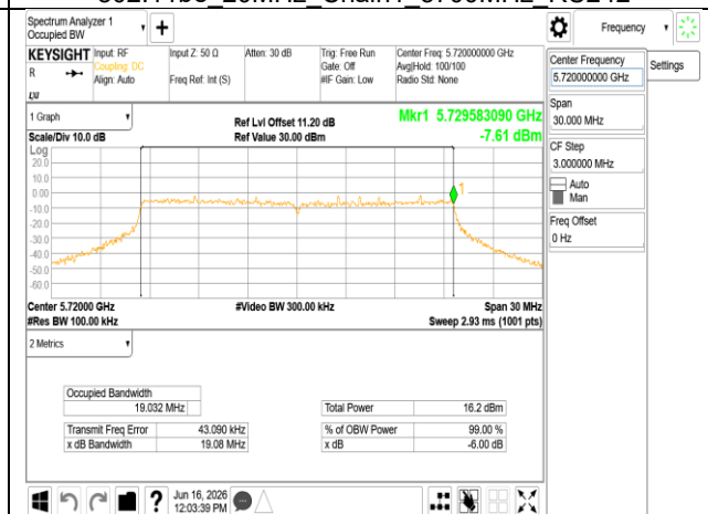
802.11be 20MHz Chain1 5720MHz UNII-3RU242
