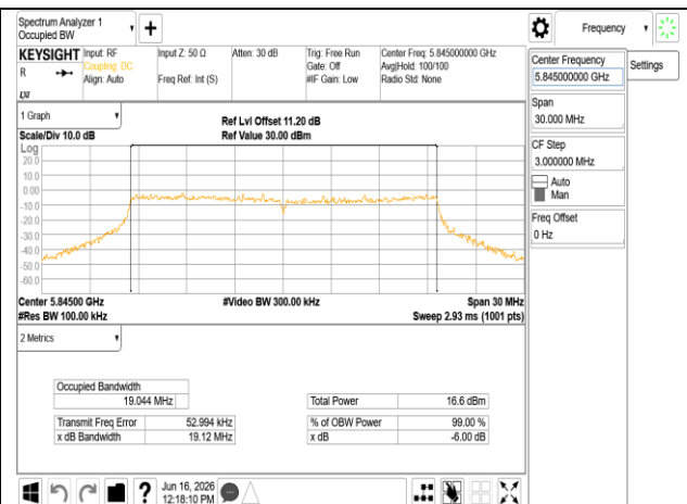
802.11be 20MHz Chain1 5845MHz RU242
