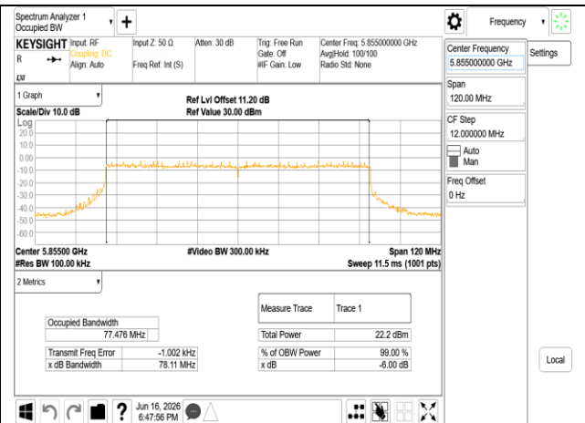
802.11be 80MHz Chain0 5855MHz RU996
