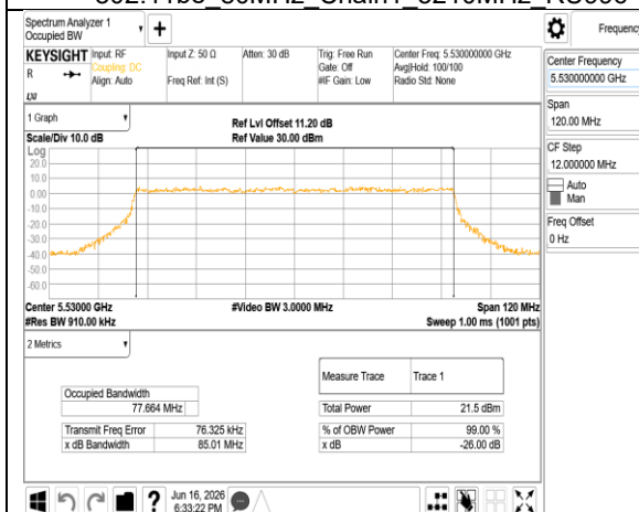
802.11be 80MHz Chain1 5530MHz RU996
