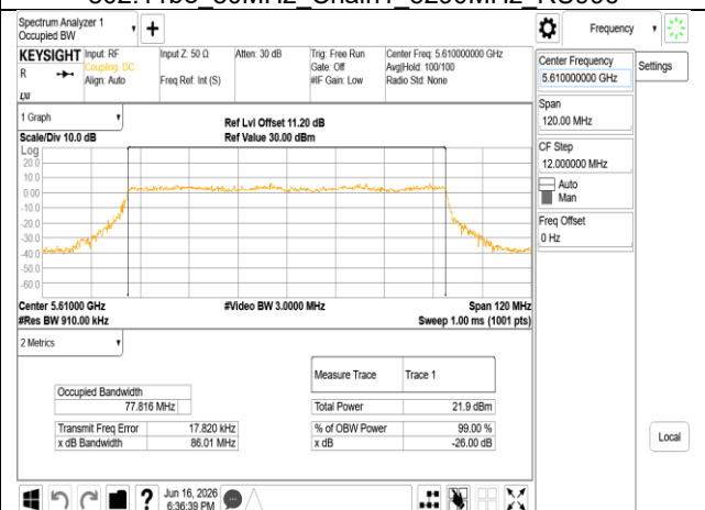
802.11be 80MHz Chain1 5610MHz RU996
