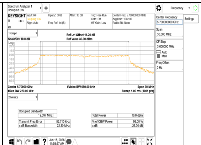
802.11be 20MHz Chain1 5700MHz RU242
