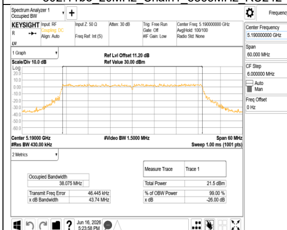
802.11be 40MHz Chain0 5190MHz RU484
