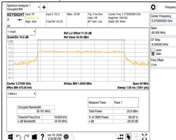
802.11be 40MHz Chain0 5270MHz RU484
