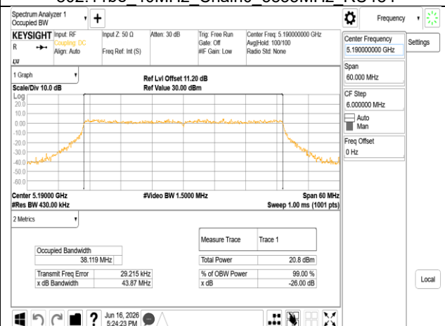
802.11be 40MHz Chain1 5190MHz RU484
