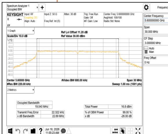
802.11be 20MHz Chain1 5600MHz RU242
