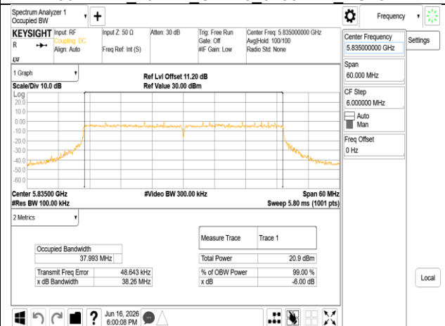
802.11be 40MHz Chain0 5835MHz RU484
