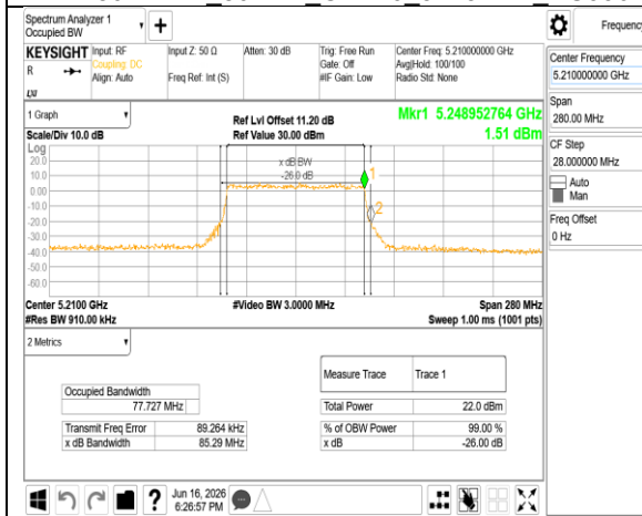
802.11be 80MHz Chain1 5210MHz RU996
