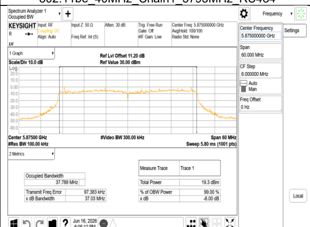
802.11be 40MHz Chain1 5875MHz RU484
