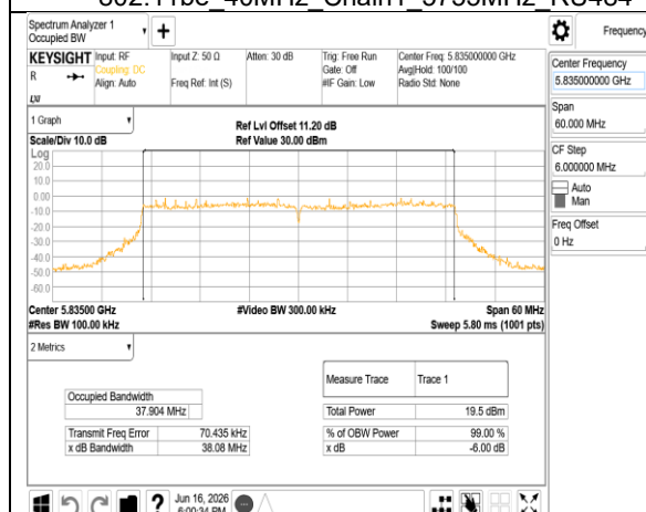
802.11be 40MHz Chain1 5835MHz RU484
