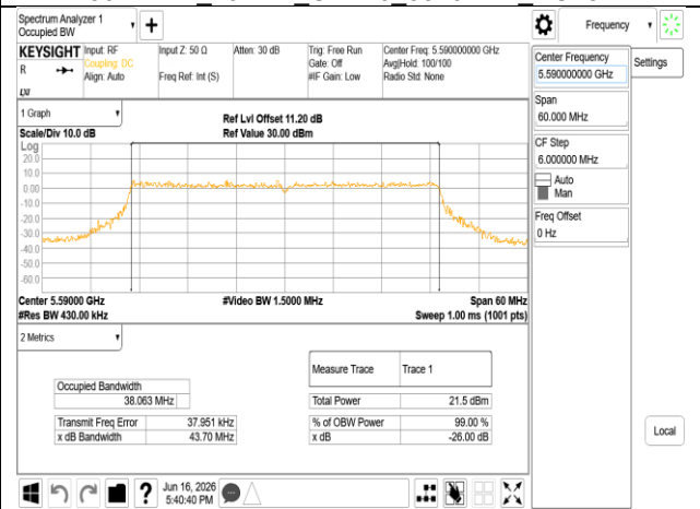
802.11be 40MHz Chain0 5590MHz RU484
