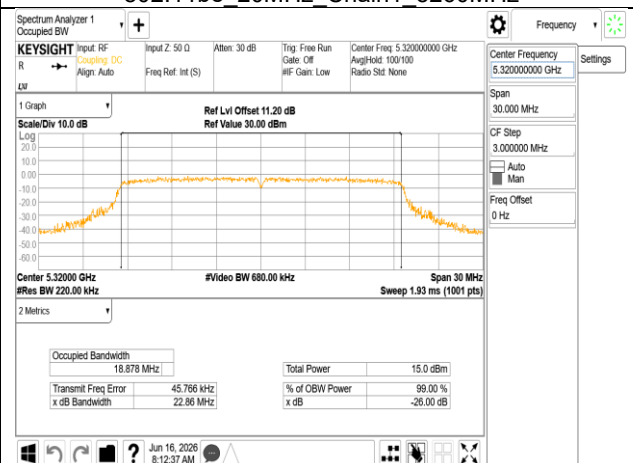
802.11be_20MHz_Chain1_5320MHz
