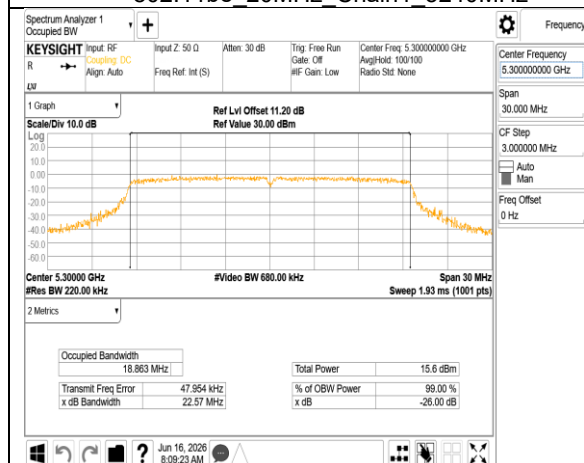
802.11be_20MHz_Chain1_5300MHz
