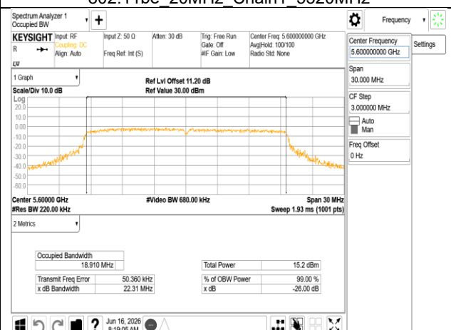
802.11be_20MHz_Chain1_5600MHz
