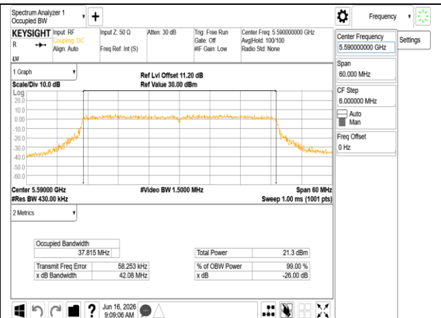
802.11be 40MHz Chain0 5590MHz
