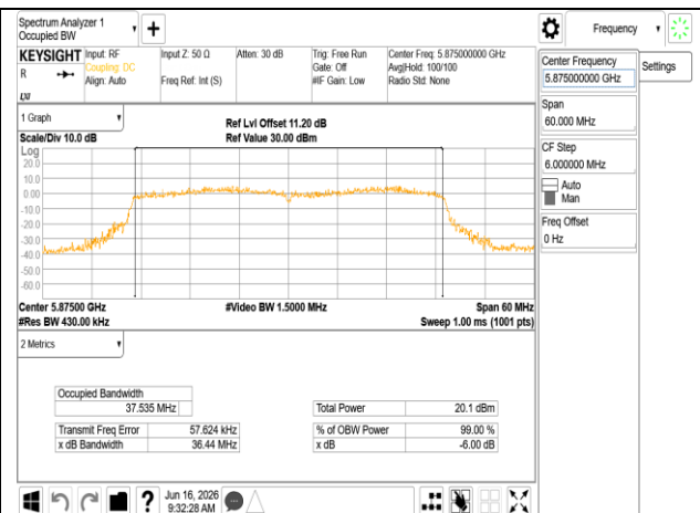
802.11be_40MHz_Chain1_5875MHz
