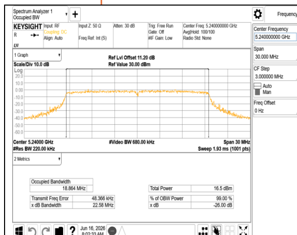
802.11be_20MHz_Chain1_5240MHz
