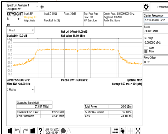
802.11be 40MHz Chain0 5510MHz
