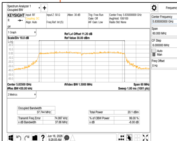
802.11be_40MHz_Chain1_5835MHz
