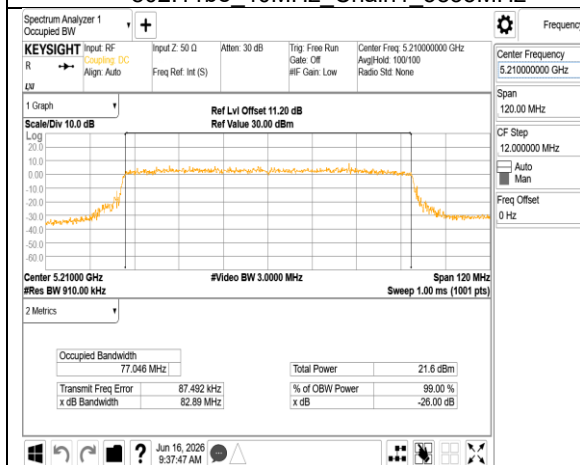
802.11be_80MHz_Chain0_5210MHz
