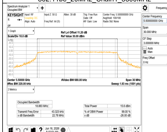
802.11be_20MHz_Chain1_5500MHz
