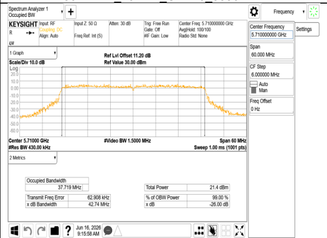
802.11be 40MHz Chain0 5710MHz
