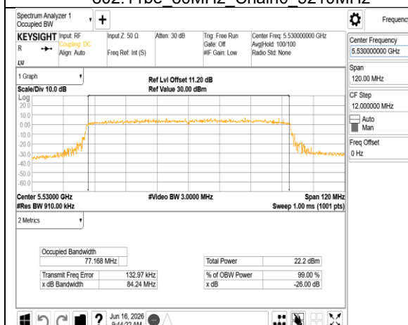
802.11be_80MHz_Chain0_5530MHz
