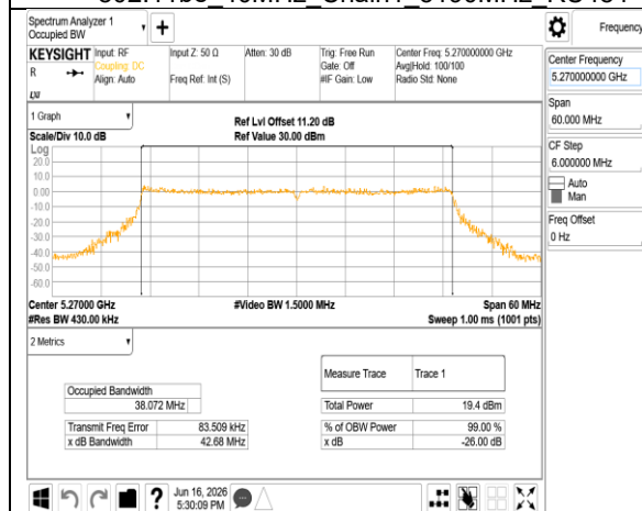
802.11be 40MHz Chain1 5270MHz RU484
