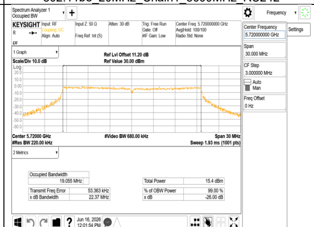
802.11be 20MHz Chain1 5720MHz RU242
