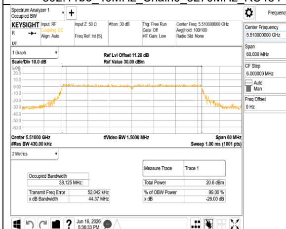
802.11be 40MHz Chain0 5510MHz RU484
