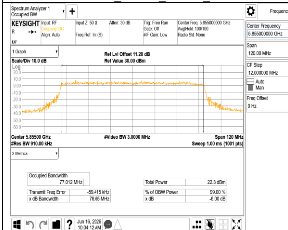
802.11be_80MHz_Chain0_5855MHz
