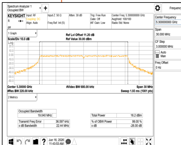
802.11be 20MHz Chain1 5300MHz RU242
