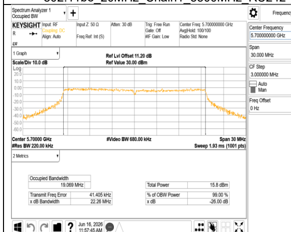
802.11be 20MHz Chain1 5700MHz RU242
