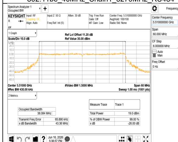
802.11be 40MHz Chain1 5510MHz RU484
