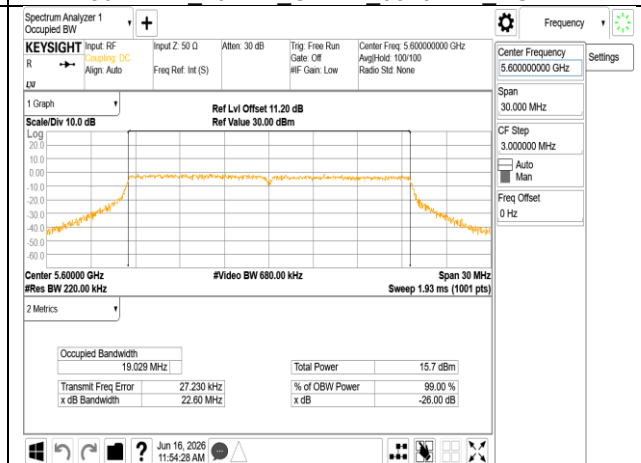
802.11be 20MHz Chain1 5600MHz RU242
