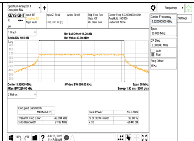
802.11be 20MHz Chain1 5320MHz RU242
