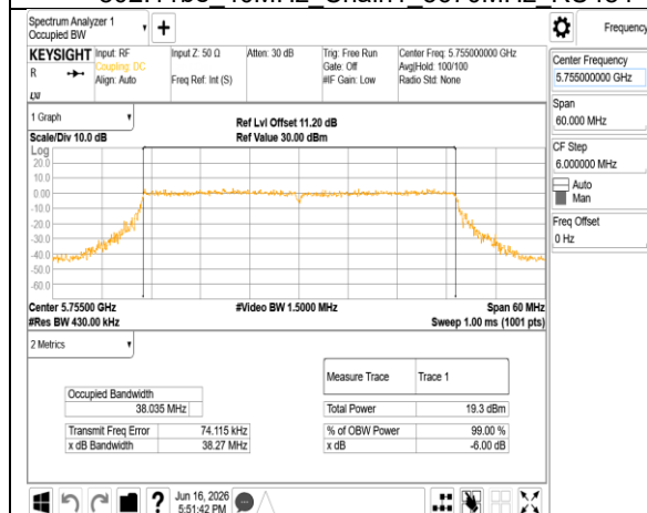
802.11be 40MHz Chain1 5755MHz RU484
