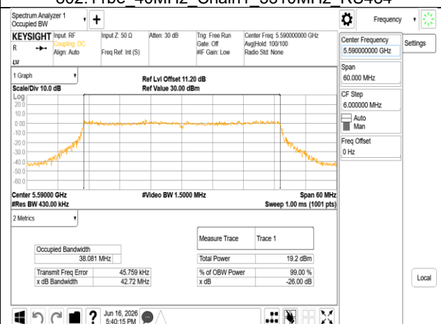
802.11be 40MHz Chain1 5590MHz RU484
