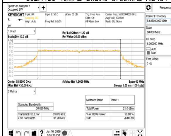
802.11be 40MHz Chain0 5835MHz RU484
