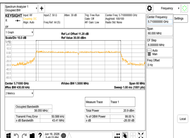
802.11be 40MHz Chain0 5710MHz RU484
