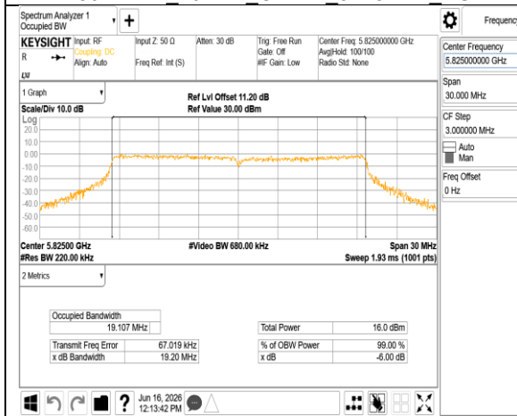
802.11be 20MHz Chain1 5825MHz RU242
