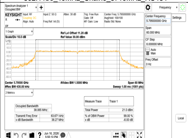
802.11be 40MHz Chain0 5795MHz RU484
