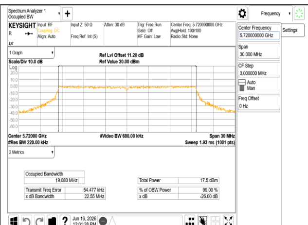
802.11be 20MHz Chain0 5720MHz RU242
