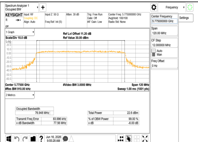
802.11be_80MHz_Chain0_5775MHz
