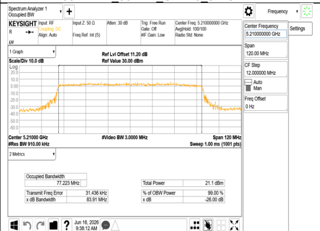
802.11be_80MHz_Chain1_5210MHz
