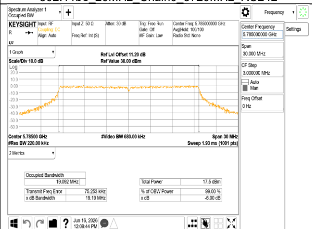
802.11be 20MHz Chain0 5785MHz RU242
