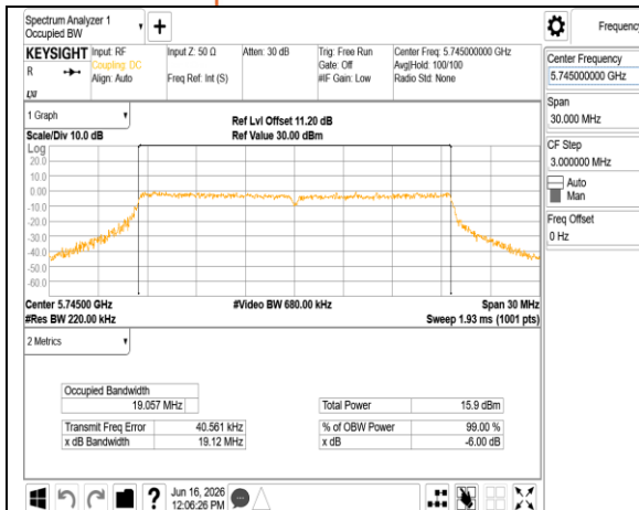
802.11be 20MHz Chain1 5745MHz RU242
