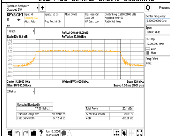
802.11be_80MHz_Chain1_5290MHz
