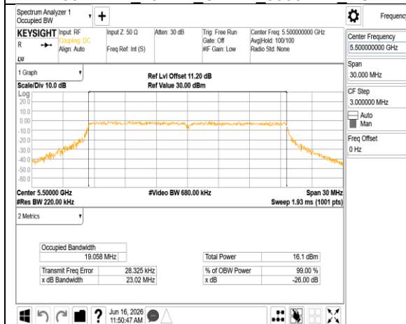
802.11be 20MHz Chain1 5500MHz RU242
