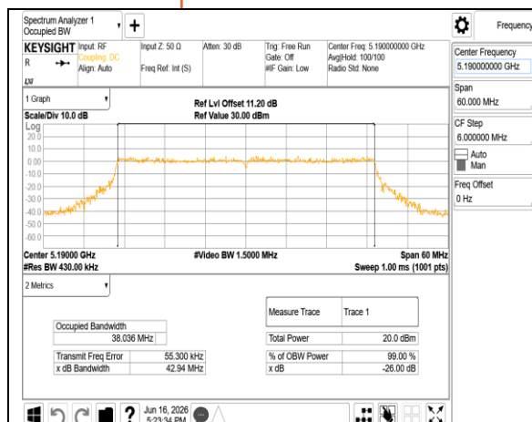
802.11be 40MHz Chain1 5190MHz RU484
