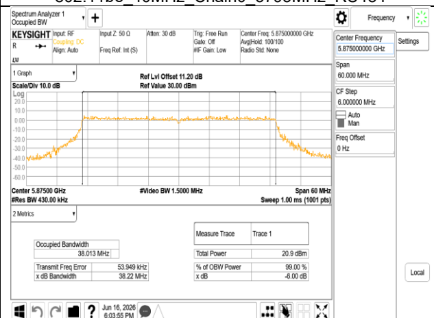
802.11be 40MHz Chain0 5875MHz RU484
