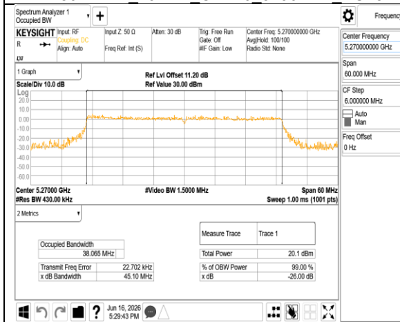
802.11be 40MHz Chain0 5270MHz RU484
