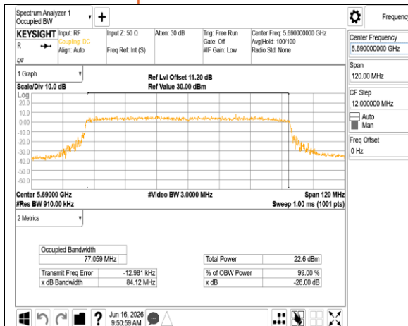
802.11be_80MHz_Chain0_5690MHz
