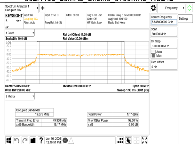
802.11be 20MHz Chain0 5845MHz RU242
