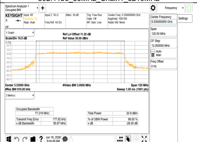
802.11be_80MHz_Chain1_5530MHz
