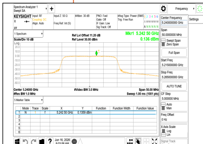
802.11be_20MHz_Chain0_5240MHz
