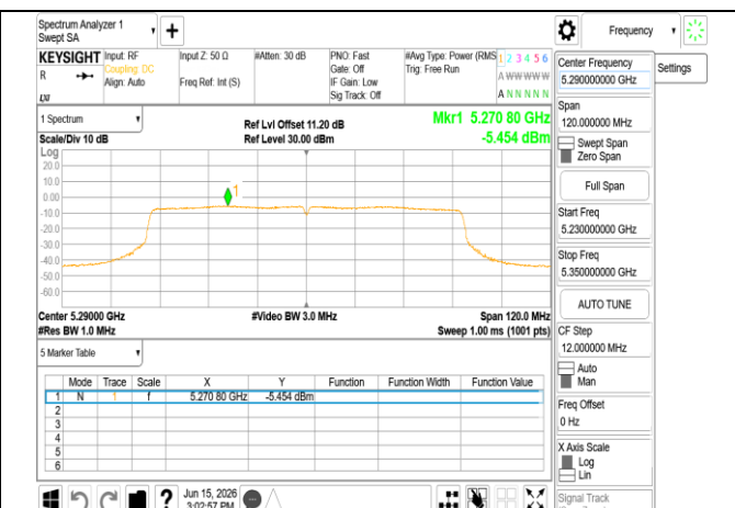
802.11ac 80MHz Chain1 5290MHz
