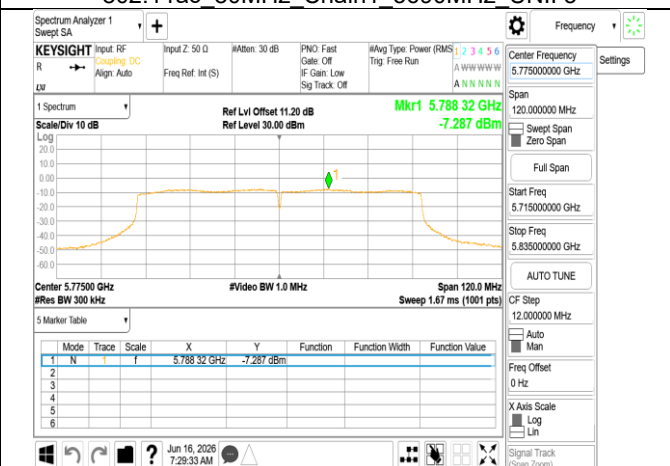
802.11ac 80MHz Chain1 5775MHz
