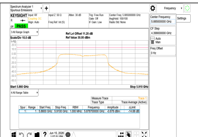
802.11n_20MHz_Chain1_5885MHz
