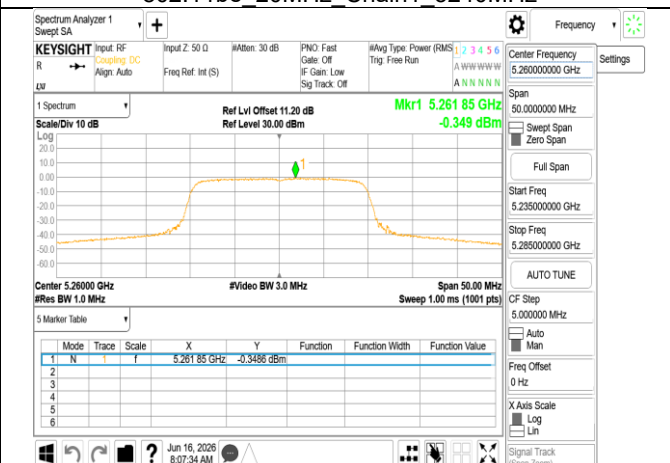
802.11be_20MHz_Chain1_5260MHz
