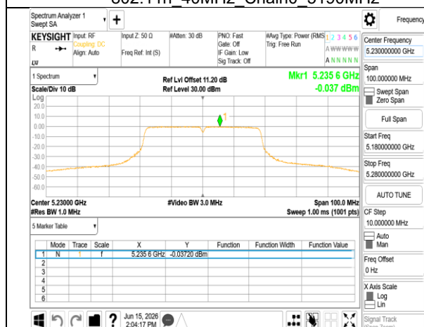
802.11n_40MHz_Chain0_5230MHz
