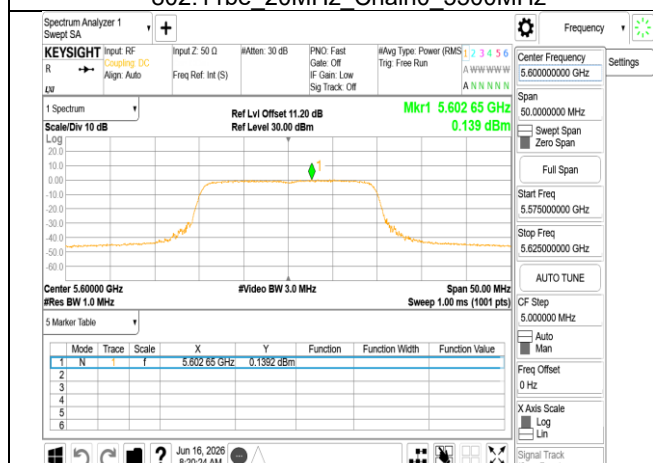
802.11be_20MHz_Chain0_5600MHz
