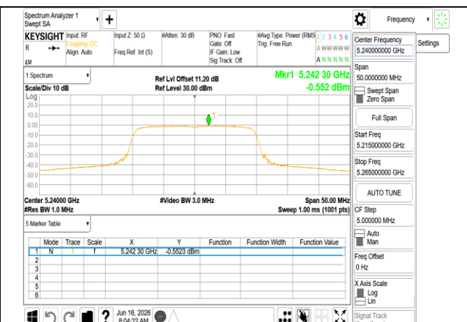
802.11be_20MHz_Chain1_5240MHz
