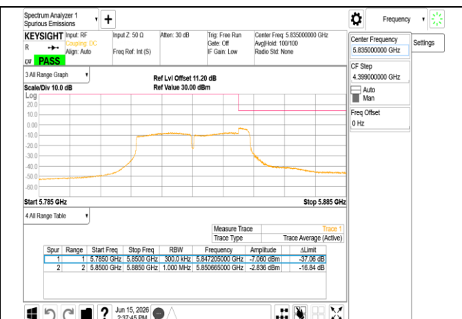
802.11n_40MHz_Chain1_5835MHz_UNII 4
