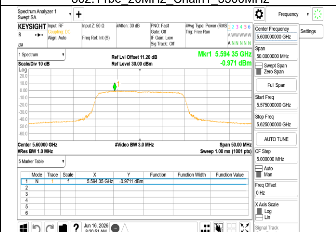
802.11be_20MHz_Chain1_5600MHz
