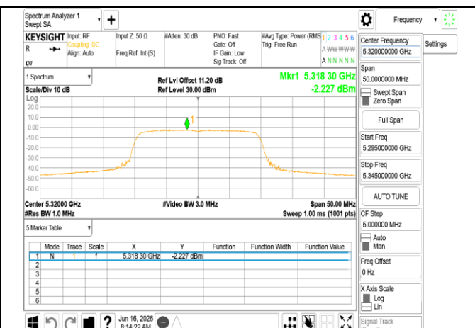
802.11be_20MHz_Chain1_5320MHz
