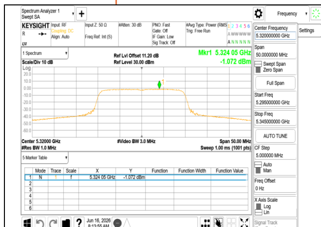
802.11be_20MHz_Chain0_5320MHz
