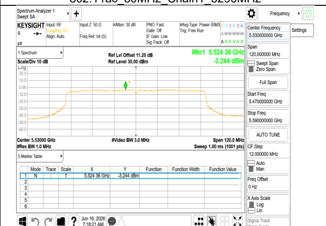
802.11ac 80MHz Chain1 5530MHz
