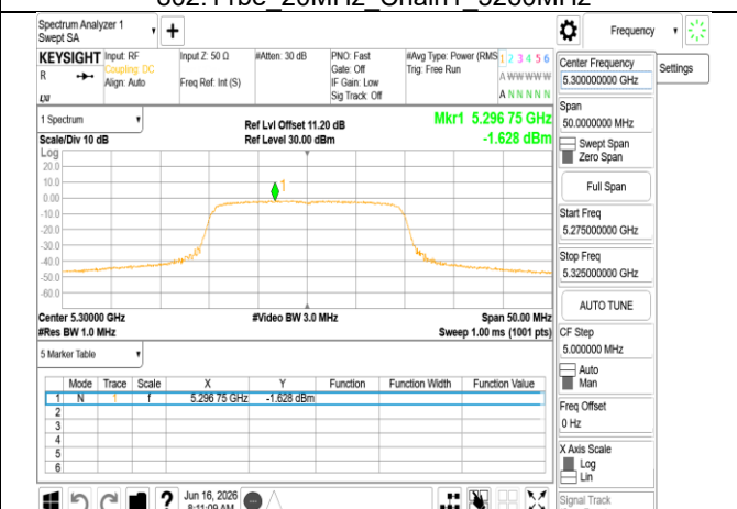
802.11be_20MHz_Chain1_5300MHz
