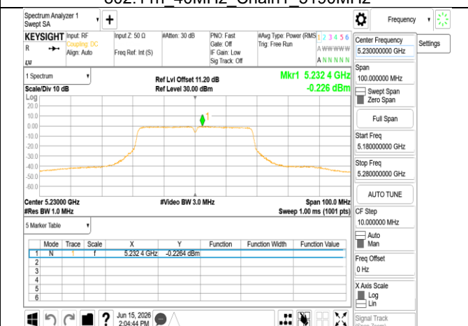
802.11n_40MHz_Chain1_5230MHz
