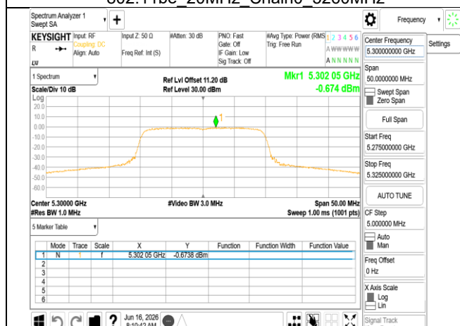
802.11be_20MHz_Chain0_5300MHz
