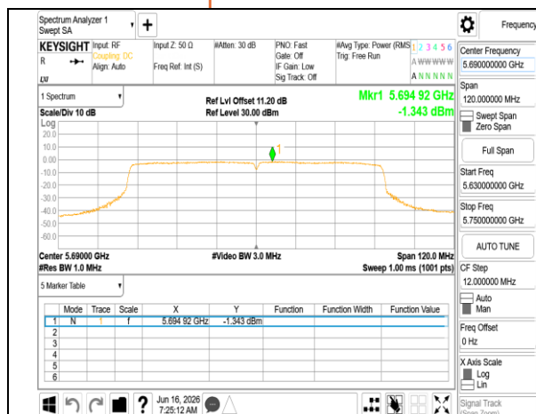
802.11ac 80MHz Chain0 5690MHz UNII 2C
