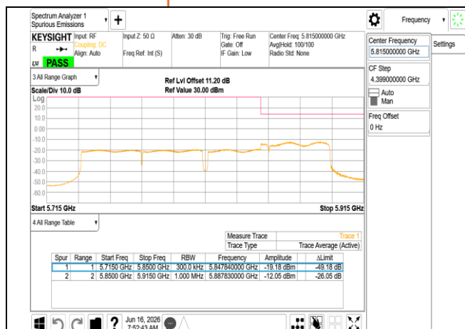
802.11ac 160MHz Chain0_5815MHz UNII 4
