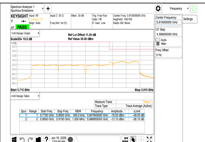
802.11ac 160MHz Chain1_5815MHz UNII 4
