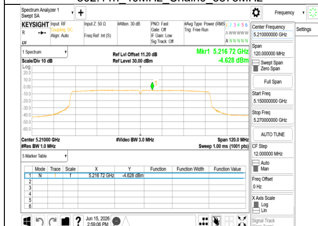
802.11ac_80MHz_Chain0_5210MHz
