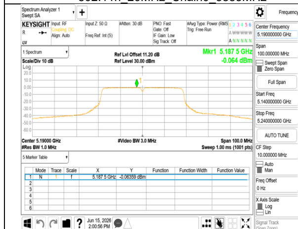
802.11n_40MHz_Chain0_5190MHz
