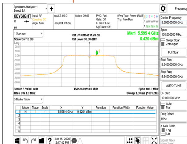
802.11n 40MHz Chain0 5590MHz
