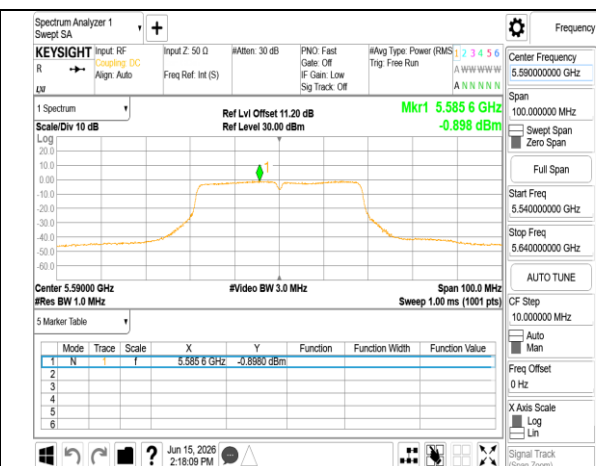
802.11n 40MHz Chain1 5590MHz
