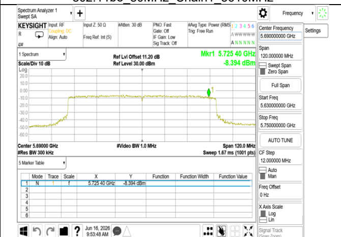
802.11be_80MHz_Chain0_5690MHz_UNII 3
