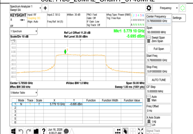
802.11be_20MHz_Chain1_5785MHz
