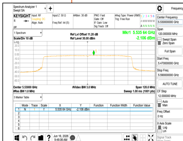
802.11be_80MHz_Chain0_5530MHz
