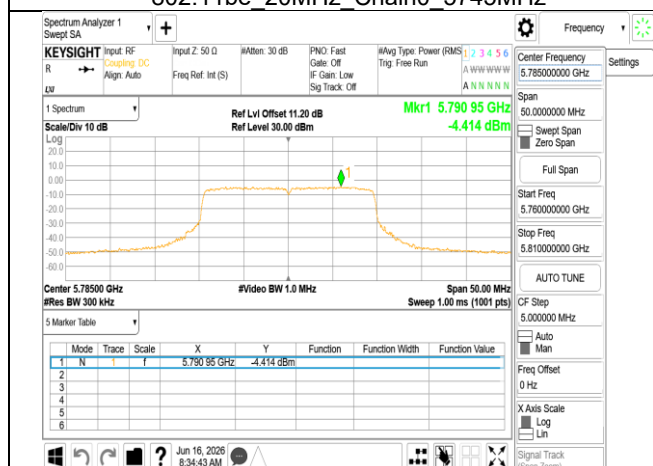
802.11be_20MHz_Chain0_5785MHz
