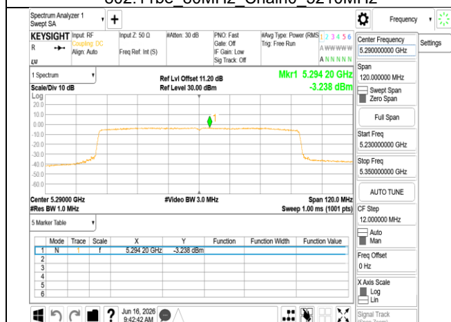
802.11be_80MHz_Chain0_5290MHz
