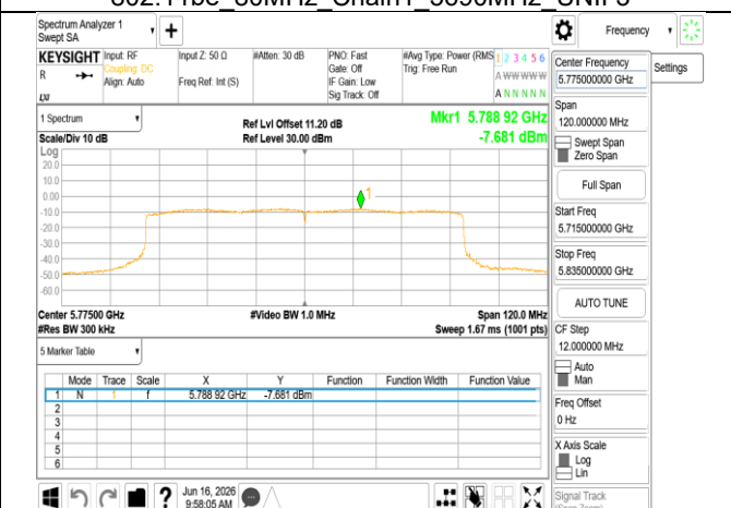
802.11be 80MHz Chain1_5775MHz
