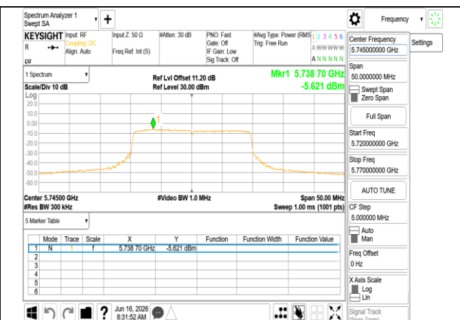
802.11be_20MHz_Chain1_5745MHz
