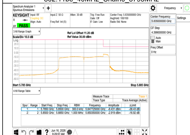
802.11be_40MHz_Chain0_5835MHz_UNII 4
