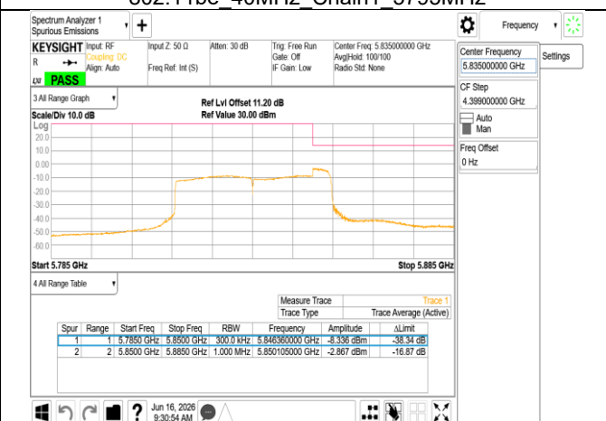
802.11be_40MHz_Chain1_5835MHz_UNII 4
