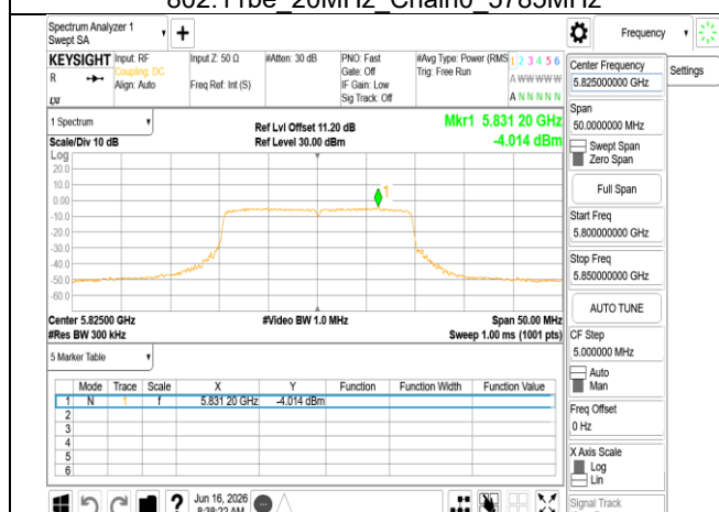
802.11be_20MHz_Chain0_5825MHz
