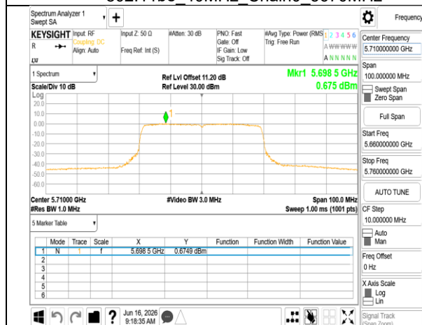
802.11be 40MHz Chain0_5710MHz UNII 2C
