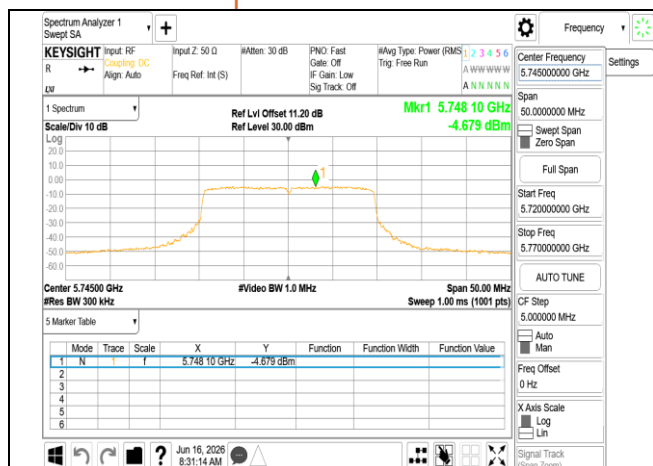
802.11be_20MHz_Chain0_5745MHz
