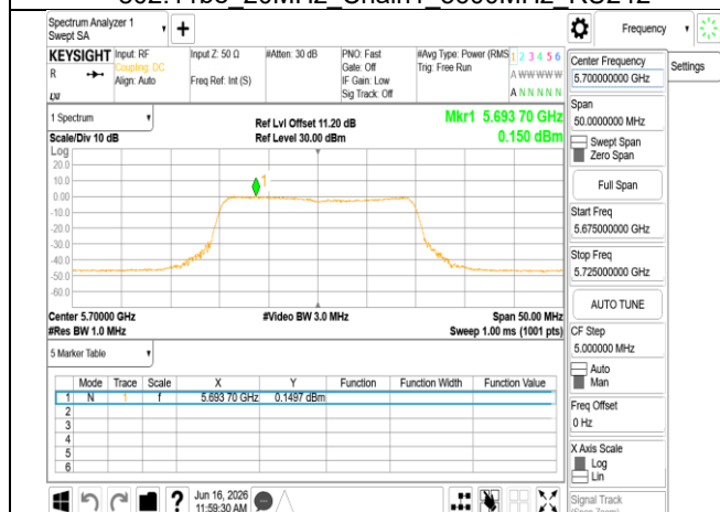
802.11be_20MHz_Chain1_5700MHz_RU242
