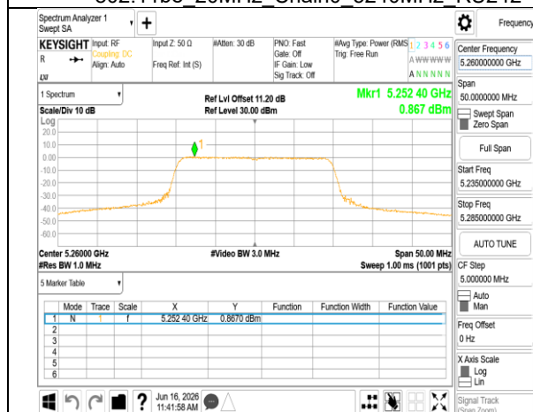
802.11be 20MHz Chain0 5260MHz RU242
