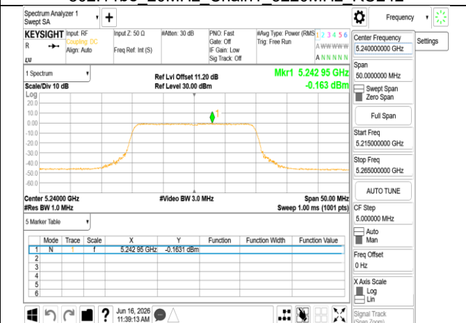
802.11be 20MHz Chain1 5240MHz RU242
