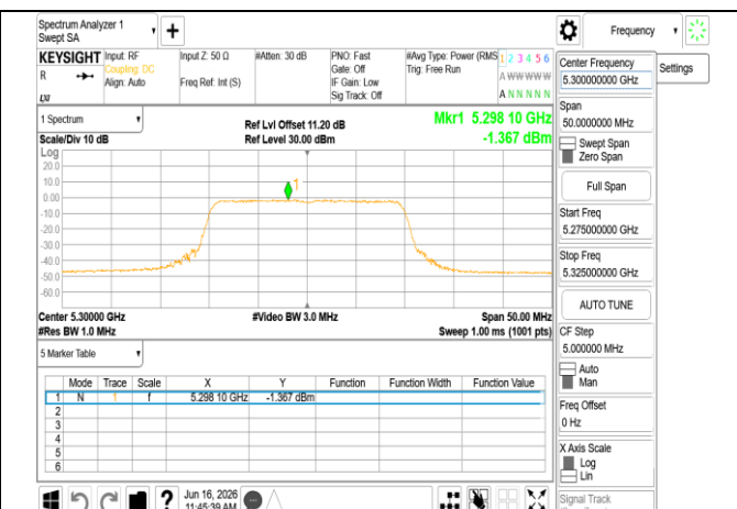
802.11be_20MHz_Chain1_5300MHz_RU242
