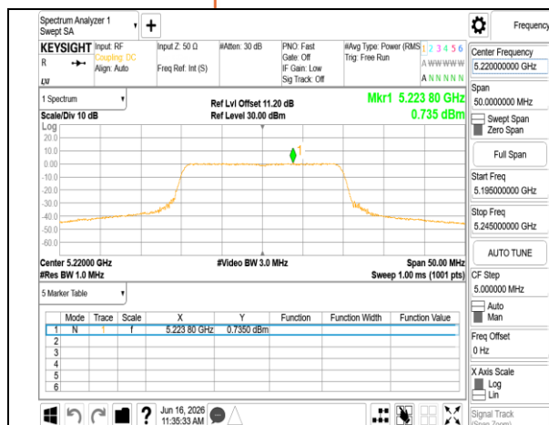
802.11be 20MHz Chain0 5220MHz RU242
