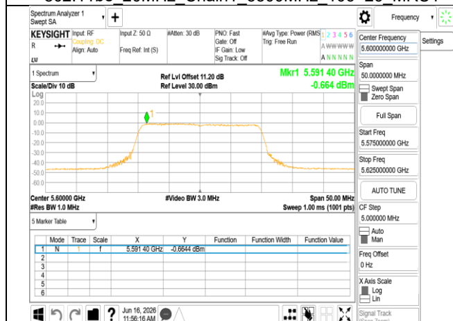
802.11be_20MHz_Chain1_5600MHz_RU242
