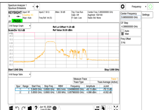
802.11be 20MHz Chain0 5865MHz RU52_37
