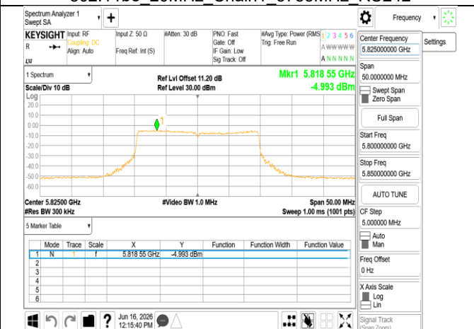
802.11be_20MHz_Chain1_5825MHz_RU242
