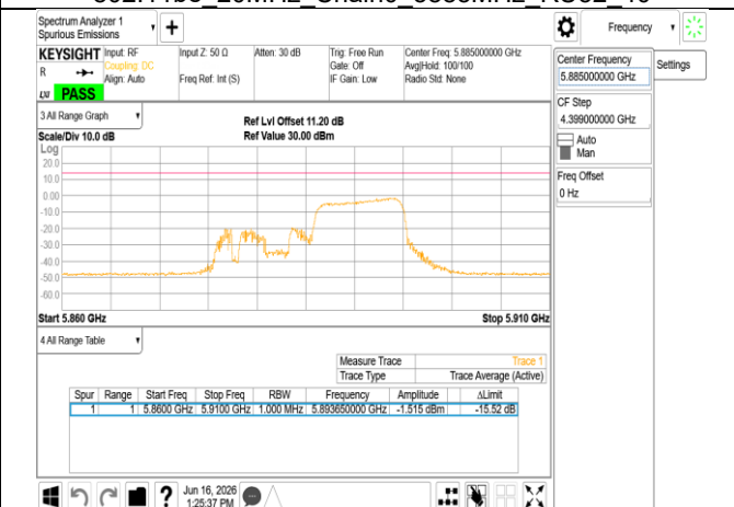
802.11be 20MHz Chain0 5885MHz RU106_54
