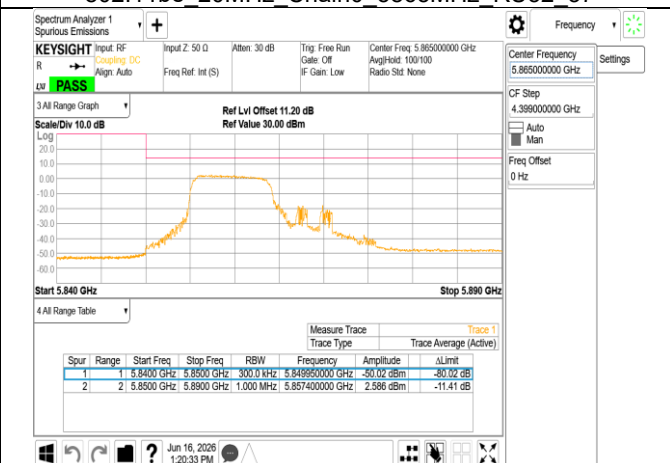
802.11be 20MHz Chain0 5865MHz RU106_53
