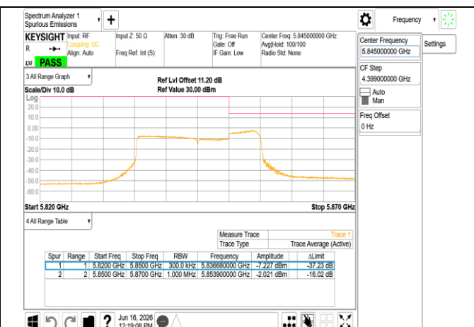
802.11be_20MHz_Chain0_5845MHz_RU242_UNII 4
