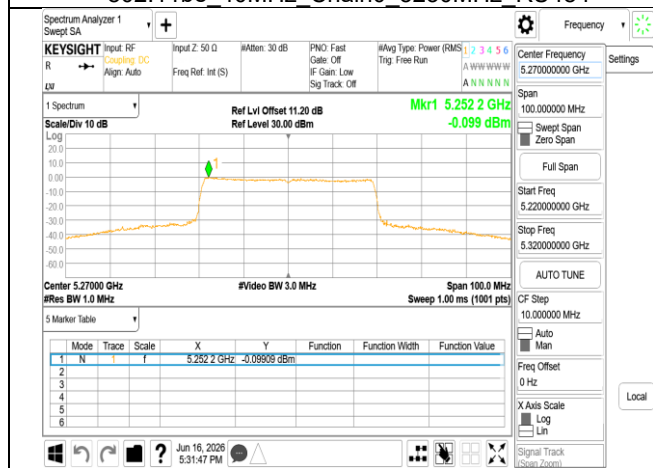
802.11be 40MHz Chain0 5270MHz RU484
