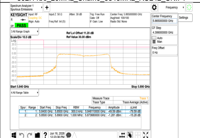
802.11be_20MHz_Chain0_5865MHz_RU242
