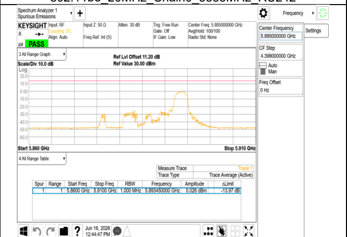
802.11be 20MHz Chain0 5885MHz RU26 8
