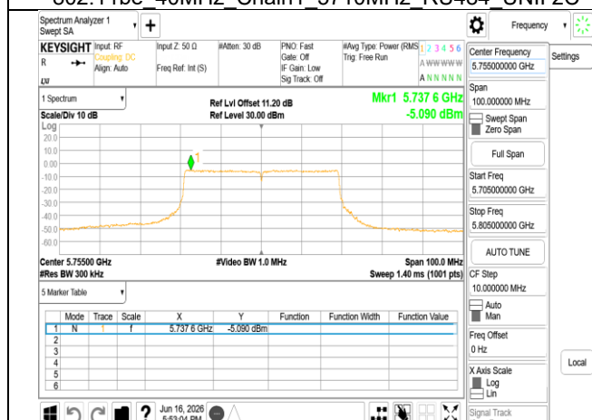
802.11be 40MHz Chain0 5755MHz RU484
