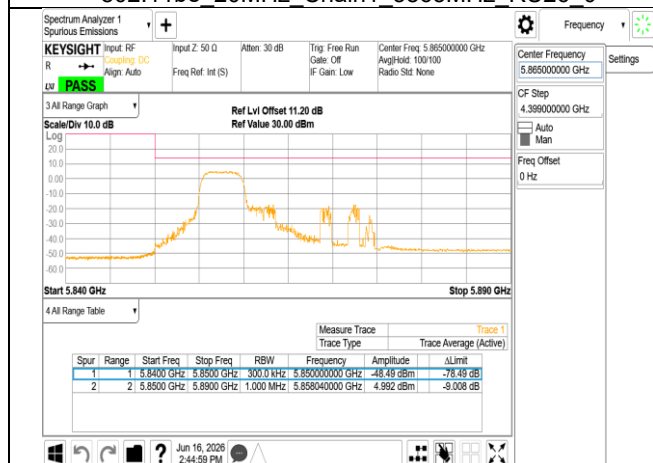
802.11be 20MHz Chain1 5865MHz RU52_37
