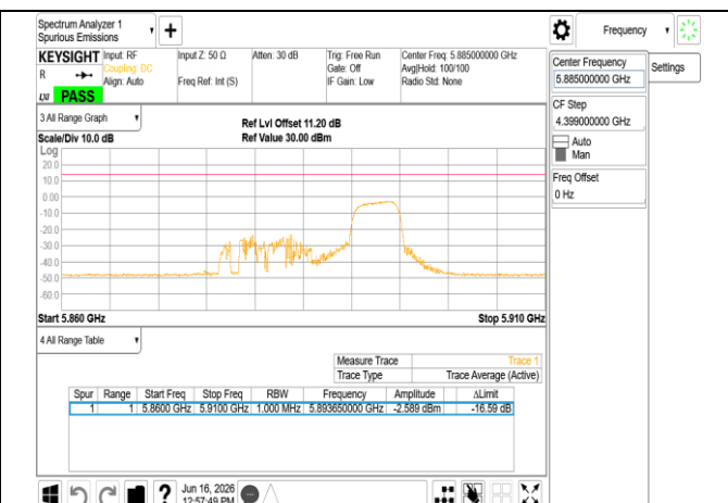
802.11be 20MHz Chain0 5885MHz RU52_40
