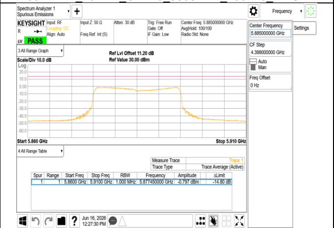
802.11be 20MHz Chain0 5885MHz RU242
