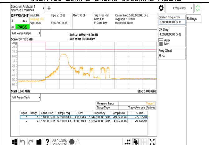
802.11be_20MHz_Chain0_5865MHz_RU26 0
