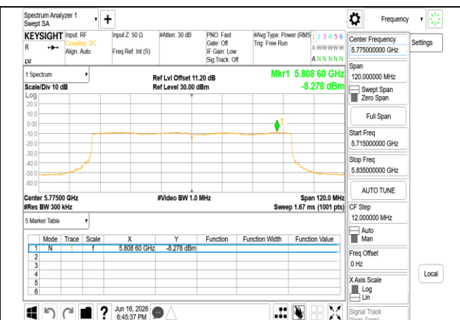
802.11be 80MHz Chain1 5775MHz RU996
