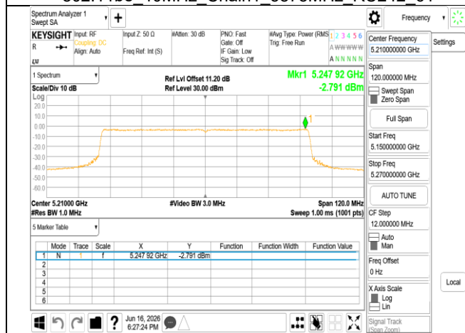
802.11be 80MHz Chain0_5210MHz RU996
