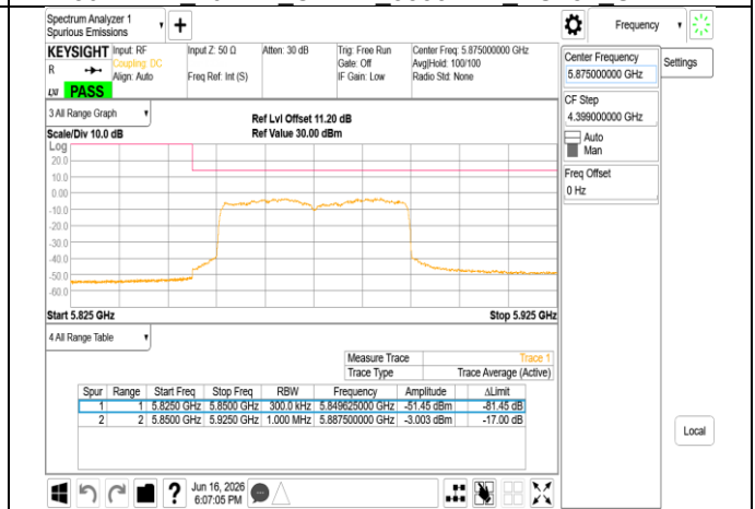
802.11be 40MHz Chain1_5875MHz_RU484
