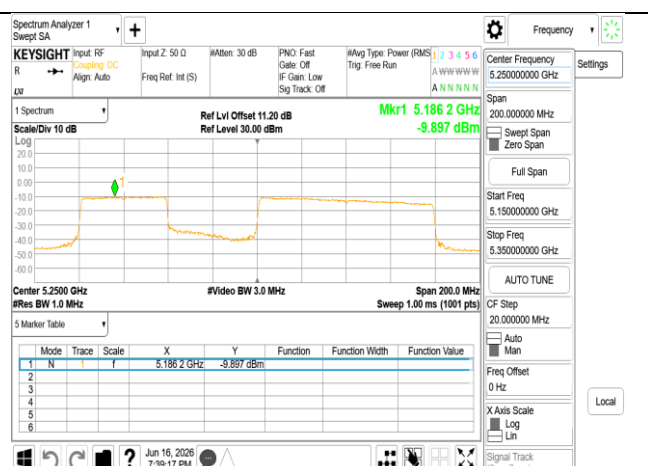
802.11be_160MHz_Chain0_5250MHz_996+484_MRU2
