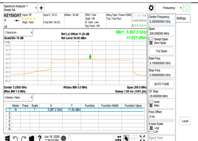
802.11be_160MHz_Chain1_5250MHz_996+484_MRU1
