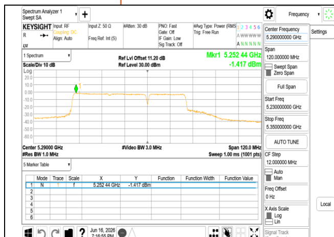
802.11be_80MHz_Chain0_5290MHz_484+242_MR44
