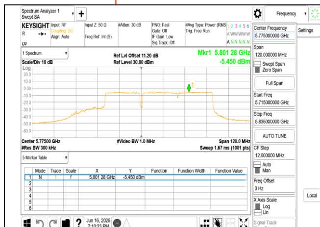
802.11be 80MHz Chain0 5775MHz 484+242 MRU1
