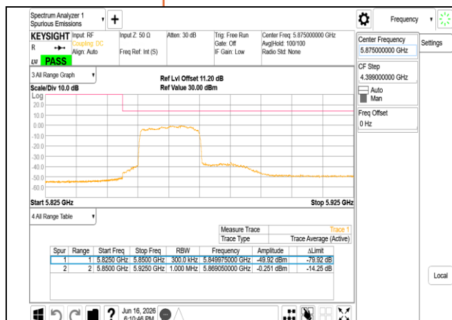
802.11be 40MHz Chain1_5875MHz RU242_61
