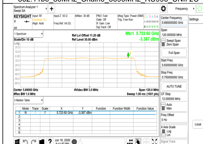
802.11be_80MHz_Chain1_5690MHz_RU996_UNII 2C
