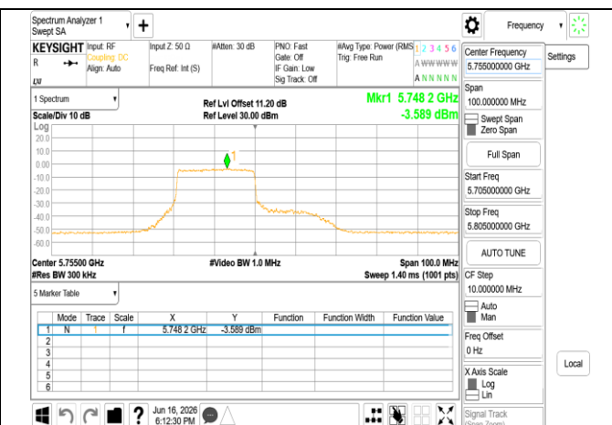
802.11be 40MHz Chain1 5755MHz RU242 61
