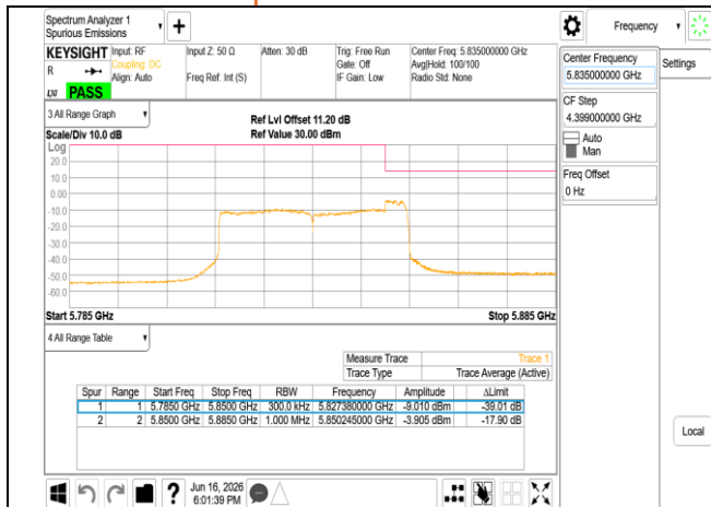
802.11be 40MHz Chain0_5835MHz_RU484_UNII 4
