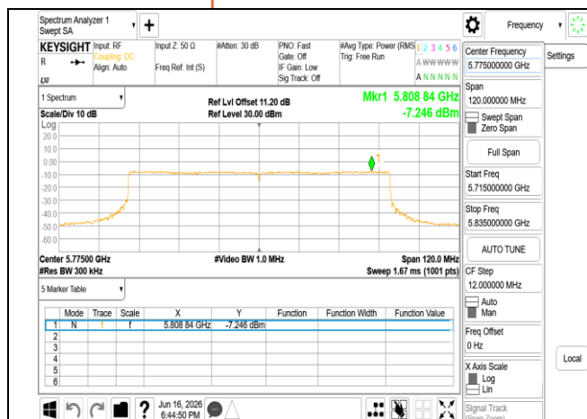
802.11be 80MHz Chain0 5775MHz RU996
