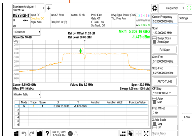
802.11be_80MHz_Chain0_5210MHz_484+242_MRUI
