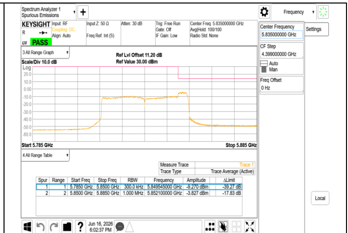
802.11be 40MHz Chain1_5835MHz_RU484_UNII 4
