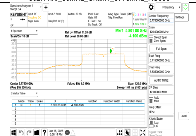
802.11be 80MHz Chain0 5775MHz RU484 66
