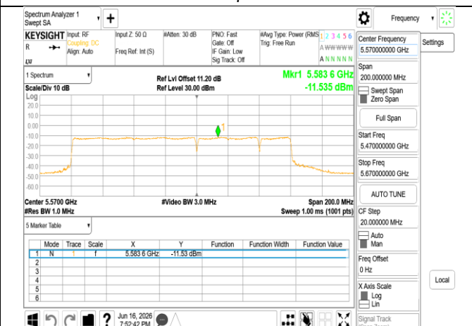
802.11be_160MHz_Chain1_5570MHz_996+484+242_MRU
