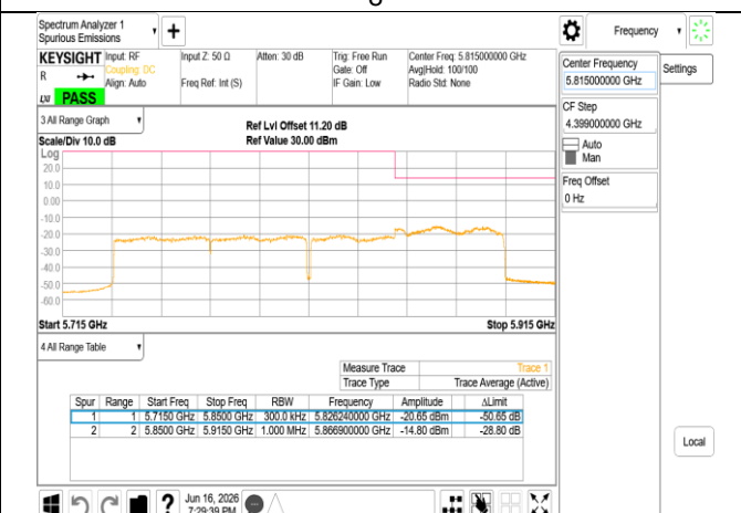
802.11be_160MHz_Chain1_5815MHz_RU996x2_UNII 4
