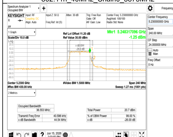
802.11n 40MHz Chain1_5230MHz
