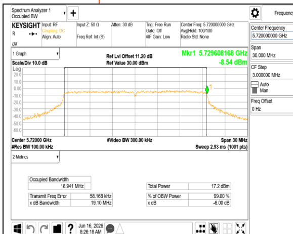
802.11be 20MHz Chain0 5720MHz UNII-3
