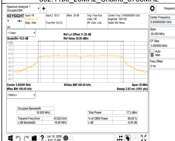
802.11be 20MHz Chain0 5845MHz
