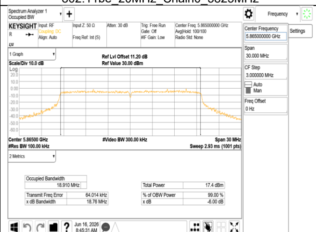
802.11be 20MHz Chain0 5865MHz
