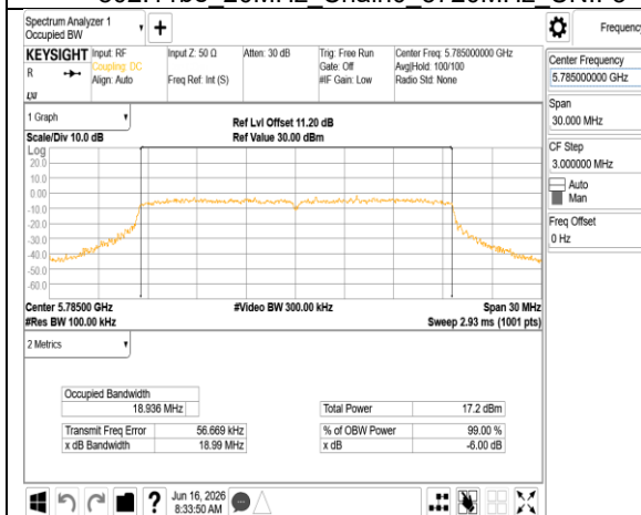
802.11be 20MHz Chain0 5785MHz
