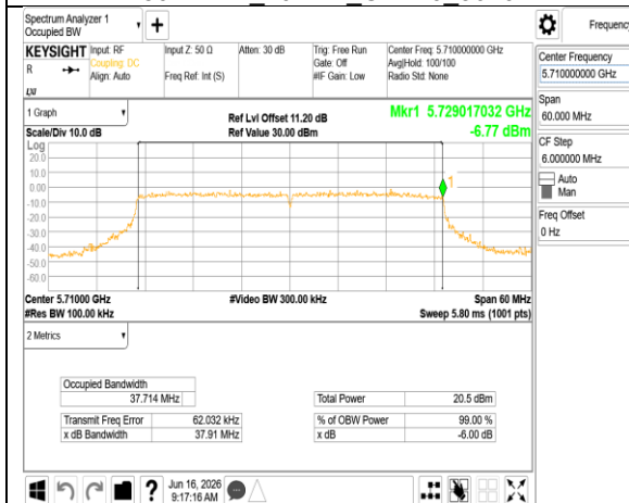
802.11be 40MHz Chain0 5710MHz UNII-3
