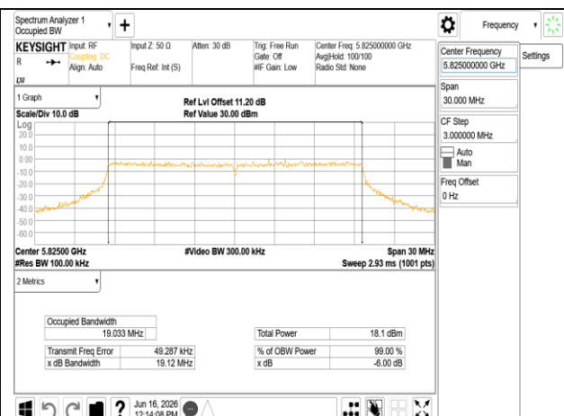
802.11be 20MHz Chain0 5825MHz RU242
