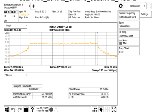
802.11be 20MHz Chain0 5865MHz RU242
