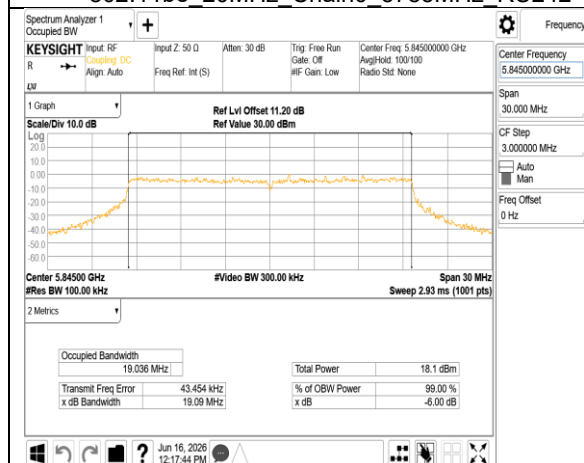
802.11be 20MHz Chain0 5845MHz RU242
