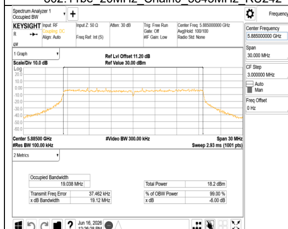
802.11be 20MHz Chain0 5885MHz RU242
