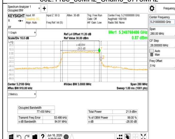
802.11be 80MHz Chain1 5210MHz
