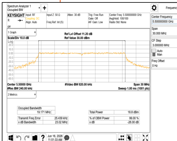
802.11be 20MHz Chain0 5500MHz RU242
