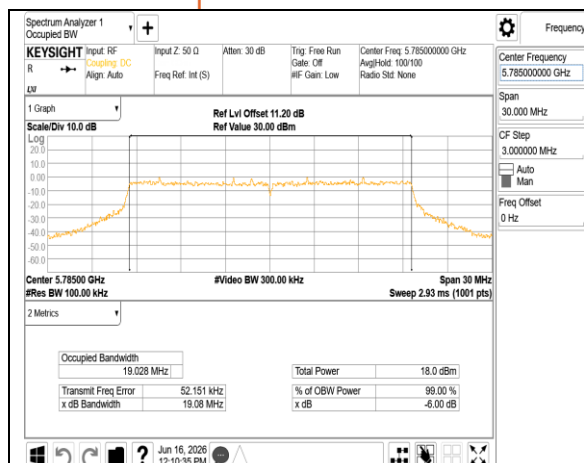
802.11be 20MHz Chain0 5785MHz RU242
