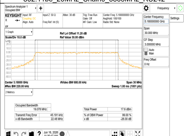
802.11be 20MHz Chain1 5180MHz RU242
