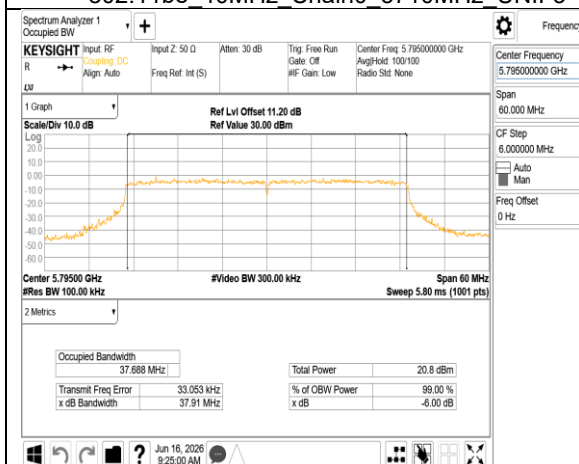
802.11be 40MHz Chain0 5795MHz
