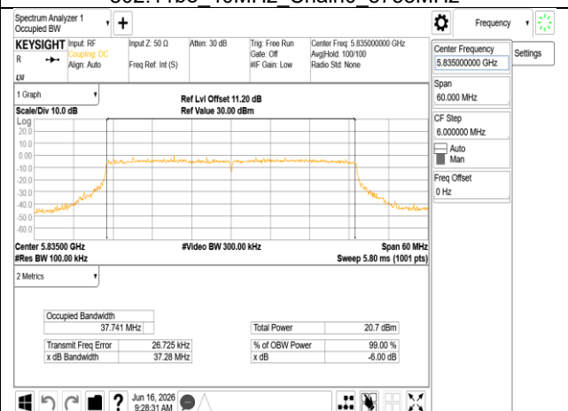
802.11be 40MHz Chain0 5835MHz
