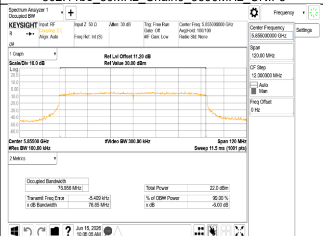
802.11be 80MHz Chain0 5855MHz
