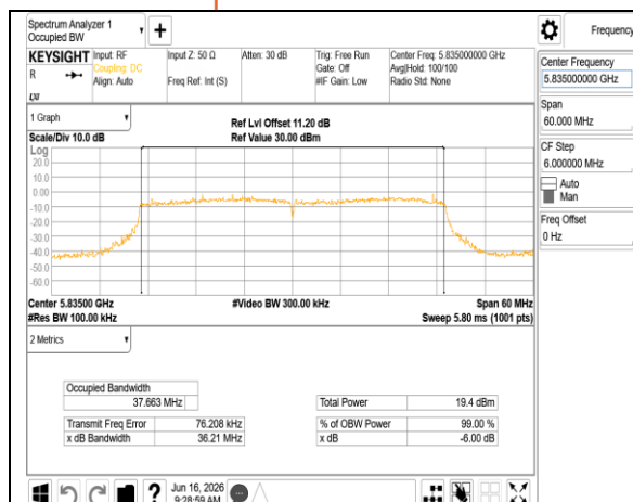
802.11be 40MHz Chain1 5835MHz
