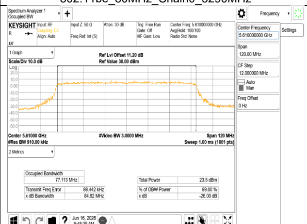
802.11be 80MHz Chain0 5610MHz
