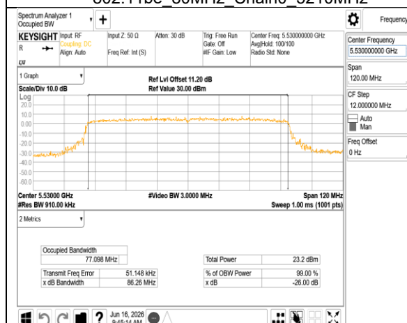
802.11be 80MHz Chain0 5530MHz
