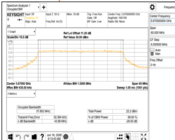
802.11be 40MHz Chain0 5670MHz
