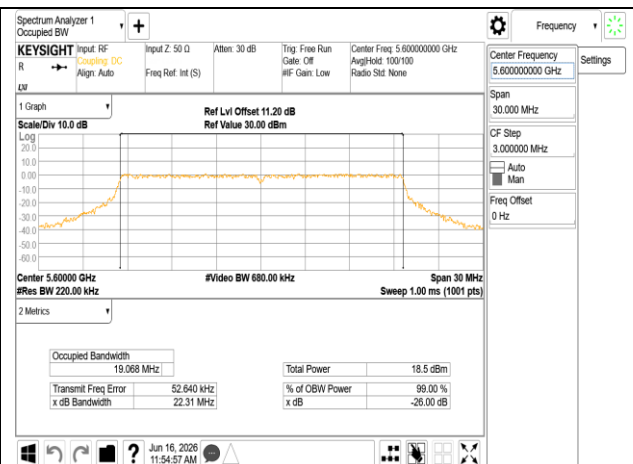
802.11be 20MHz Chain0 5600MHz RU242
