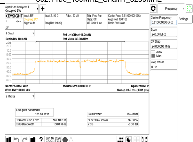
802.11be 160MHz Chain1 5815MHz
