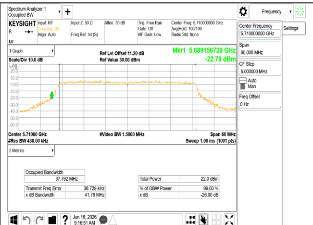
802.11be 40MHz Chain0 5710MHz UNII-2C
