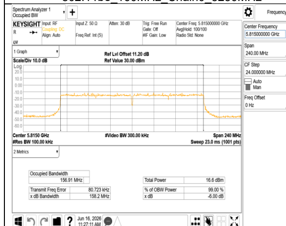
802.11be 160MHz Chain0 5815MHz
