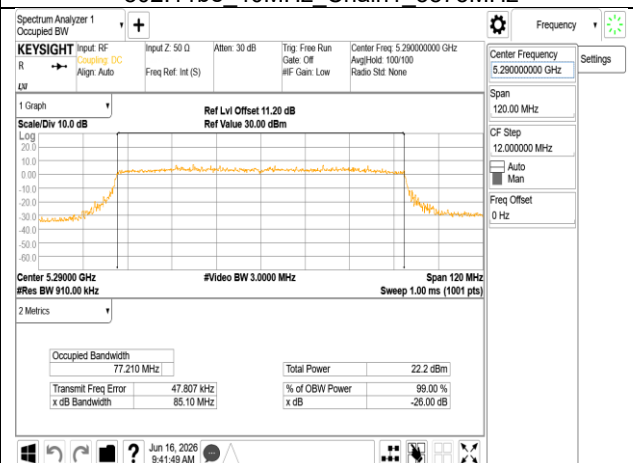
802.11be 80MHz Chain0 5290MHz
