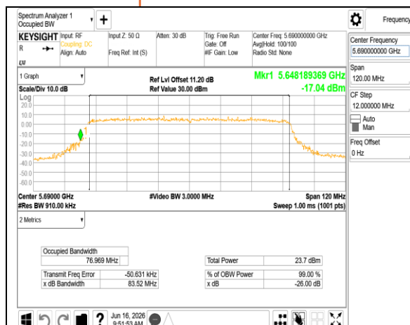
802.11be 80MHz Chain0 5690MHz UNII-2C
