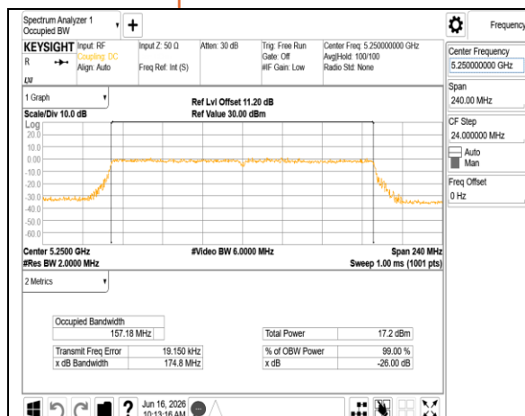
802.11be 160MHz Chain0 5250MHz
