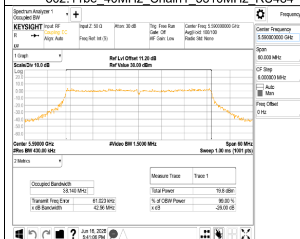
802.11be 40MHz Chain1 5590MHz RU484
