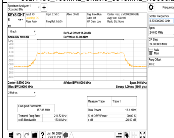
802.11be 160MHz Chain1 5570MHz RU996x2
