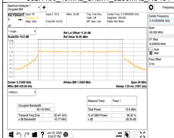
802.11be 40MHz Chain1 5310MHz RU484
