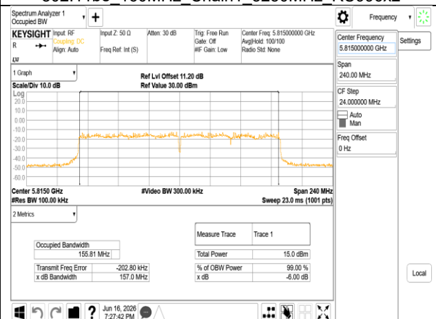
802.11be 160MHz Chain1 5815MHz RU996x2
