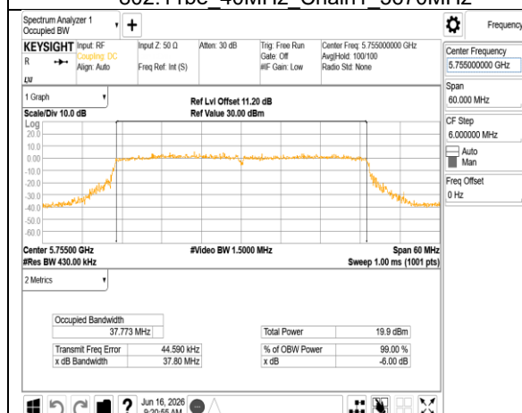
802.11be 40MHz Chain1 5755MHz
