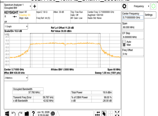
802.11be 40MHz Chain1 5710MHz
