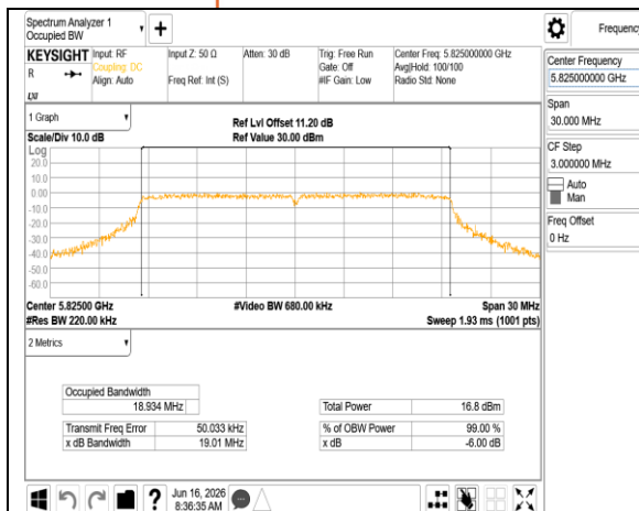
802.11be 20MHz Chain0 5825MHz
