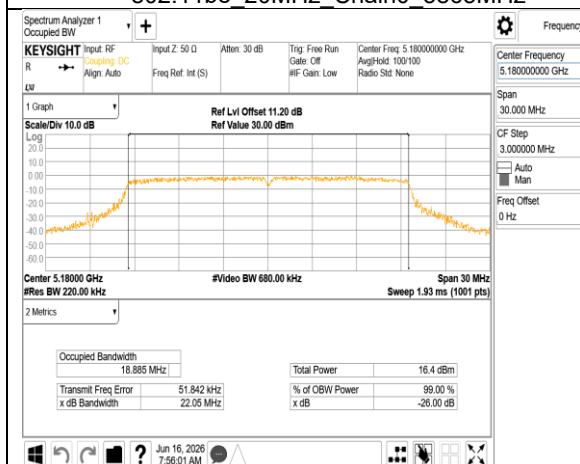
802.11be 20MHz Chain1 5180MHz
