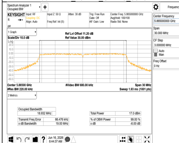
802.11be 20MHz Chain0 5865MHz
