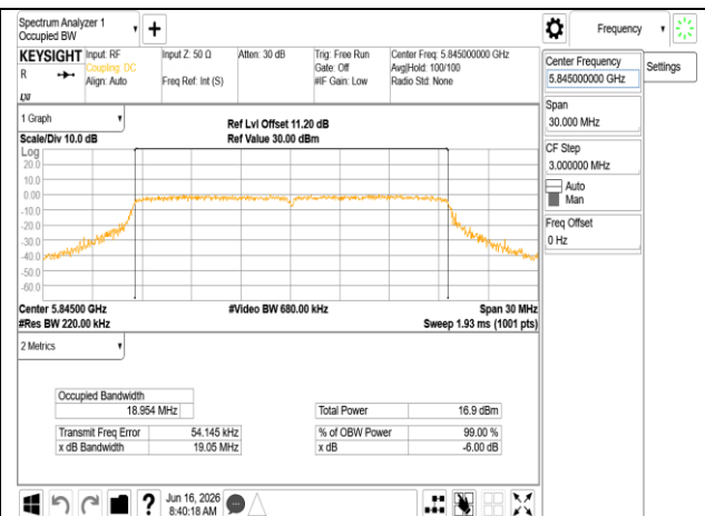
802.11be 20MHz Chain0 5845MHz
