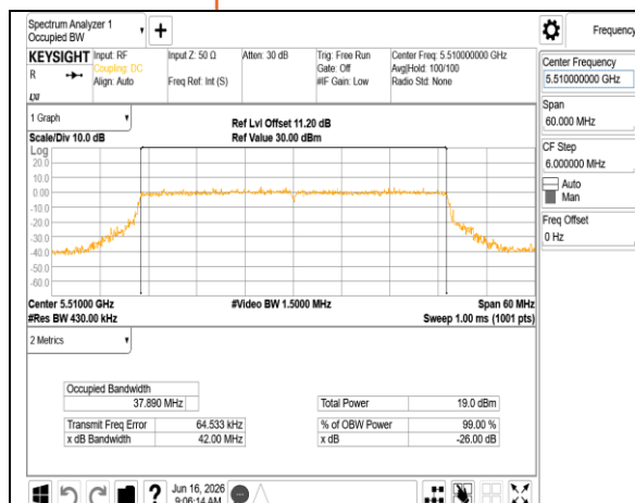
802.11be 40MHz Chain1 5510MHz
