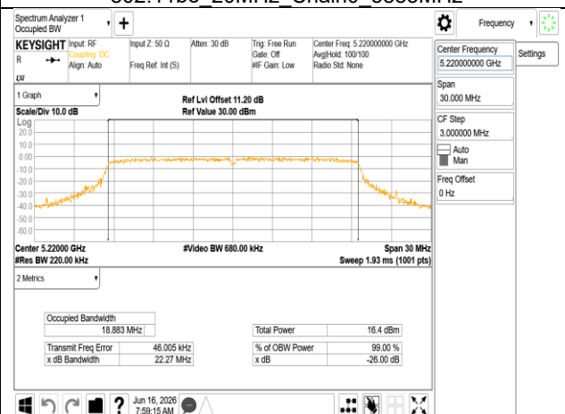
802.11be 20MHz Chain1 5220MHz
