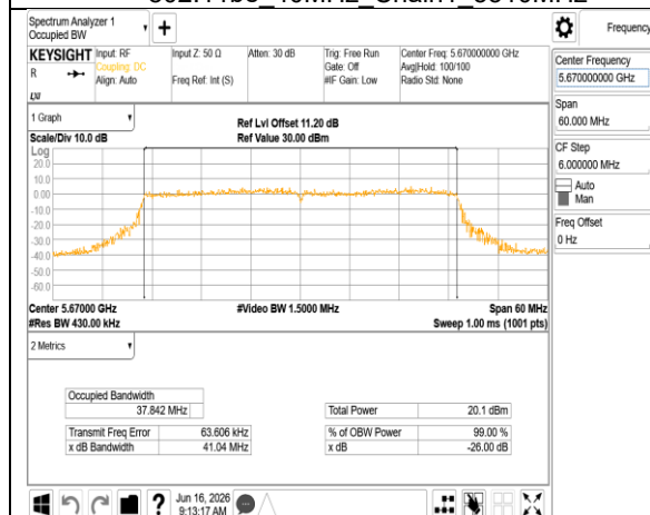
802.11be 40MHz Chain1 5670MHz
