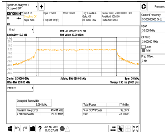
802.11be 20MHz Chain0 5300MHz RU242
