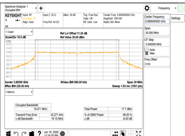
802.11be 20MHz Chain0 5885MHz RU242
