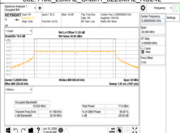
802.11be 20MHz Chain1 5260MHz RU242
