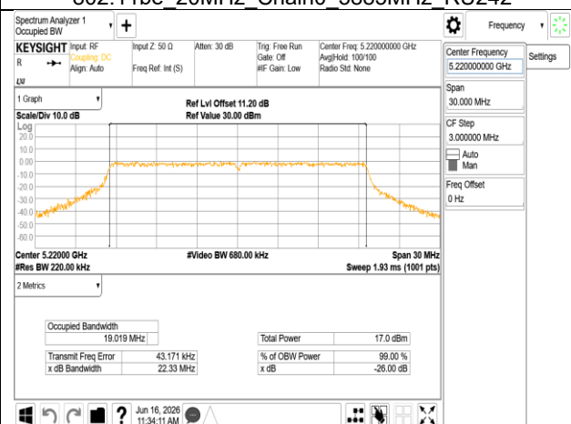
802.11be 20MHz Chain1 5220MHz RU242
