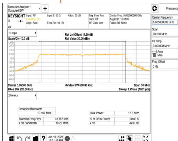
802.11be 20MHz Chain0 5865MHz RU242
