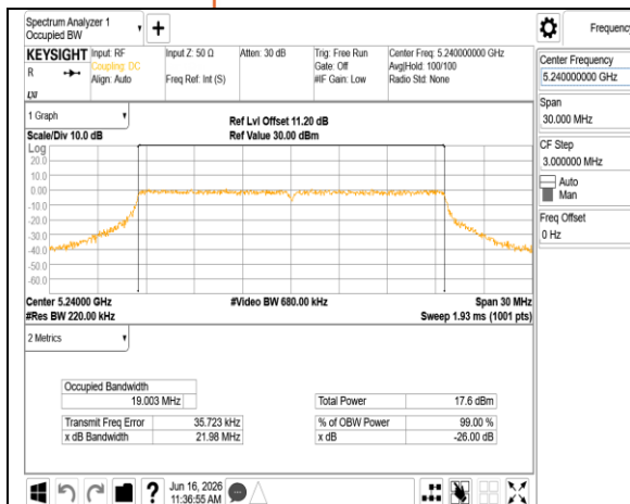
802.11be 20MHz Chain0 5240MHz RU242
