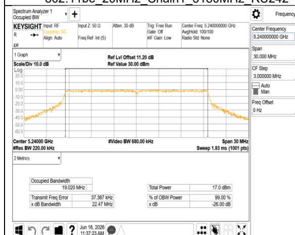
802.11be 20MHz Chain1 5240MHz RU242
