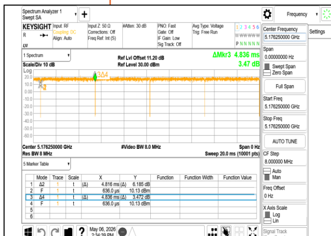
802.11be_20MHz_Chain0_5180MHz_106+26_MRU1
