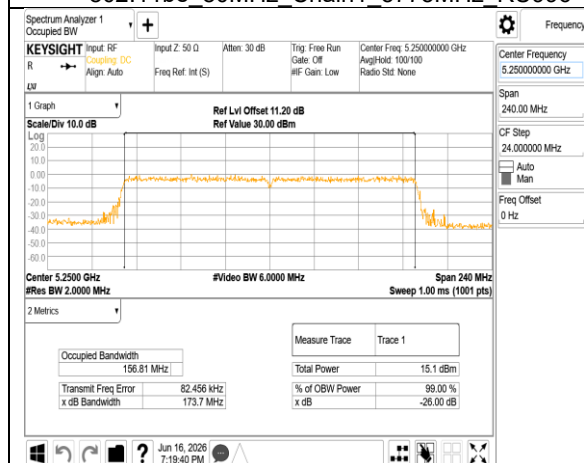
802.11be 160MHz Chain0 5250MHz RU996x2
