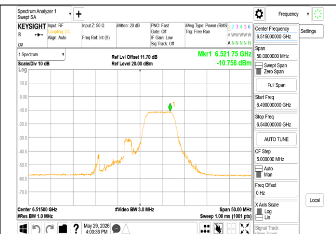
802.11be_20MHz_Chain1_6515MHz_52+26_MR1U3
