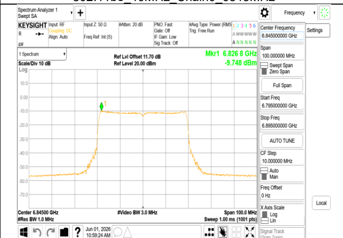
802.11be 40MHz Chain0 6845MHz RU484
