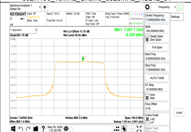
802.11be 40MHz Chain0 7005MHz
