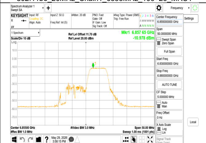
802.11be_20MHz_Chain1_6855MHz_52+26_MR1U3
