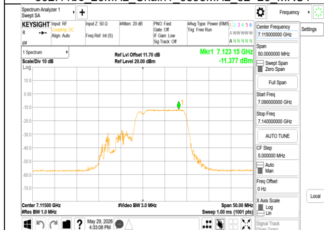
802.11be 20MHz Chain1 7115MHz 106+26 MRU2
