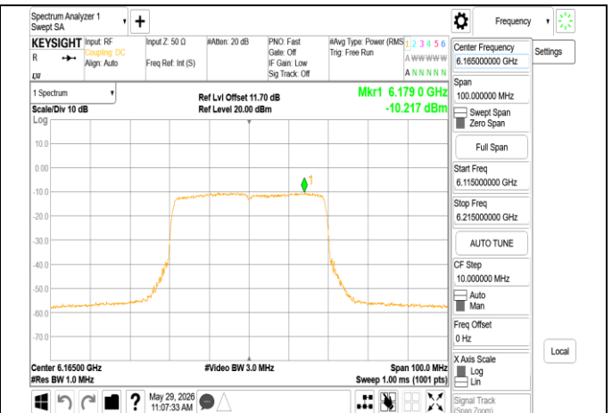
802.11be 40MHz Chain0 6165MHz
