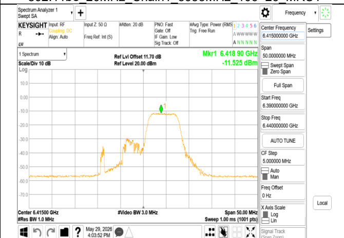
802.11be_20MHz_Chain1_6415MHz_52+26_MRUI
