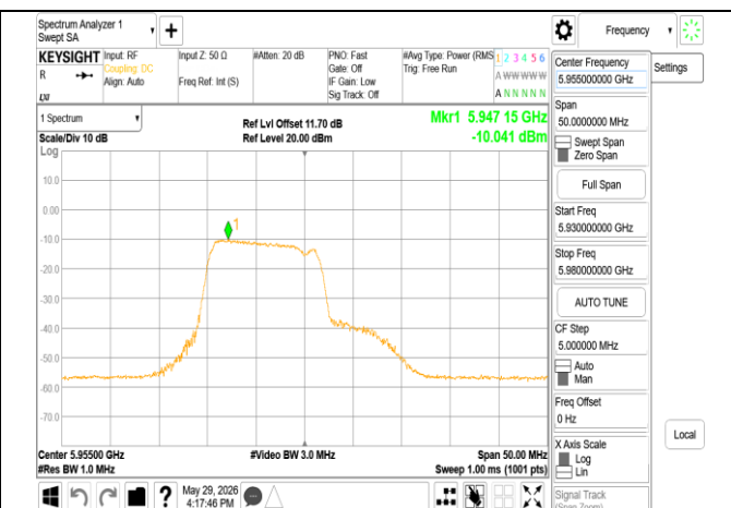
802.11be_20MHz_Chain1_5955MHz_106+26_MRUI
