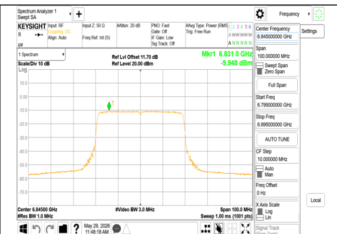
802.11be 40MHz Chain0 6845MHz
