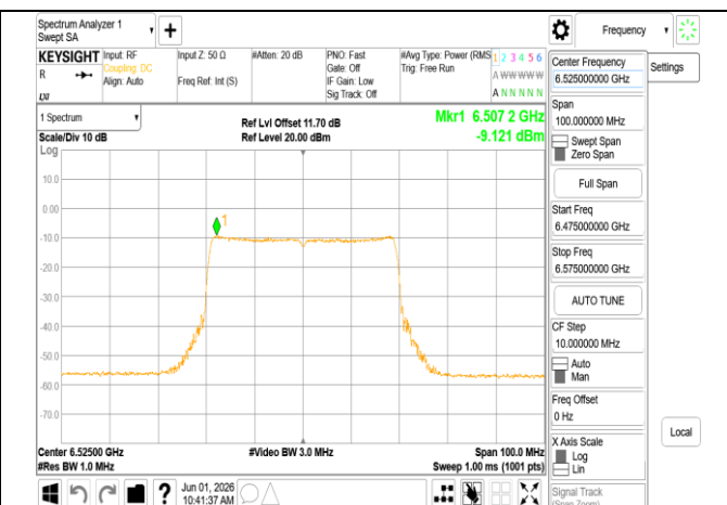
802.11be 40MHz Chain0 6525MHz RU484
