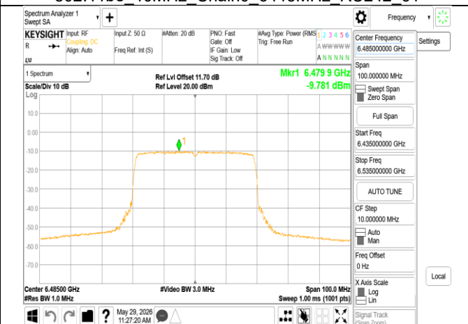
802.11be 40MHz Chain0 6485MHz
