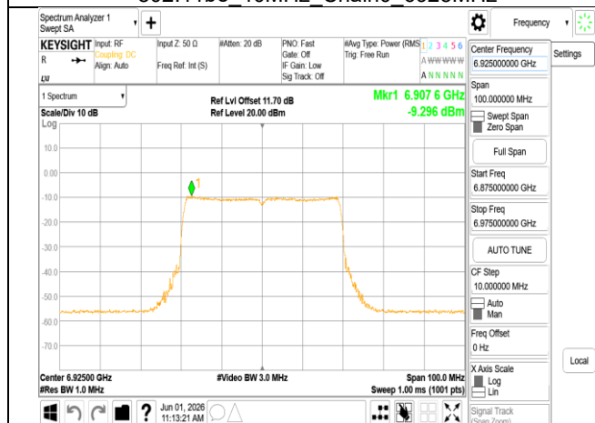
802.11be 40MHz Chain0 6925MHz RU484
