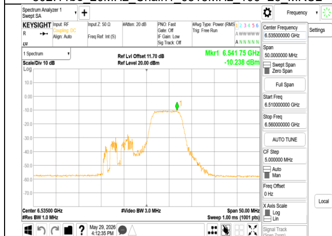
802.11be_20MHz_Chain1_6535MHz_52+26_MR1U1
