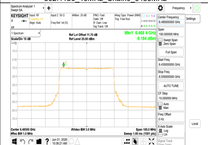
802.11be 40MHz Chain0 6485MHz RU484
