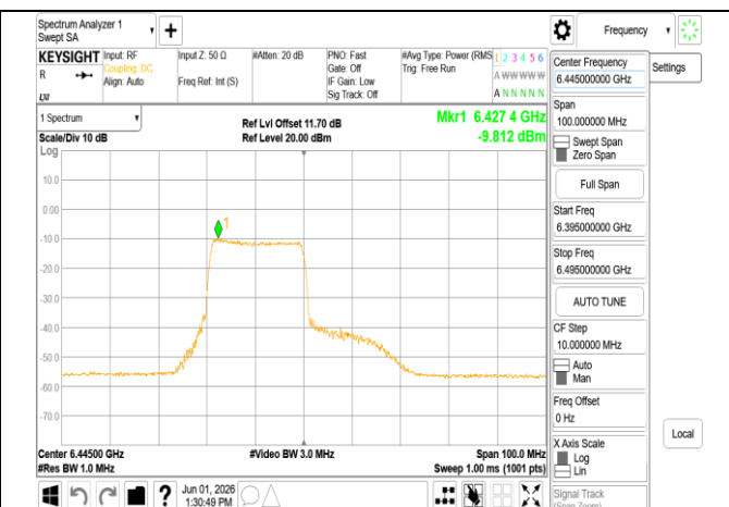
802.11be 40MHz Chain0 6445MHz RU242 61
