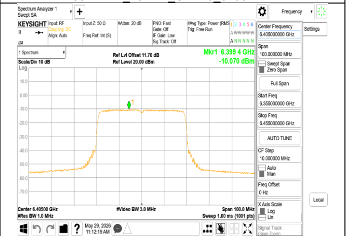
802.11be 40MHz Chain0 6405MHz
