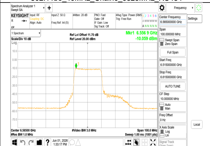
802.11be 40MHz Chain0 6565MHz RU242 61
