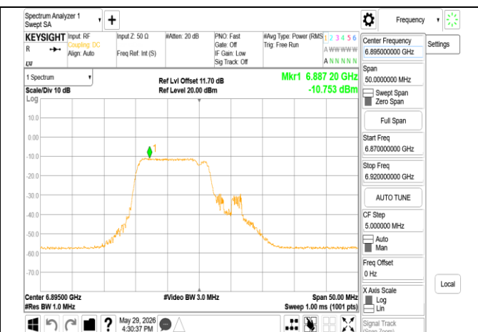
802.11be 20MHz Chain1 6895MHz 106+26 MRU1
