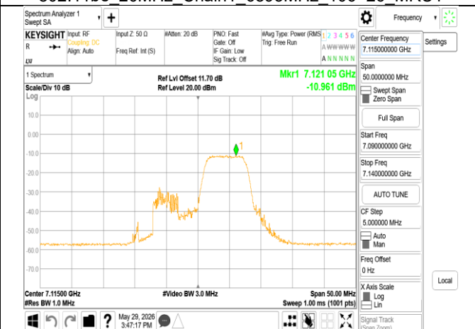
802.11be 20MHz Chain1 7115MHz 52+26 MRU3
