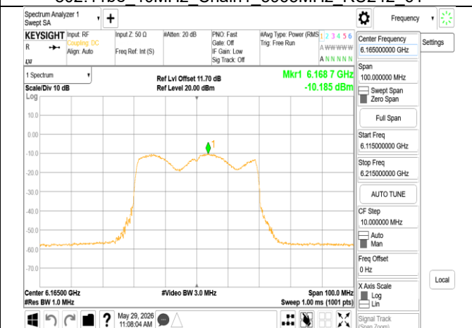
802.11be 40MHz Chain1 6165MHz
