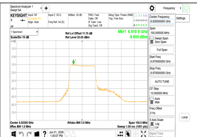
802.11be 40MHz Chain0 6925MHz RU242 61
