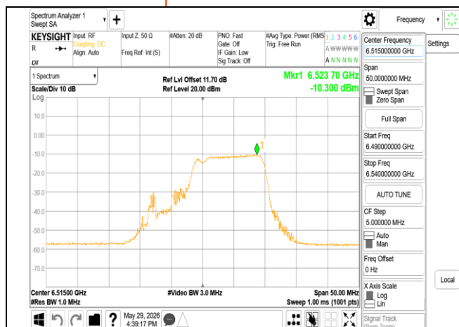
802.11be_20MHz_Chain1_6515MHz_106+26_MR1U2
