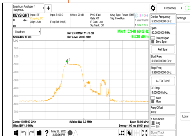
802.11be_20MHz_Chain1_5955MHz_52+26_MRUI
