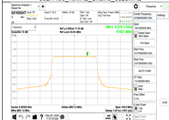
802.11be 40MHz Chain0 6565MHz
