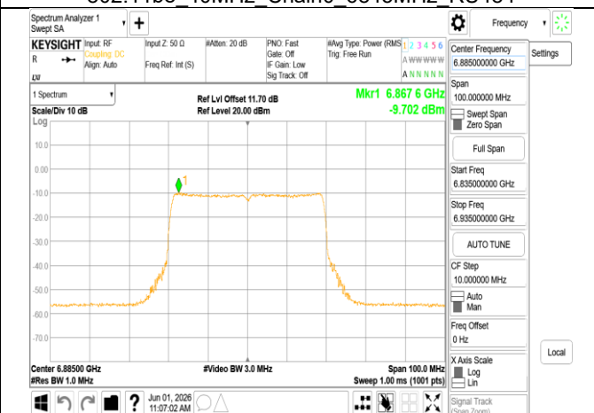
802.11be 40MHz Chain0 6885MHz RU484
