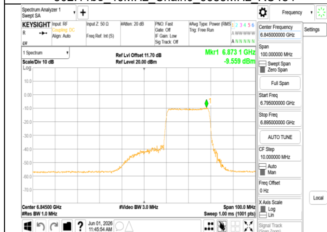
802.11be 40MHz Chain0 6845MHz RU242 62
