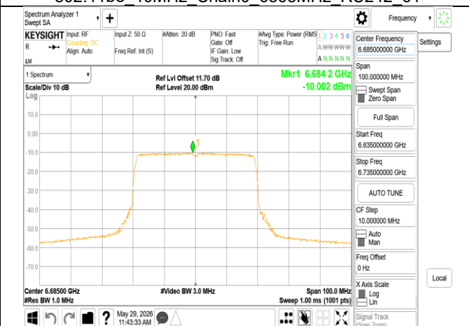
802.11be 40MHz Chain0 6685MHz
