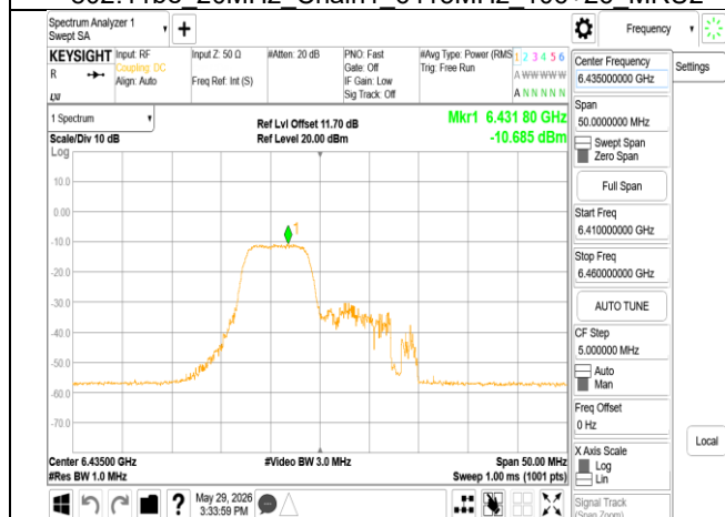
802.11be_20MHz_Chain1_6435MHz_52+26_MRUI
