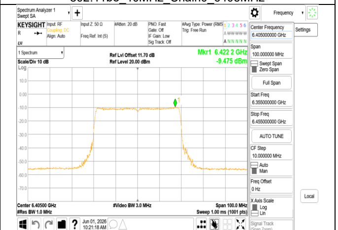
802.11be 40MHz Chain0 6405MHz RU484
