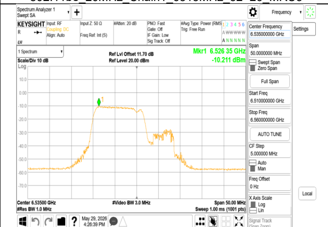
802.11be_20MHz_Chain1_6535MHz_106+26_MR1U1
