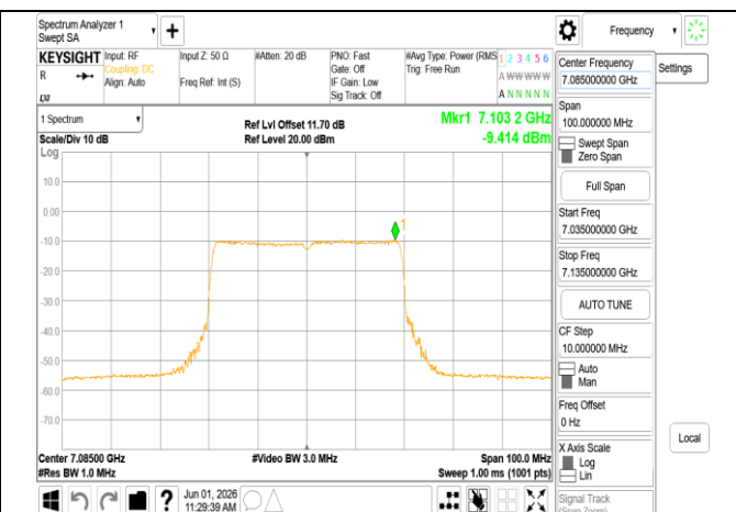
802.11be 40MHz Chain0 7085MHz RU484
