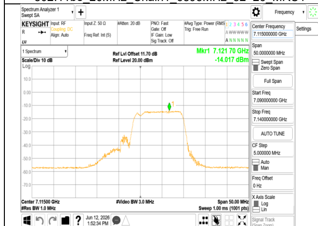
802.11be_20MHz_Chain1_7115MHz_106+26_MRUI
