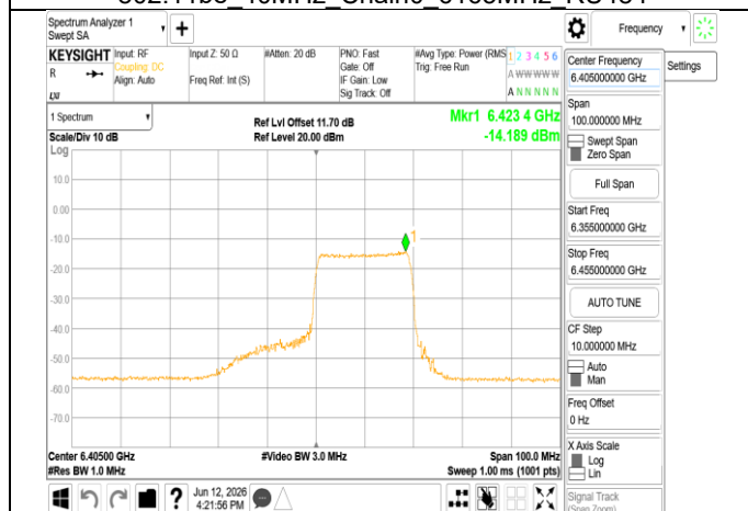
802.11be 40MHz Chain0 6405MHz RU242 62
