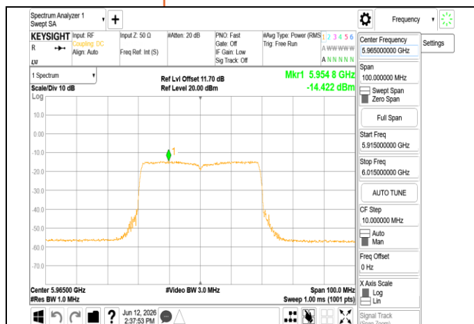
802.11be 40MHz Chain0 5965MHz RU484
