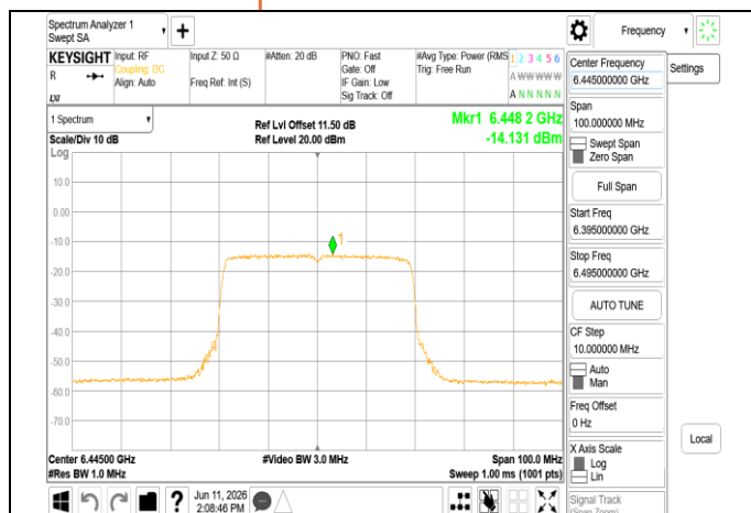
802.11be 40MHz Chain0 6445MHz
