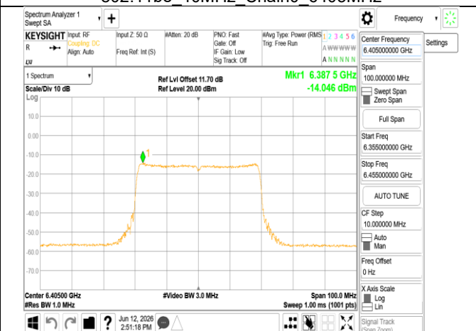
802.11be 40MHz Chain0 6405MHz RU484
