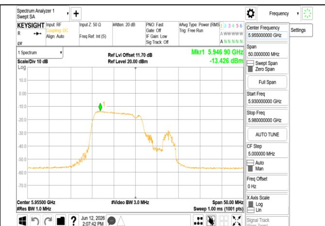
802.11be_20MHz_Chain1_5955MHz_106+26_MRU1
