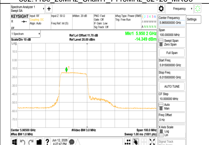
802.11be_40MHz_Chain0_5965MHz_RU242_61
