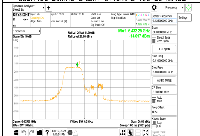
802.11be_20MHz_Chain1_6435MHz_52+26_MRU1
