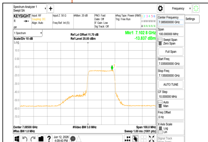
802.11be 40MHz Chain0 7085MHz RU242 62
