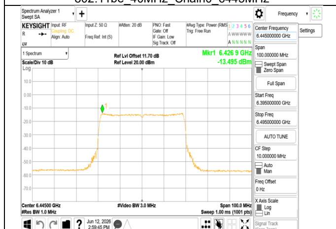
802.11be 40MHz Chain0 6445MHz RU484
