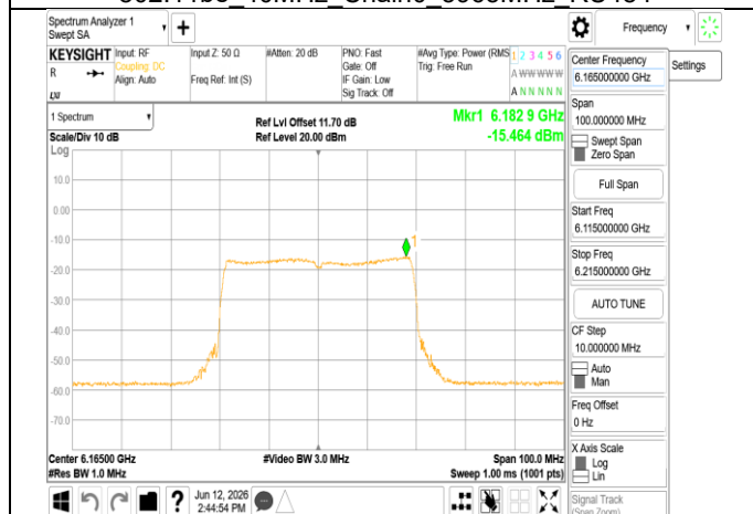
802.11be 40MHz Chain0 6165MHz RU484
