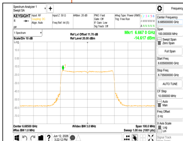
802.11be 40MHz Chain0 6685MHz RU484
