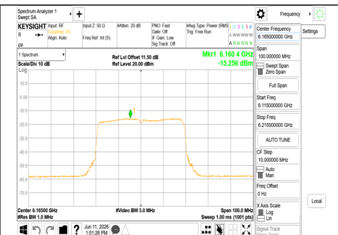
802.11be 40MHz Chain0 6165MHz
