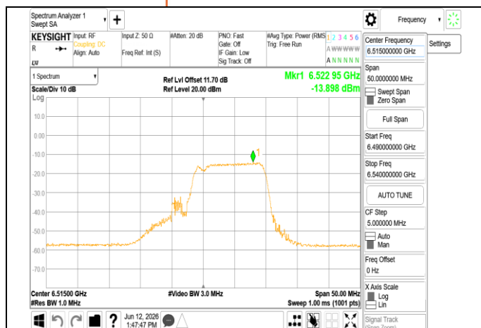
802.11be_20MHz_Chain1_6515MHz_106+26_MR1U2
