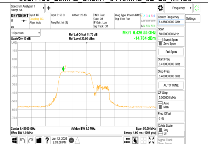
802.11be_20MHz_Chain1_6435MHz_106+26_MRU1
