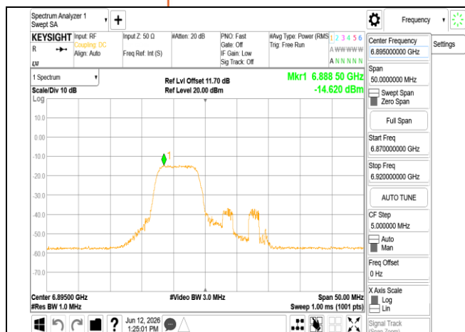
802.11be_20MHz_Chain1_6895MHz_52+26_MRUI
