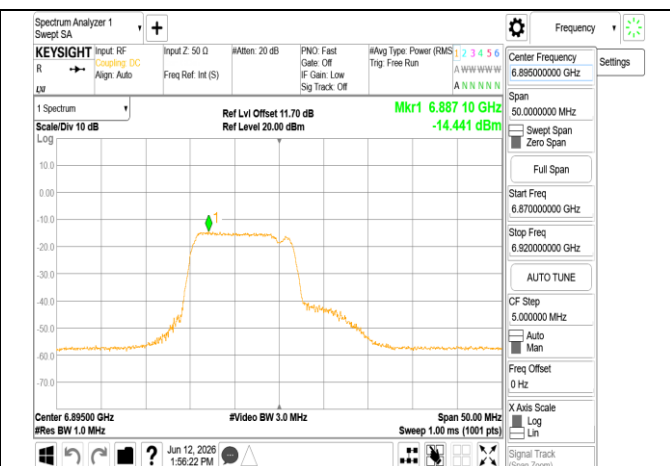
802.11be_20MHz_Chain1_6895MHz_106+26_MRUI
