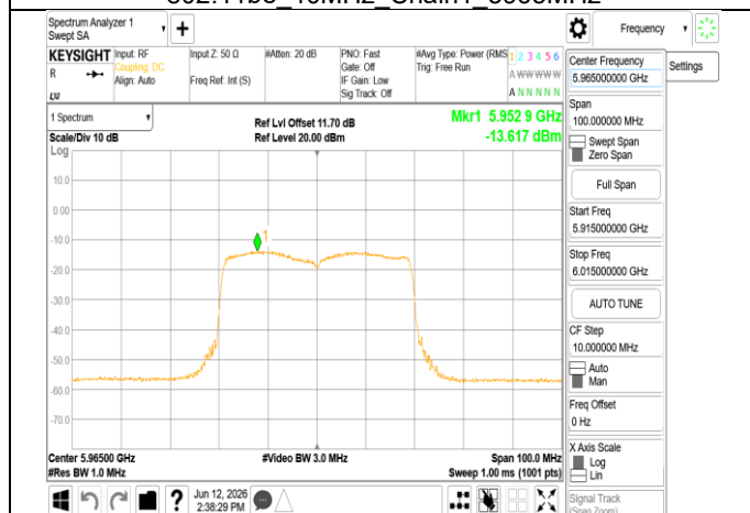
802.11be 40MHz Chain1 5965MHz RU484
