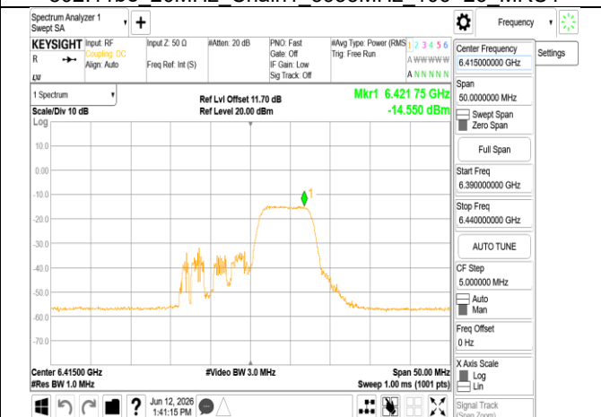
802.11be_20MHz_Chain1_6415MHz_52+26_MRU3
