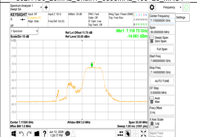
802.11be_20MHz_Chain1_7115MHz_52+26_MRUI
