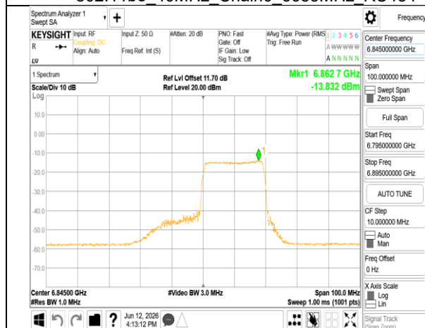
802.11be 40MHz Chain0 6845MHz RU242 62
