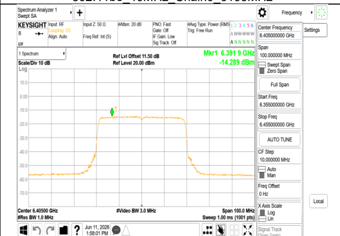
802.11be 40MHz Chain0 6405MHz
