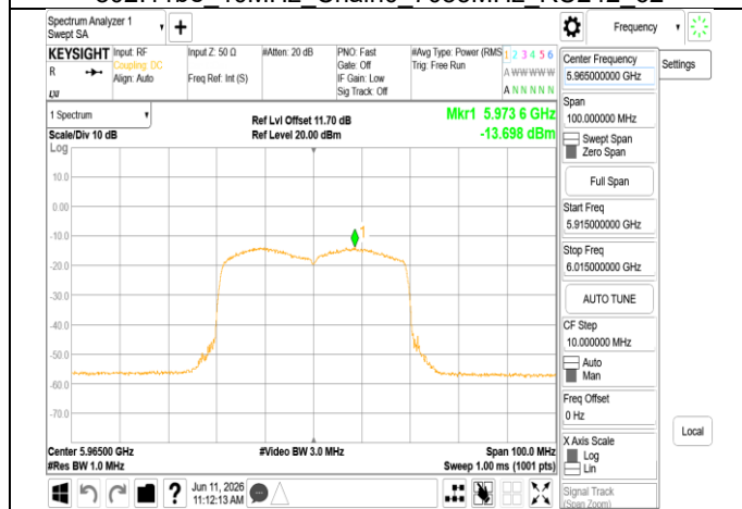
802.11be 40MHz Chain1 5965MHz
