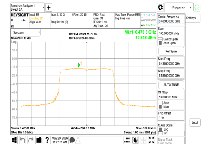
802.11be 40MHz Chain1 6485MHz
