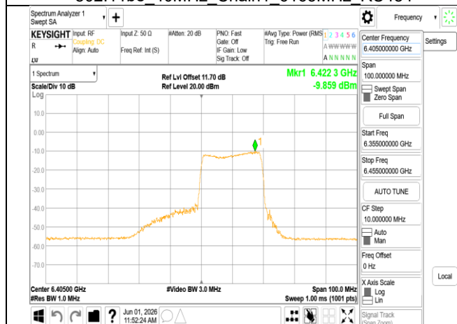
802.11be 40MHz Chain1 6405MHz RU242 62
