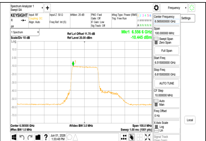
802.11be 40MHz Chain1_6565MHz_RU242_61
