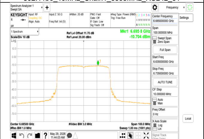
802.11be 40MHz Chain1_6685MHz
