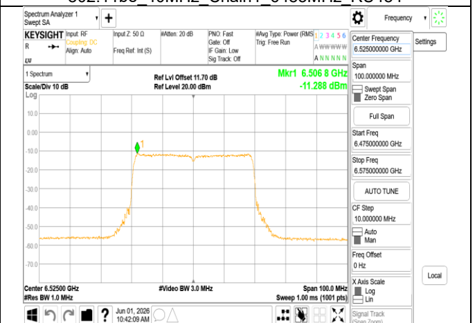
802.11be 40MHz Chain1 6525MHz RU484
