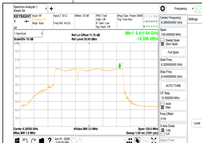
802.11be 80MHz Chain1 6385MHz 484+242 MRU1
