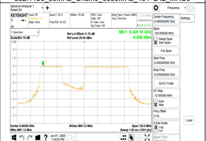
802.11be 80MHz Chain0 6465MHz 484+242 MRU2
