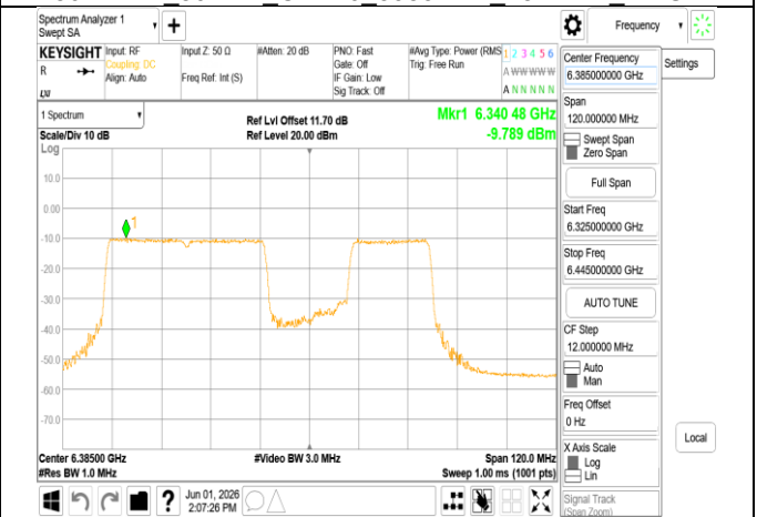
802.11be 80MHz Chain0 6385MHz 484+242 MRU3
