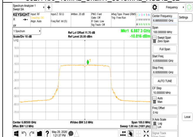
802.11be 40MHz Chain1 6885MHz
