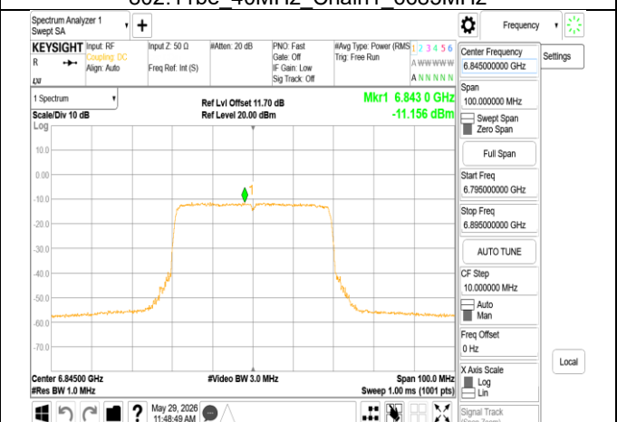
802.11be 40MHz Chain1_6845MHz
