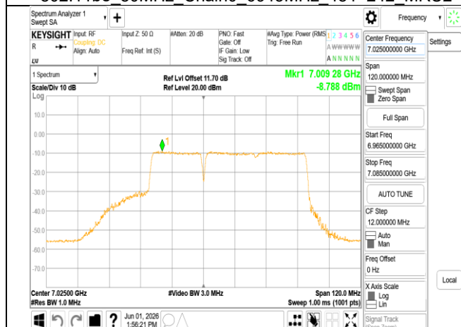
802.11be 80MHz Chain0 7025MHz 484+242 MRU1
