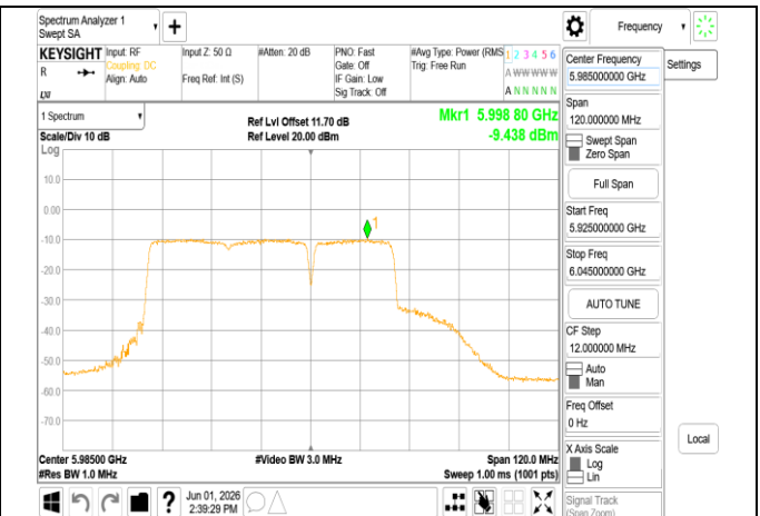
802.11be 80MHz Chain0 5985MHz 484+242 MRU4
