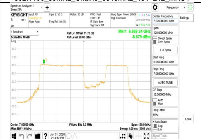
802.11be 80MHz Chain0 7025MHz 484+242 MRU3
