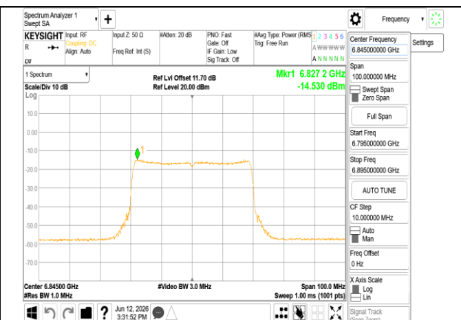
802.11be 40MHz Chain1 6845MHz RU484
