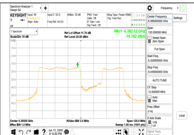
802.11be 80MHz Chain1 6385MHz 484+242 MRU3
