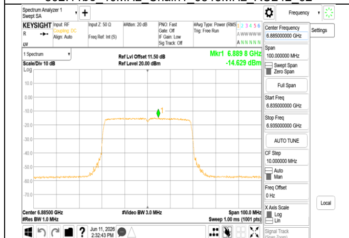
802.11be 40MHz Chain1 6885MHz
