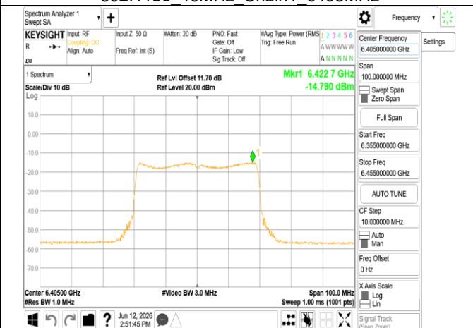
802.11be 40MHz Chain1 6405MHz RU484
