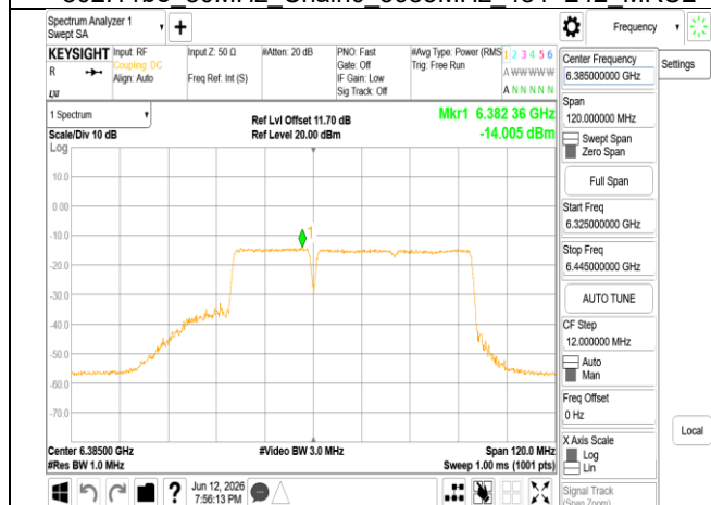
802.11be 80MHz Chain0 6385MHz 484+242 MRU1
