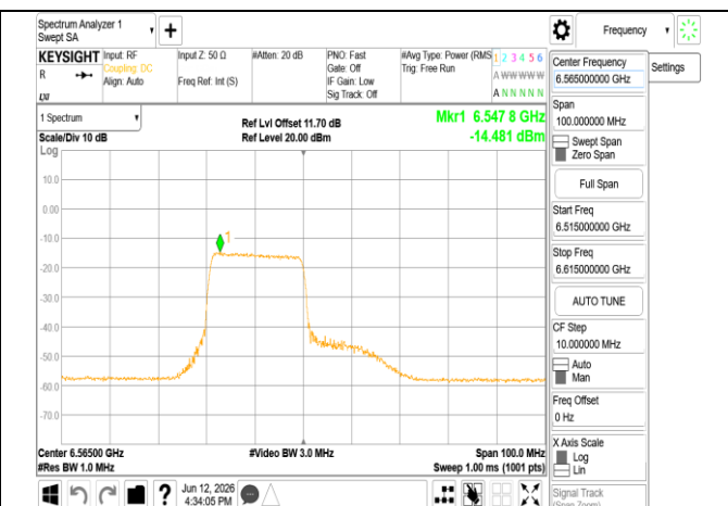
802.11be 40MHz Chain1 6565MHz RU242 61
