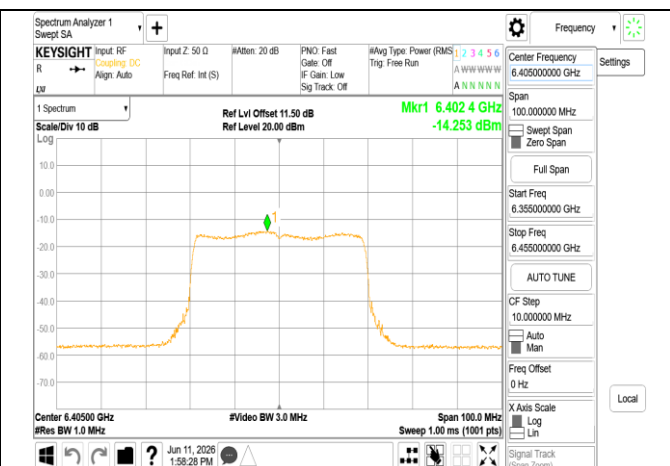
802.11be 40MHz Chain1 6405MHz
