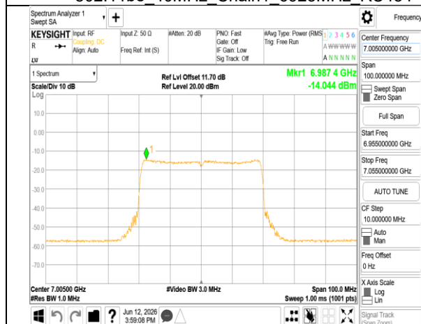
802.11be 40MHz Chain1 7005MHz RU484
