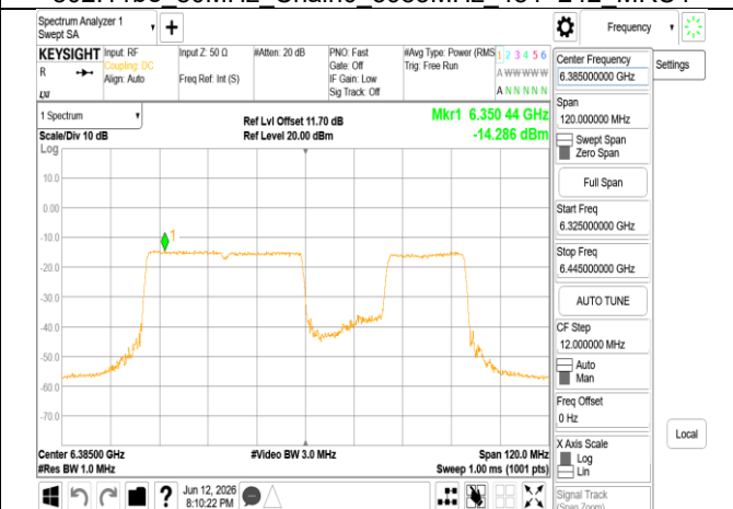
802.11be 80MHz Chain0 6385MHz 484+242 MRU3
