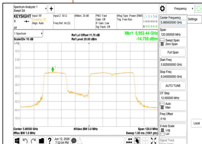
802.11be 80MHz Chain0 5985MHz 484+242 MRU2
