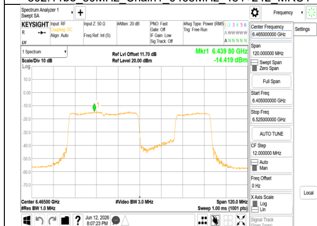
802.11be 80MHz Chain1 6465MHz 484+242 MRU3
