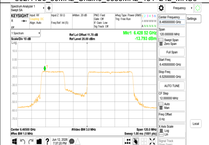
802.11be 80MHz Chain0 6465MHz 484+242 MRU2
