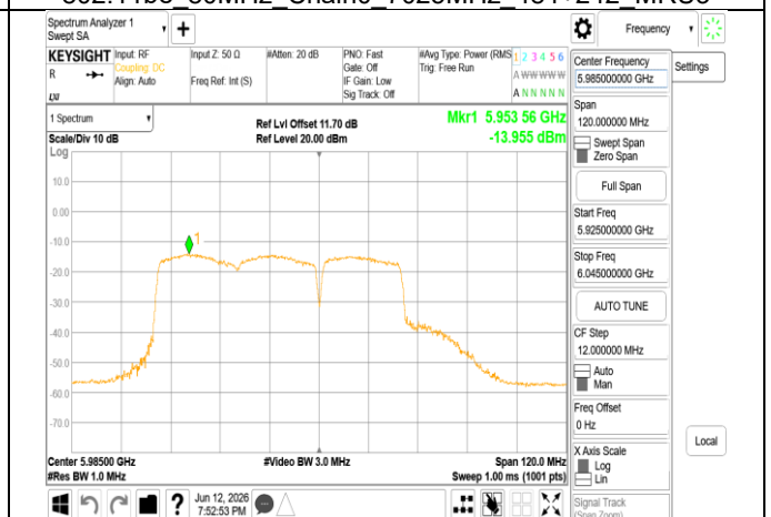
802.11be 80MHz Chain1 5985MHz 484+242 MRU4
