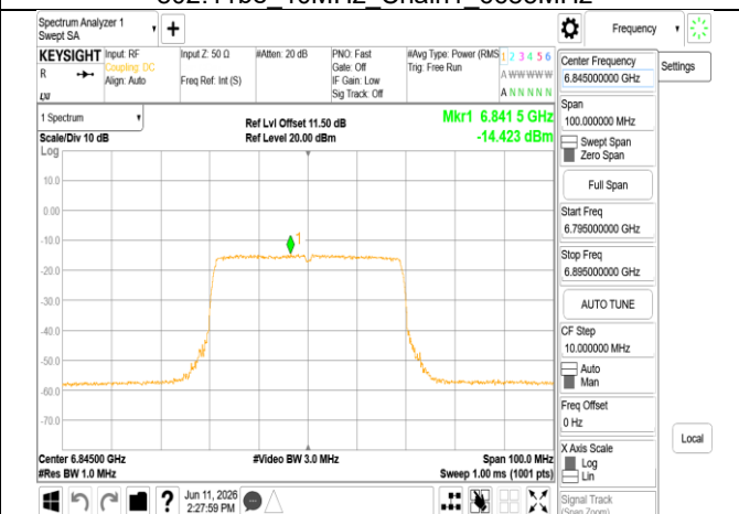
802.11be 40MHz Chain1 6845MHz
