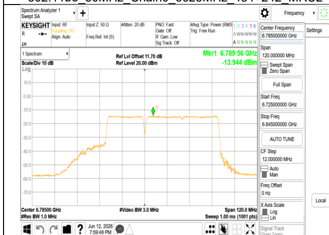
802.11be 80MHz Chain0_6785MHz 484+242 MRU1
