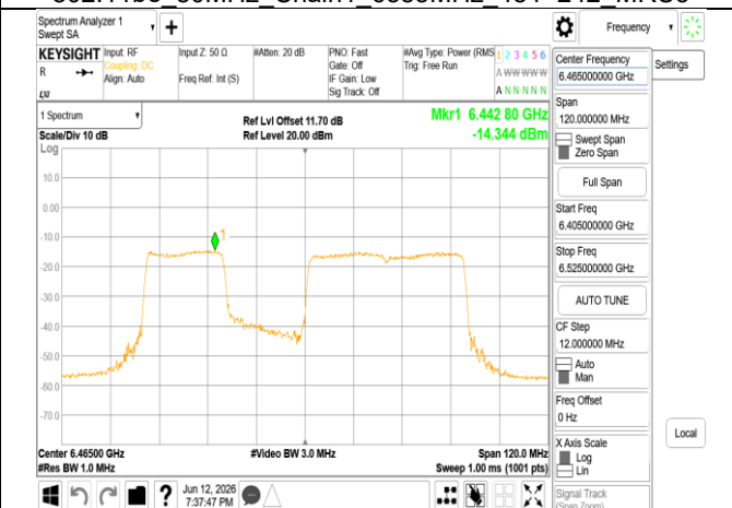
802.11be 80MHz Chain1 6465MHz 484+242 MRU2
