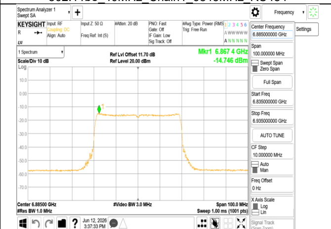
802.11be 40MHz Chain1 6885MHz RU484
