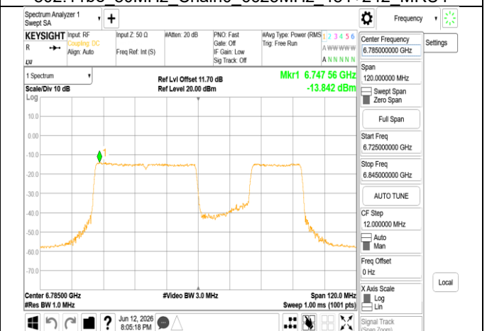
802.11be 80MHz Chain0_6785MHz 484+242 MRU3
