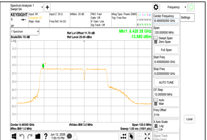
802.11be 80MHz Chain0_6465MHz 484+242 MRU4
