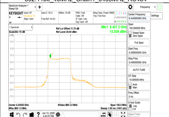
802.11be 40MHz Chain1 6445MHz RU242 61
