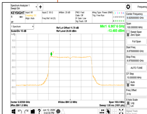
802.11be 40MHz Chain1 6925MHz RU484
