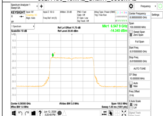
802.11be 40MHz Chain1 6565MHz RU484
