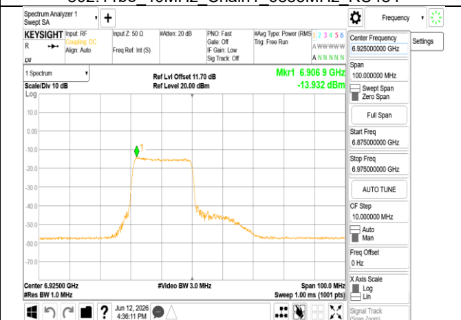
802.11be 40MHz Chain1 6925MHz RU242 61
