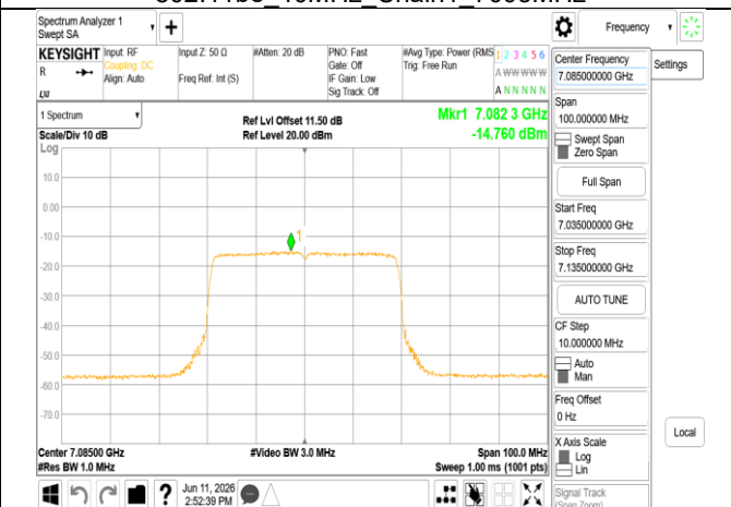
802.11be 40MHz Chain1 7085MHz
