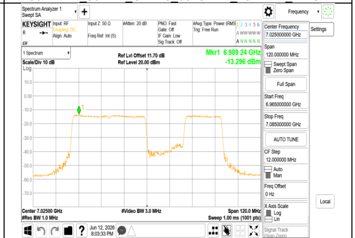
802.11be 80MHz Chain0 7025MHz 484+242 MRU3
