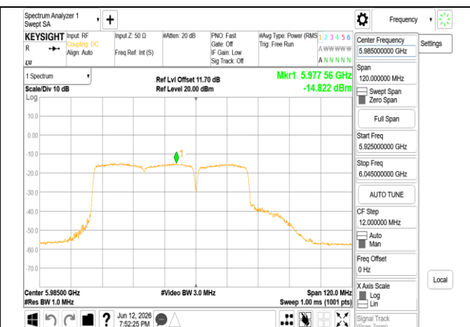
802.11be 80MHz Chain0 5985MHz 484+242 MRU4
