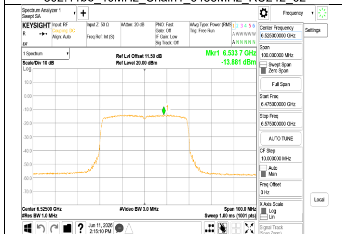
802.11be 40MHz Chain1 6525MHz
