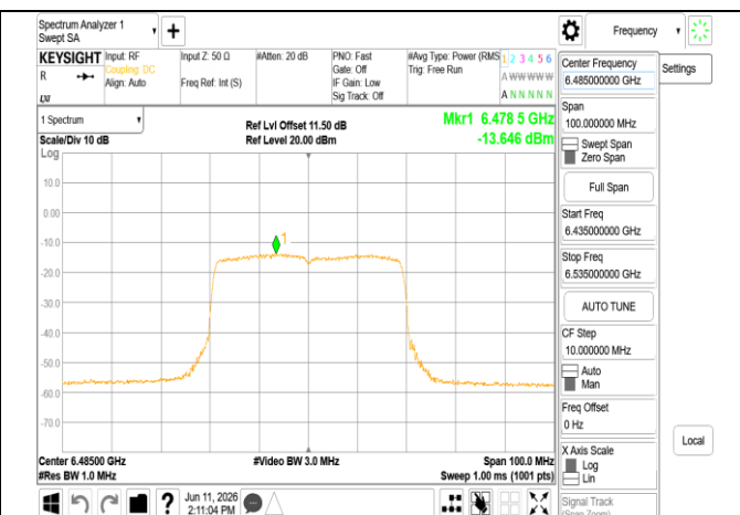
802.11be 40MHz Chain1 6485MHz
