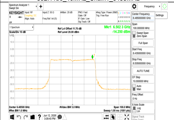
802.11be 40MHz Chain1 6485MHz RU484
