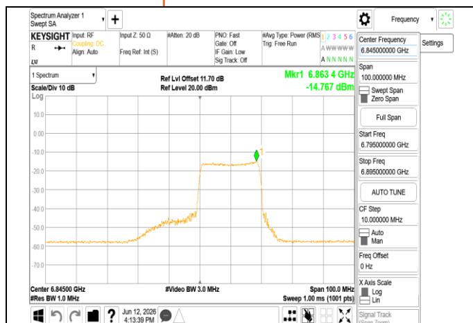
802.11be 40MHz Chain1 6845MHz RU242 62
