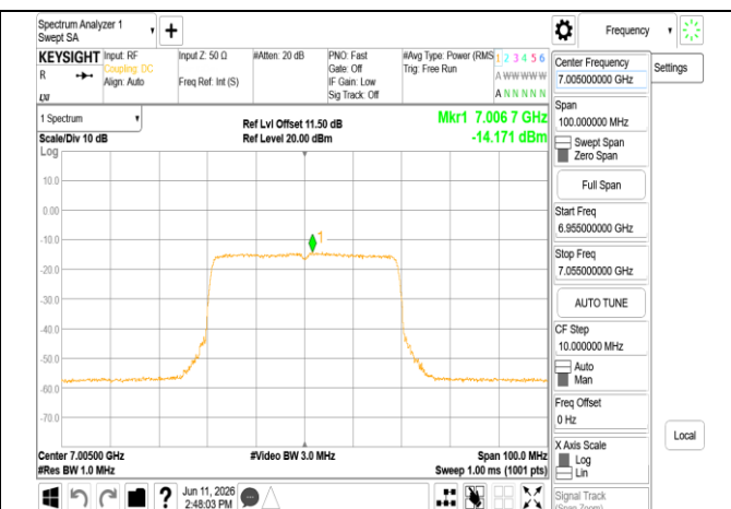
802.11be 40MHz Chain1 7005MHz
