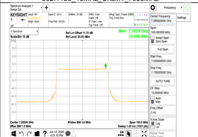
802.11be 40MHz Chain1 7085MHz RU484
