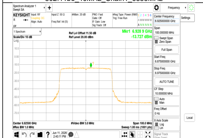
802.11be 40MHz Chain1 6925MHz
