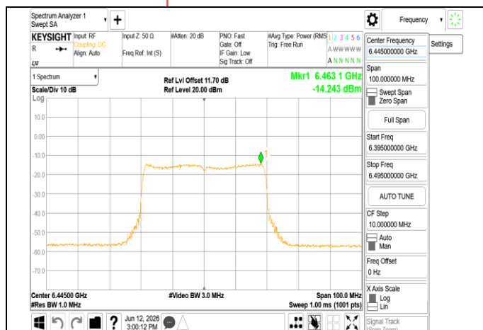
802.11be 40MHz Chain1 6445MHz RU484
