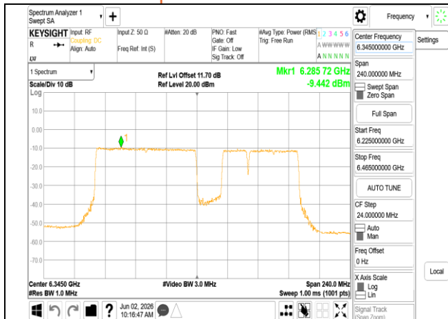
802.11be_160MHz_Chain0_6345MHz_996+484+242_MRU
