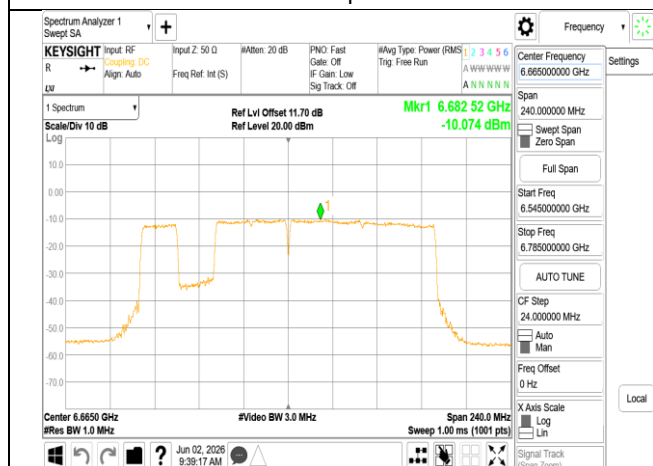
802.11be_160MHz_Chain0_6665MHz_996+484+242_MRU
