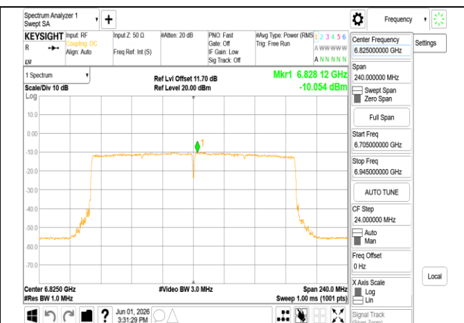
802.11be 160MHz Chain0 6825MHz RU996x2
