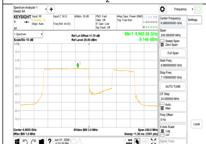
802.11be_160MHz_Chain0_6985MHz_996+484_MRU3
