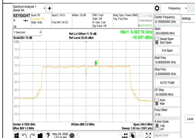
802.11be_160MHz_Chain0_6185MHz
