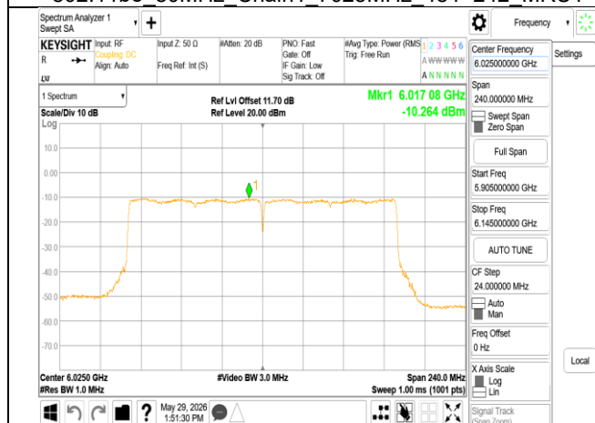
802.11be_160MHz_Chain0_6025MHz
