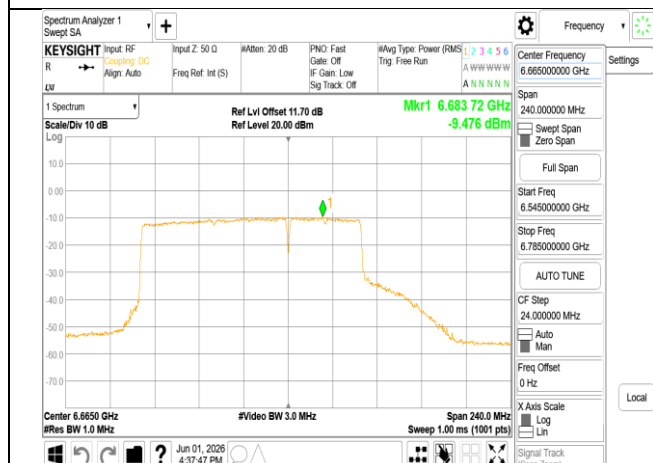
802.11be_160MHz_Chain0_6665MHz_996+484_MRU4
