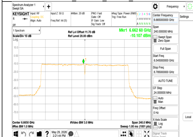
802.11be_160MHz_Chain0_6665MHz
