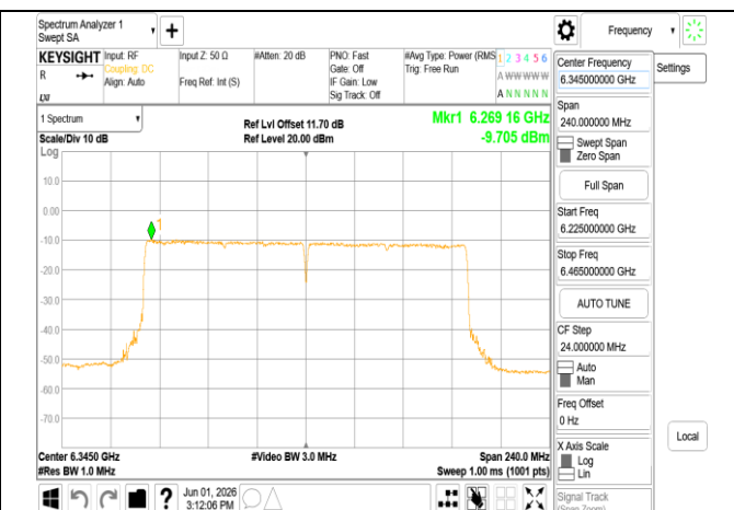
802.11be_160MHz_Chain0_6345MHz_RU996x2
