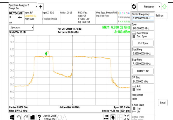
802.11be_160MHz_Chain0_6985MHz_996+484_MRU2
