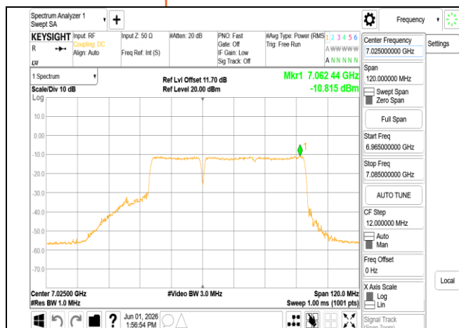
802.11be_80MHz_Chain1_7025MHz_484+242_MR1
