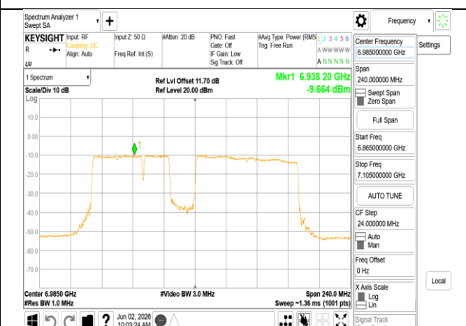
802.11be_160MHz_Chain0_6985MHz_996+484+242_MRU
