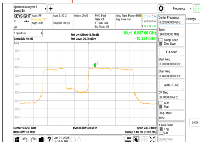
802.11be_160MHz_Chain0_6025MHz_996+484_MRU2
