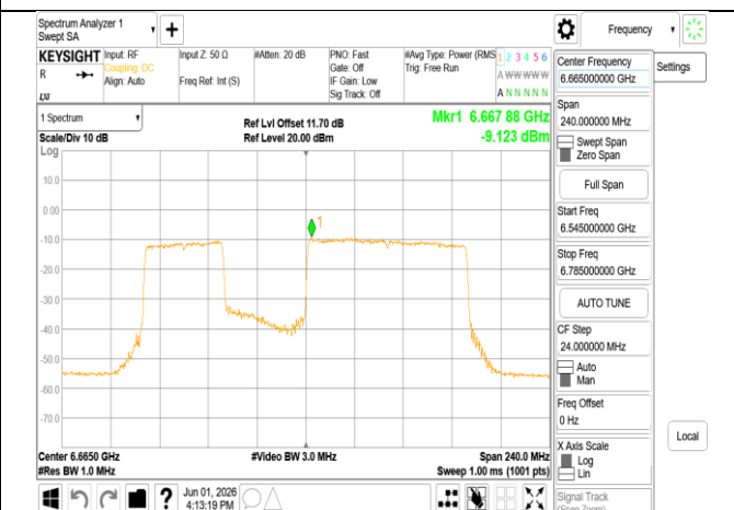
802.11be_160MHz_Chain0_6665MHz_996+484_MRU2
