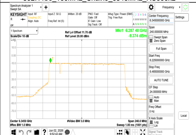
802.11be_160MHz_Chain0_6345MHz_996+484+242_MRU
