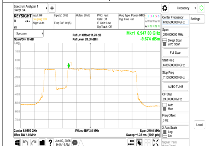
802.11be_160MHz_Chain0_6985MHz_996+484+242_MRU
