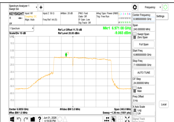
802.11be_160MHz_Chain0_6985MHz_996+484_MRU1
