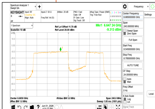
802.11be_160MHz_Chain0_6665MHz_996+484_MRU3
