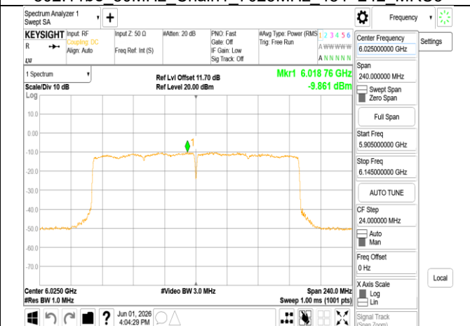
802.11be_160MHz_Chain0_6025MHz_RU996x2
