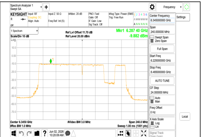
802.11be_160MHz_Chain0_6345MHz_996+484+242_MRU
