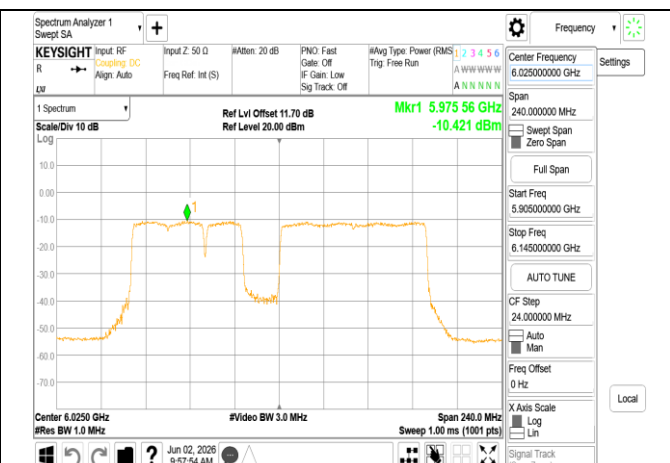
802.11be_160MHz_Chain0_6025MHz_996+484+242_MRU
