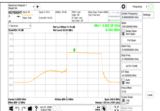
802.11be_160MHz_Chain0_6665MHz_RU996_S67
