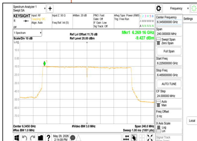
802.11be_160MHz_Chain0_6345MHz
