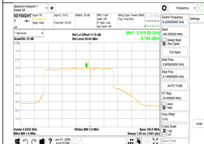
802.11be_160MHz_Chain0_6025MHz_996+484_MRU4
