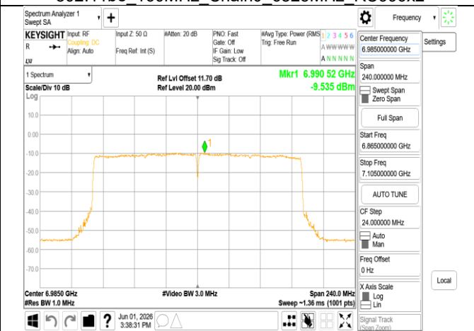
802.11be 160MHz Chain0 6985MHz RU996x2
