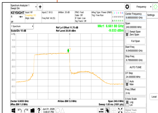
802.11be_160MHz_Chain0_6665MHz_RU996_67
