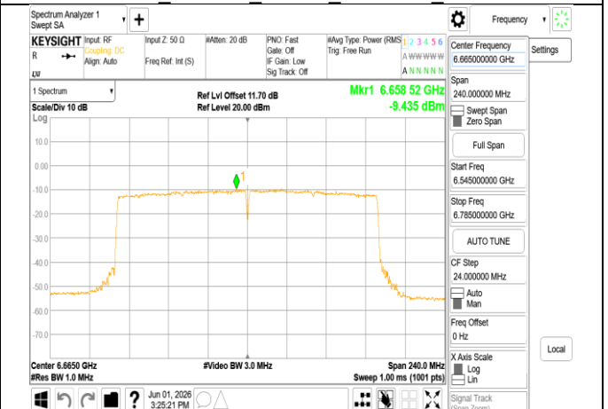
802.11be_160MHz_Chain0_6665MHz_RU996x2
