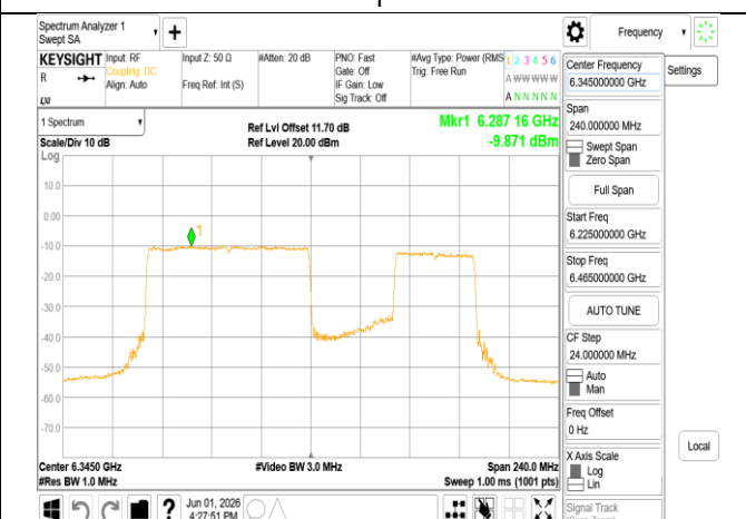
802.11be_160MHz_Chain0_6345MHz_996+484_MRU3
