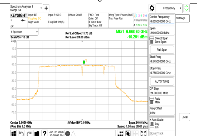
802.11be_160MHz_Chain0_6665MHz_996+484+242_MRU
