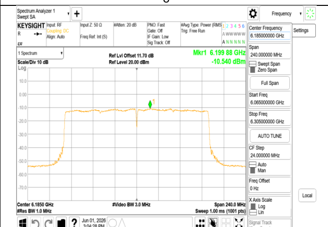
802.11be_160MHz_Chain0_6185MHz RU996x2
