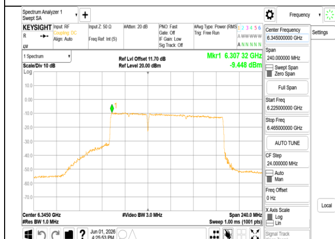
802.11be_160MHz_Chain0_6345MHz_996+484_MRU1
