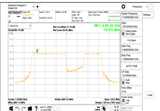
802.11be_80MHz_Chain1_7025MHz_484+242_MR3
