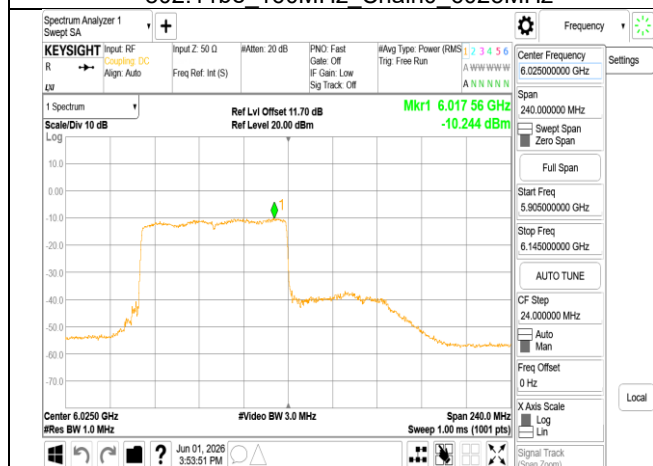
802.11be_160MHz_Chain0_6025MHz_RU996_67
