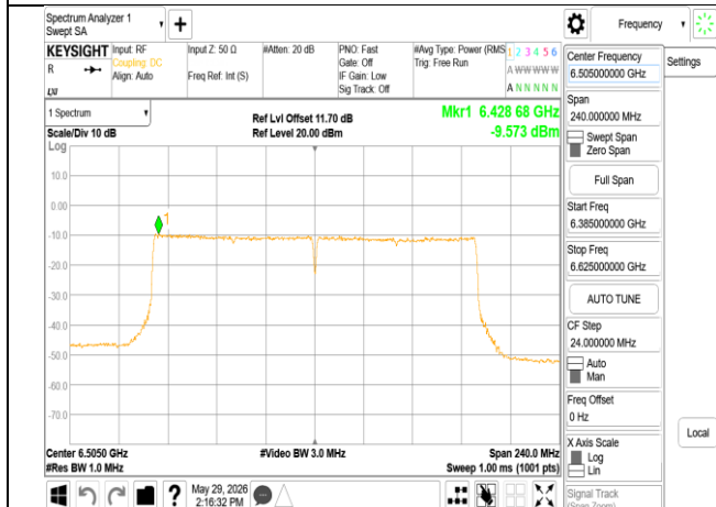
802.11be_160MHz_Chain0_6505MHz
