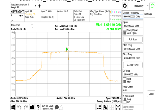
802.11be_160MHz_Chain0_6665MHz_996+484+242_MRU
