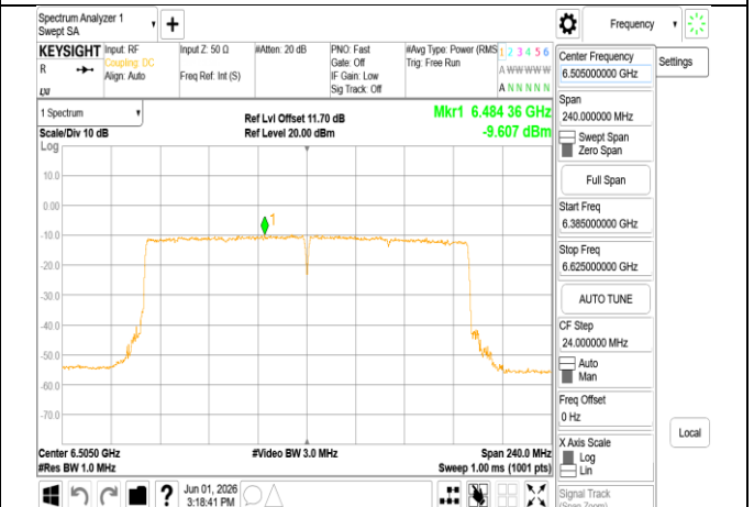
802.11be_160MHz_Chain0_6505MHz_RU996x2
