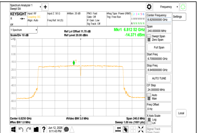
802.11be_160MHz_Chain0_6825MHz_RU996x2
