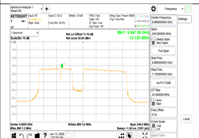
802.11be_160MHz_Chain0_6985MHz_996+484+242_MRU
