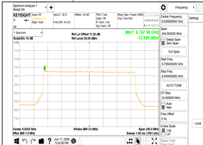
802.11be_160MHz_Chain0_6825MHz
