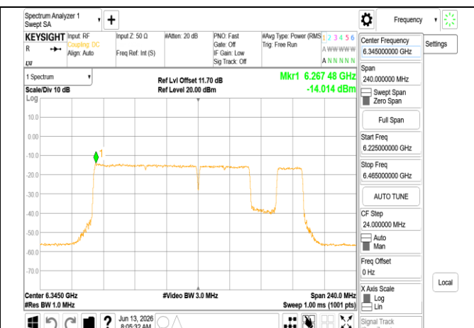
802.11be_160MHz_Chain0_6345MHz_996+484+242_MRU
