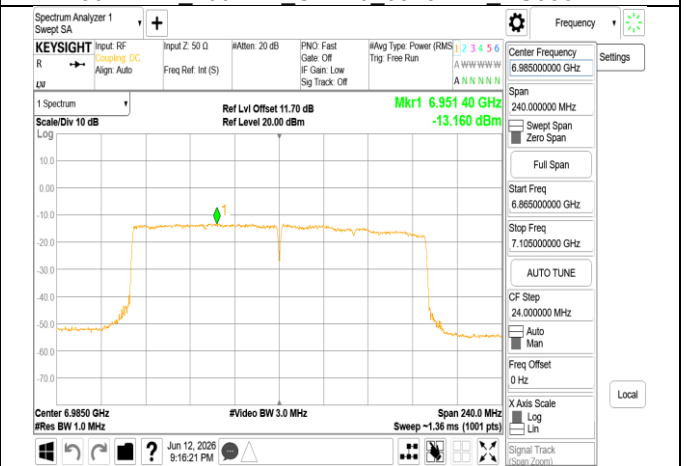
802.11be_160MHz_Chain0_6985MHz_RU996x2
