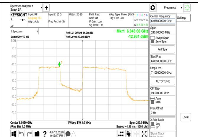
802.11be_160MHz_Chain0_6985MHz_996+484_MRU2
