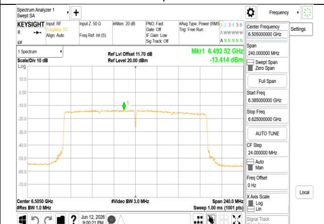
802.11be_160MHz_Chain0_6505MHz_RU996x2
