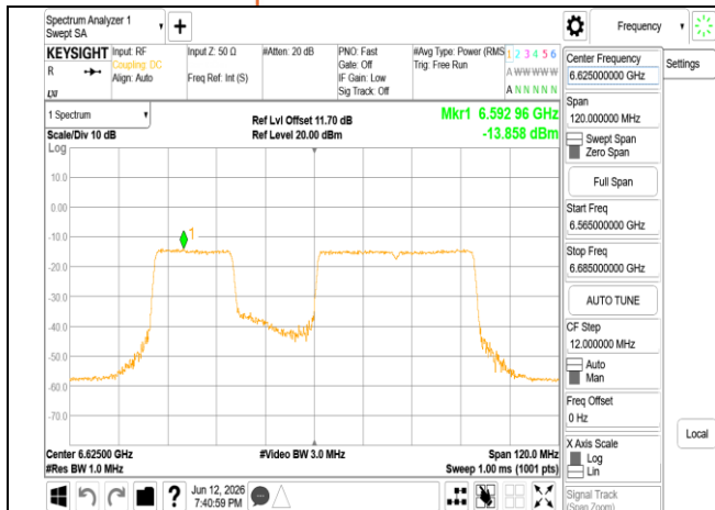
802.11be 80MHz Chain1 6625MHz 484+242 MRU2
