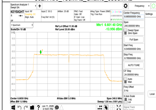
802.11be_160MHz_Chain0_6665MHz
