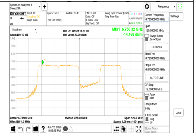
802.11be 80MHz Chain1 6785MHz 484+242 MRU3
