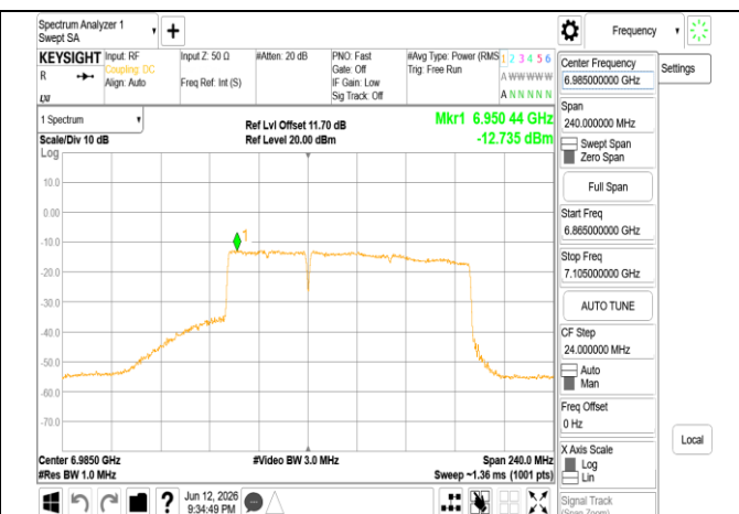
802.11be_160MHz_Chain0_6985MHz_996+484_MRU1
