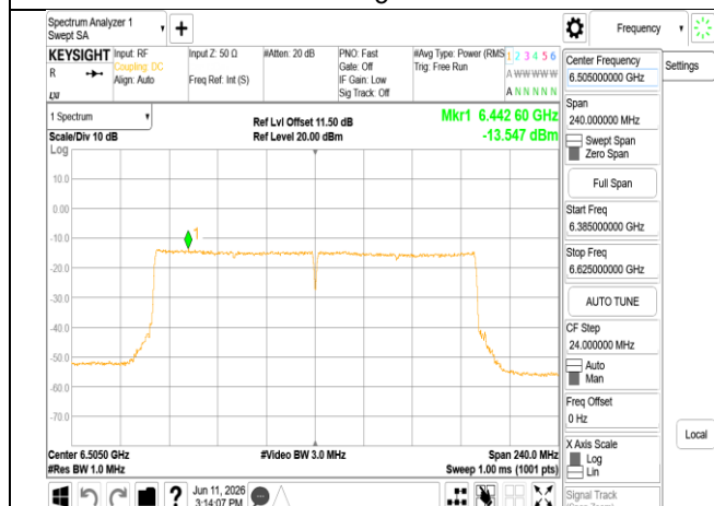
802.11be_160MHz_Chain0_6505MHz
