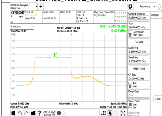
802.11be_160MHz_Chain0_6985MHz_RU996_67
