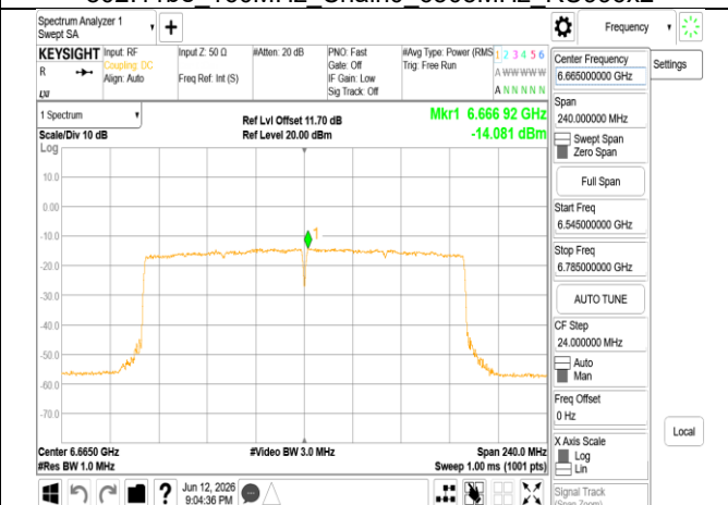
802.11be_160MHz_Chain0_6665MHz_RU996x2
