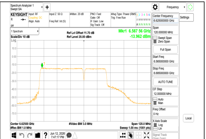
802.11be 80MHz Chain1 6625MHz 484+242 MRU4
