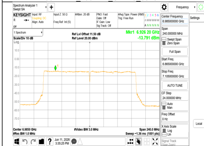
802.11be_160MHz_Chain0_6985MHz
