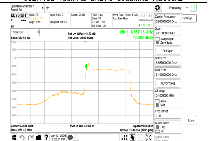
802.11be_160MHz_Chain0_6985MHz_RU996_S67
