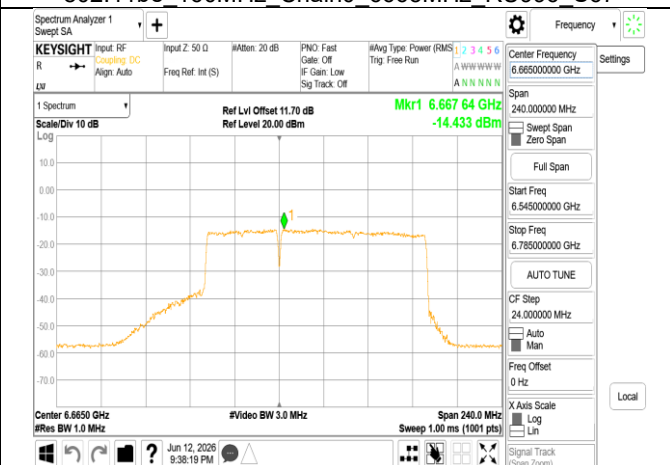
802.11be_160MHz_Chain0_6665MHz_996+484_MRU1
