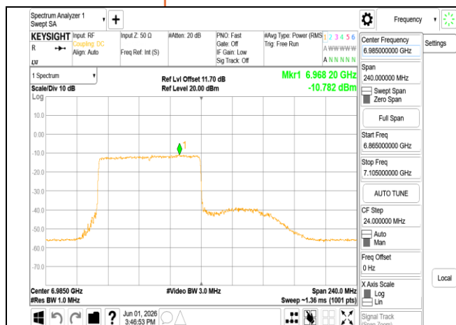
802.11be_160MHz_Chain1_6985MHz_RU996_67
