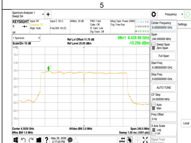
802.11be_160MHz_Chain1_6505MHz
