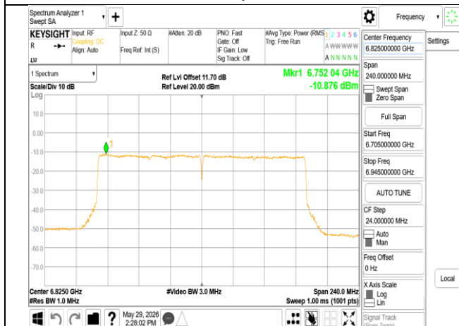
802.11be_160MHz_Chain1_6825MHz
