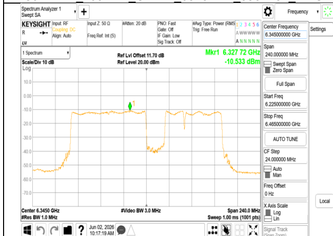
802.11be_160MHz_Chain1_6345MHz_996+484+242_MRU
