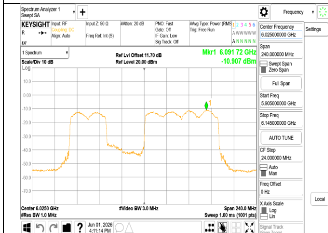
802.11be_160MHz_Chain1_6025MHz_996+484_MRU2
