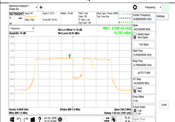
802.11be_160MHz_Chain1_6665MHz_996+484+242_MRU
