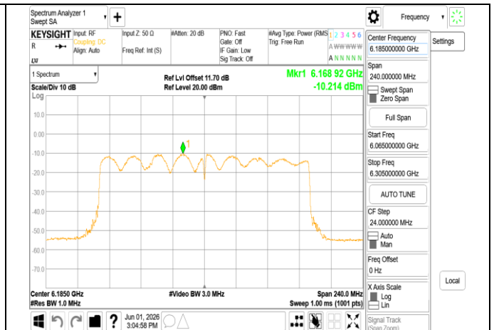
802.11be_160MHz_Chain1_6185MHz_RU996x2
