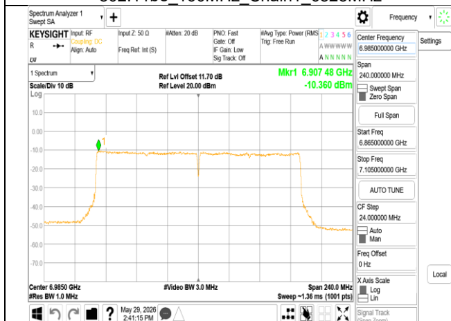
802.11be_160MHz_Chain1_6985MHz
