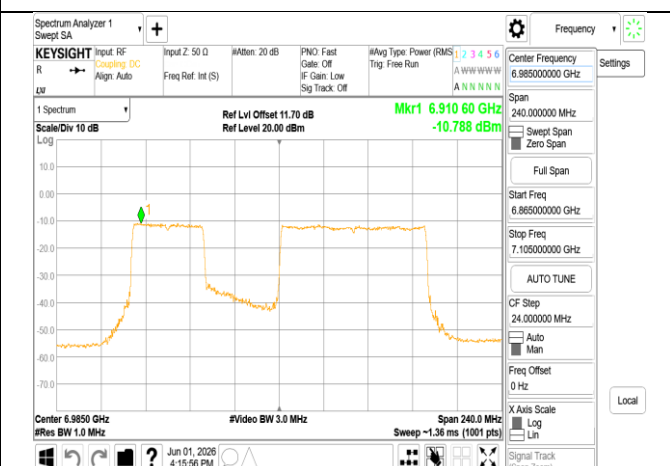
802.11be_160MHz_Chain1_6985MHz_996+484_MRU2
