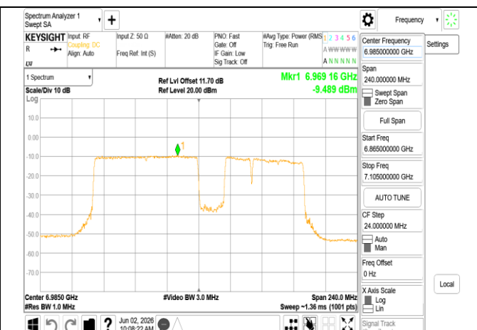
802.11be_160MHz_Chain0_6985MHz_996+484+242_MRU
