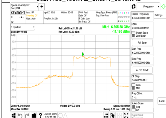
802.11be_160MHz_Chain1_6345MHz_RU996_S67
