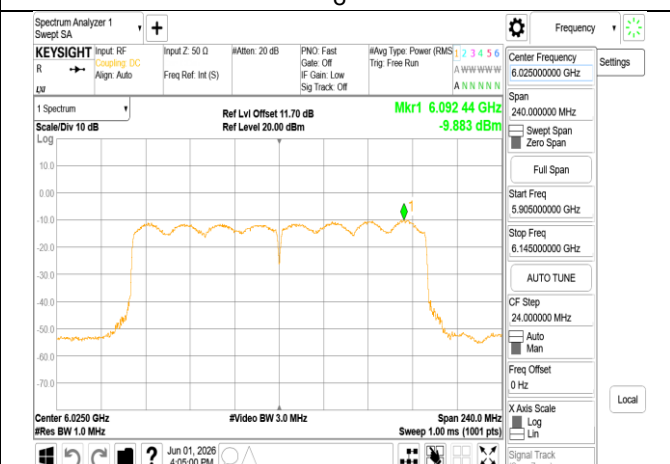
802.11be_160MHz_Chain1_6025MHz RU996x2
