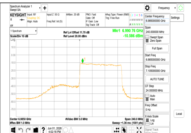
802.11be_160MHz_Chain1_6985MHz_RU996_S67
