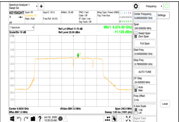
802.11be_160MHz_Chain1_6665MHz_996+484+242_MRU
