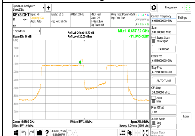
802.11be_160MHz_Chain1_6665MHz_996+484_MRU3
