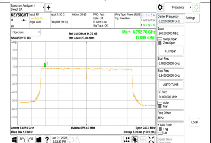
802.11be_160MHz_Chain1_6825MHz_RU996x2
