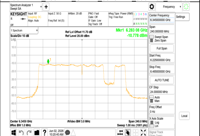
802.11be_160MHz_Chain1_6345MHz_996+484+242_MRU
