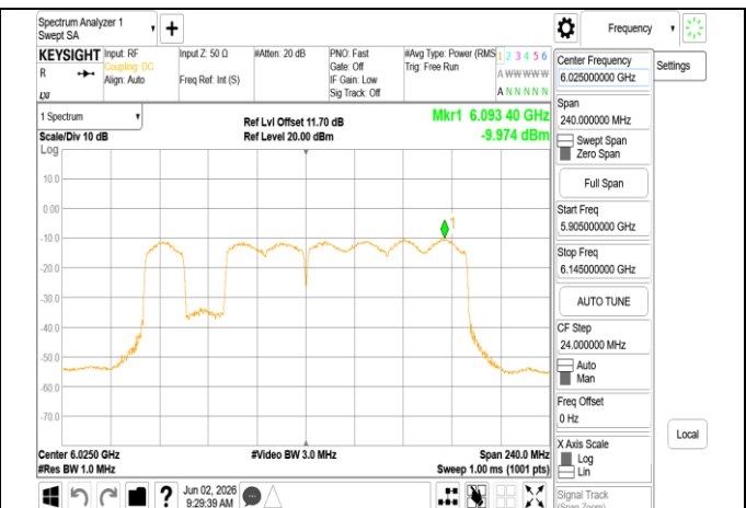
802.11be_160MHz_Chain1_6025MHz_996+484+242_MRU
