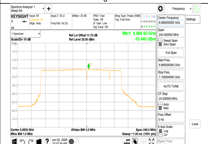
802.11be_160MHz_Chain1_6985MHz_996+484+242_MRU
