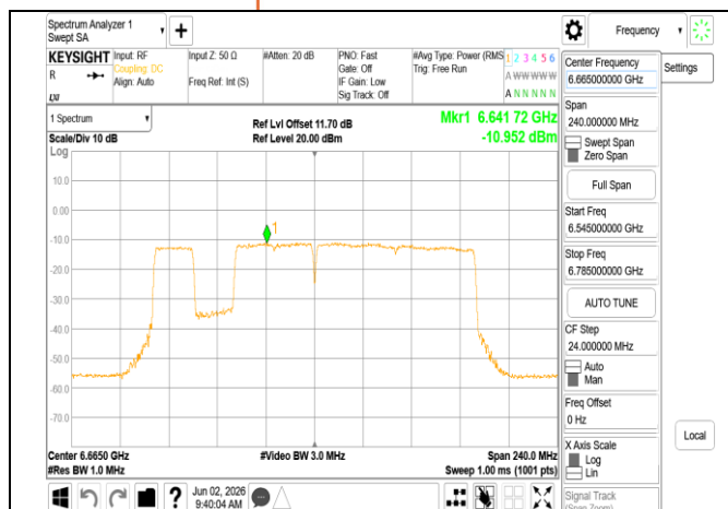
802.11be_160MHz_Chain1_6665MHz_996+484+242_MRU
