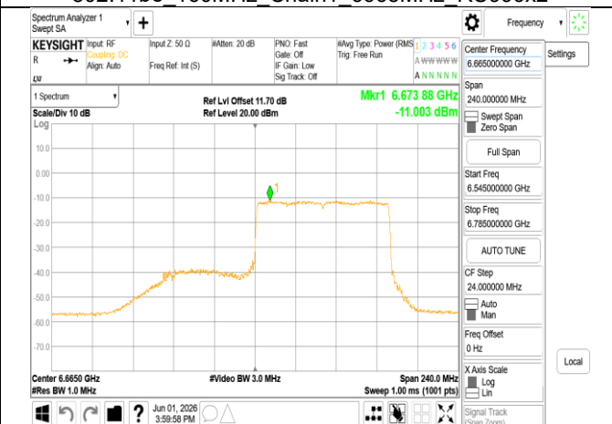
802.11be_160MHz_Chain1_6665MHz_RU996_S67
