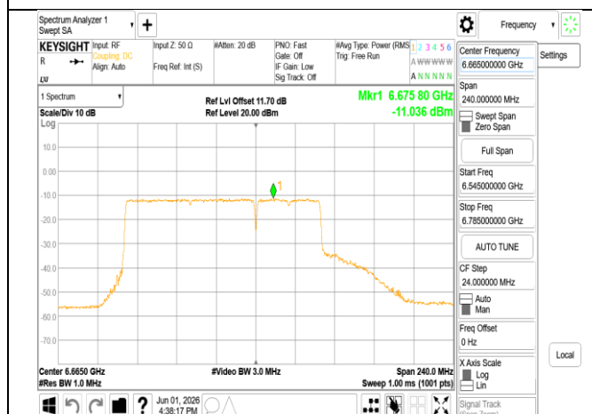
802.11be_160MHz_Chain1_6665MHz_996+484_MRU4
