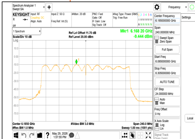
802.11be_160MHz_Chain1_6185MHz
