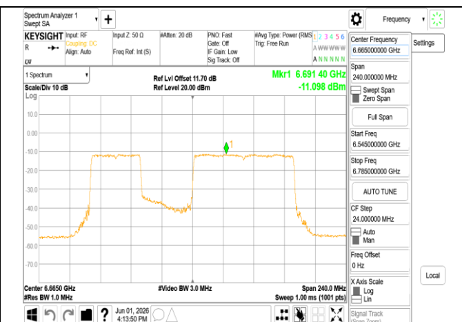
802.11be_160MHz_Chain1_6665MHz_996+484_MRU2
