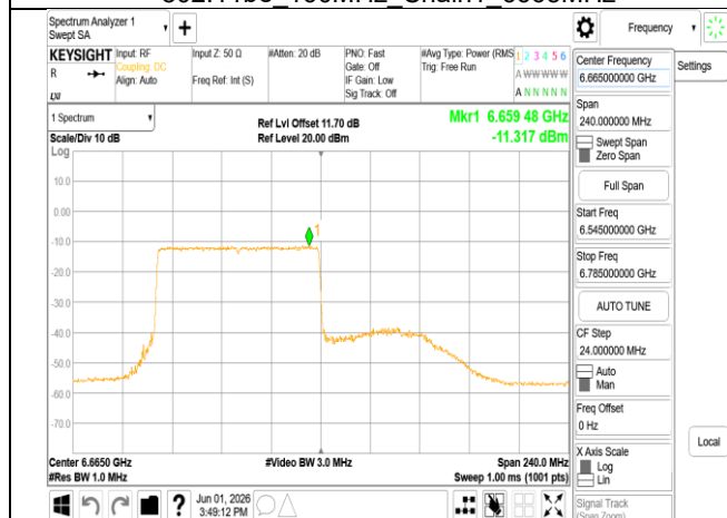
802.11be_160MHz_Chain1_6665MHz_RU996_67
