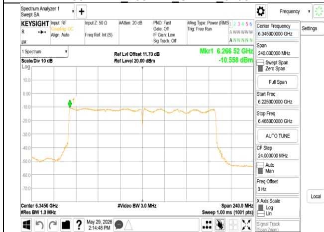
802.11be_160MHz_Chain1_6345MHz
