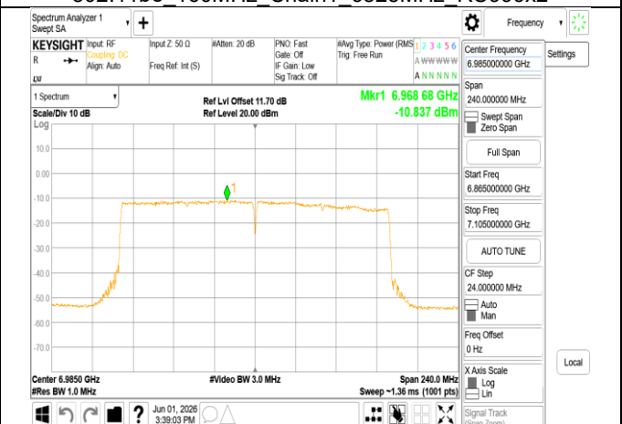
802.11be_160MHz_Chain1_6985MHz_RU996x2
