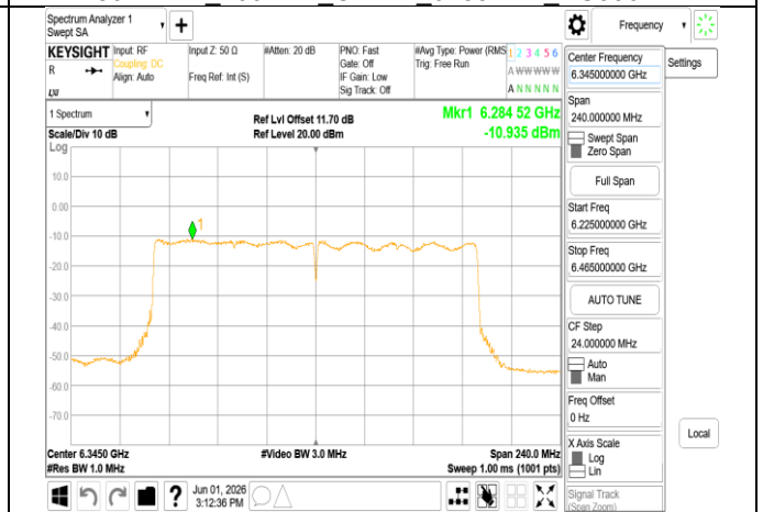
802.11be_160MHz_Chain1_6345MHz_RU996x2
