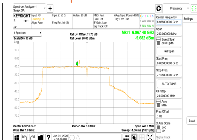
802.11be_160MHz_Chain0_6985MHz_996+484_MRU4
