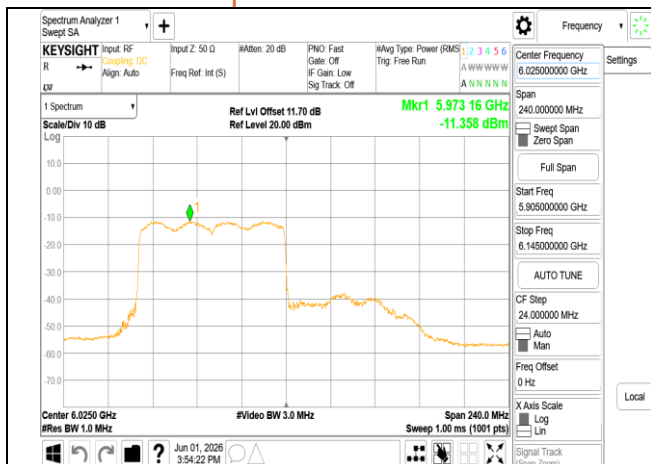
802.11be_160MHz_Chain1_6025MHz_RU996_67
