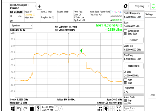
802.11be_160MHz_Chain1_6025MHz_996+484_MRU4
