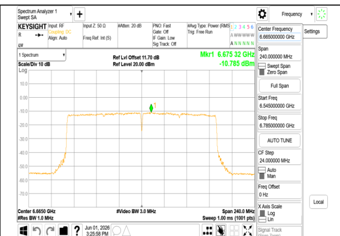
802.11be_160MHz_Chain1_6665MHz_RU996x2
