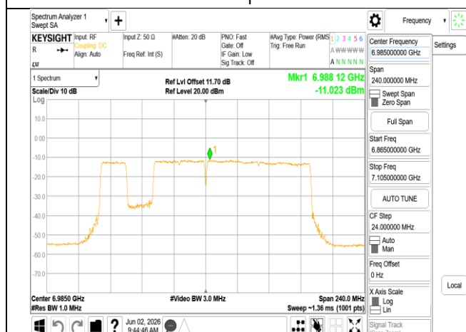
802.11be_160MHz_Chain1_6985MHz_996+484+242_MRU
