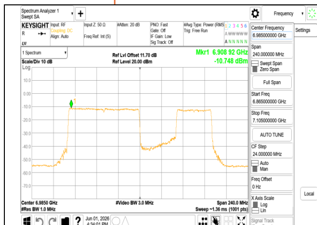
802.11be_160MHz_Chain1_6985MHz_996+484_MRU3
