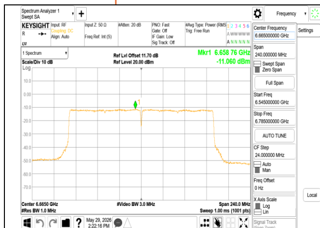
802.11be_160MHz_Chain1_6665MHz
