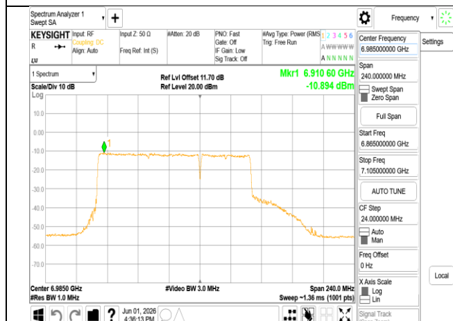
802.11be_160MHz_Chain1_6985MHz_996+484_MRU4
