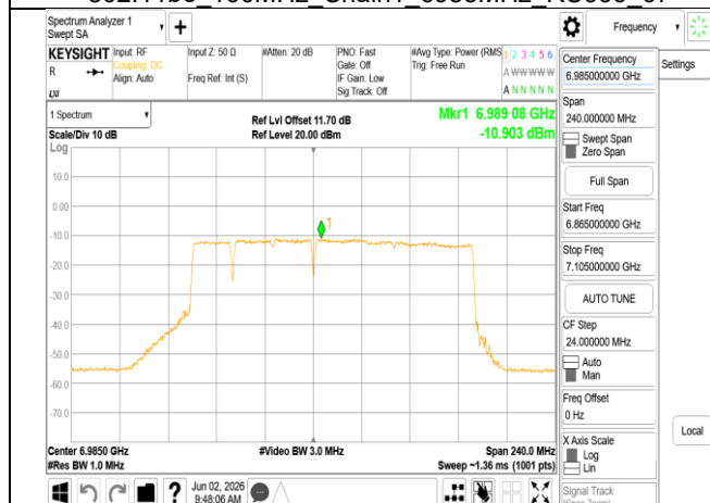
802.11be_160MHz_Chain1_6985MHz_996+484+242_MRU
