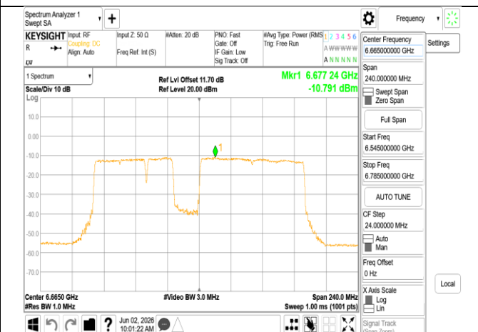
802.11be_160MHz_Chain1_6665MHz_996+484+242_MRU
