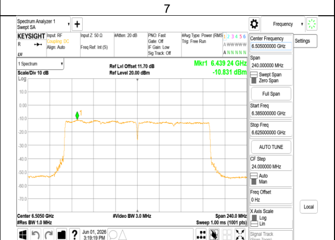
802.11be_160MHz_Chain1_6505MHz RU996x2
