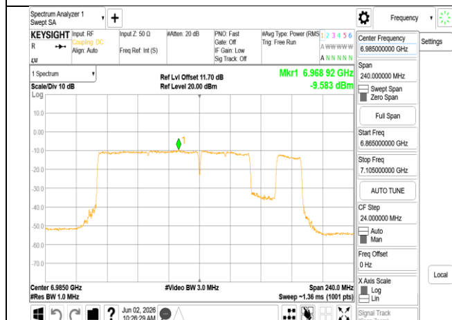
802.11be_160MHz_Chain0_6985MHz_996+484+242_MRU
