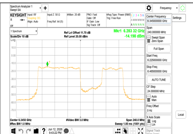
802.11be_160MHz_Chain1_6345MHz_996+484_MRU3
