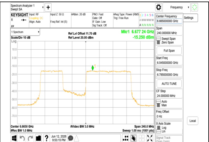
802.11be_160MHz_Chain1_6665MHz_996+484_MRU2
