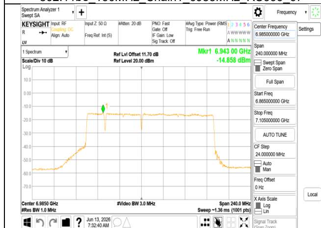
802.11be_160MHz_Chain1_6985MHz_996+484+242_MRU
