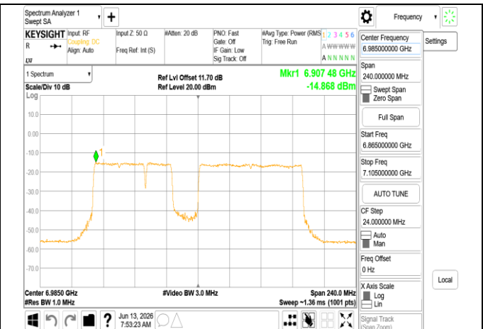
802.11be_160MHz_Chain1_6985MHz_996+484+242_MRU
