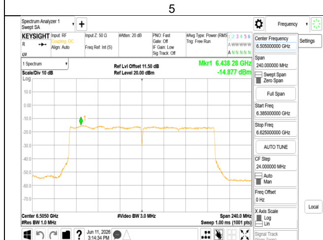
802.11be_160MHz_Chain1_6505MHz
