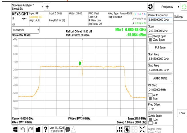
802.11be_160MHz_Chain1_6665MHz
