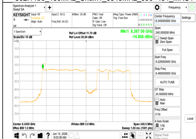
802.11be_160MHz_Chain1_6345MHz_996+484+242_MRU
