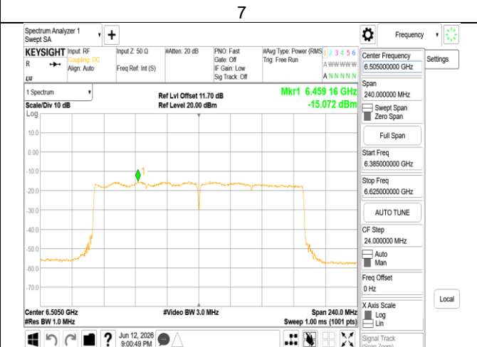
802.11be_160MHz_Chain1_6505MHz_RU996x2
