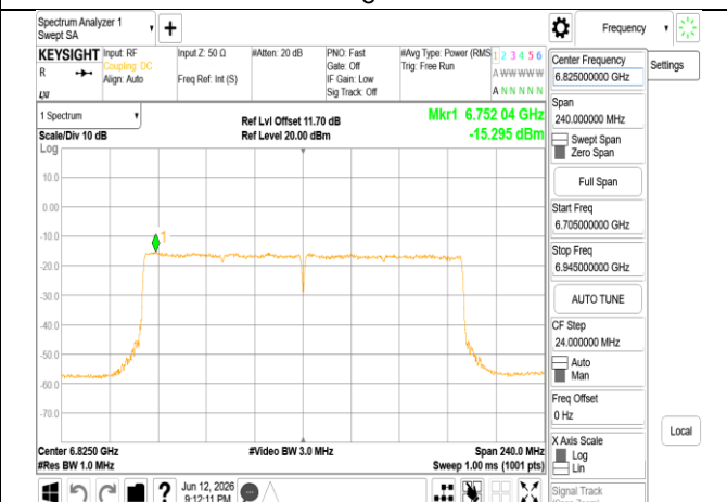
802.11be_160MHz_Chain1_6825MHz_RU996x2
