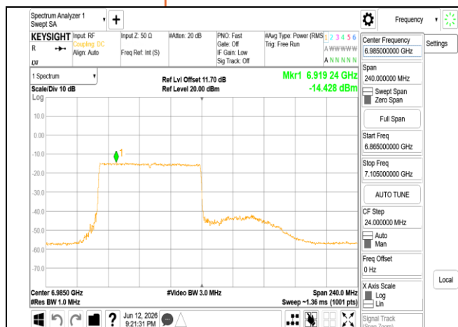
802.11be_160MHz_Chain1_6985MHz_RU996_67
