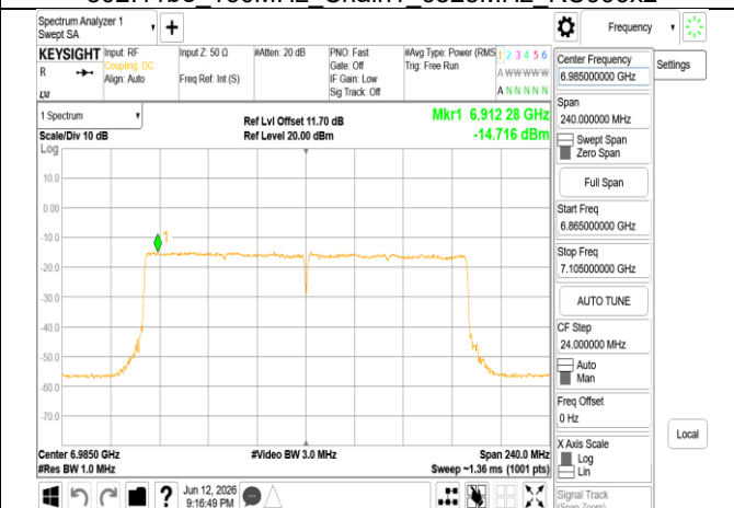
802.11be_160MHz_Chain1_6985MHz_RU996x2
