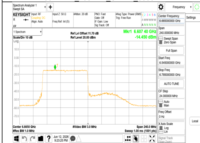
802.11be_160MHz_Chain1_6665MHz_RU996_67
