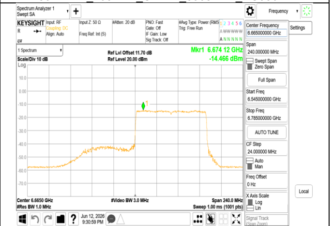
802.11be_160MHz_Chain1_6665MHz_RU996_S67
