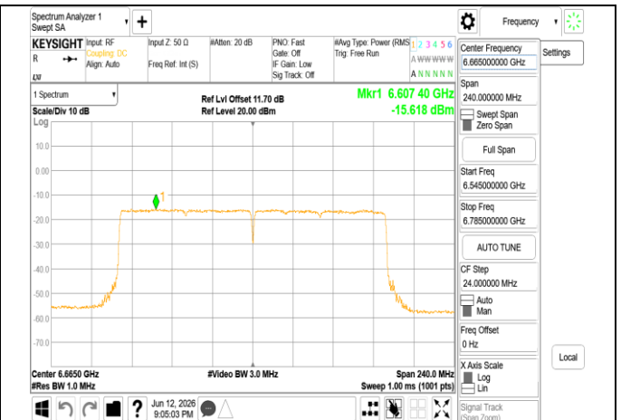
802.11be_160MHz_Chain1_6665MHz_RU996x2
