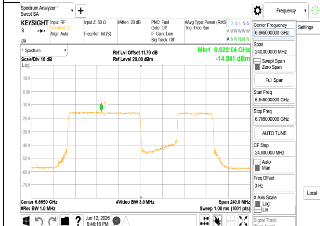
802.11be_160MHz_Chain1_6665MHz_996+484_MRU3
