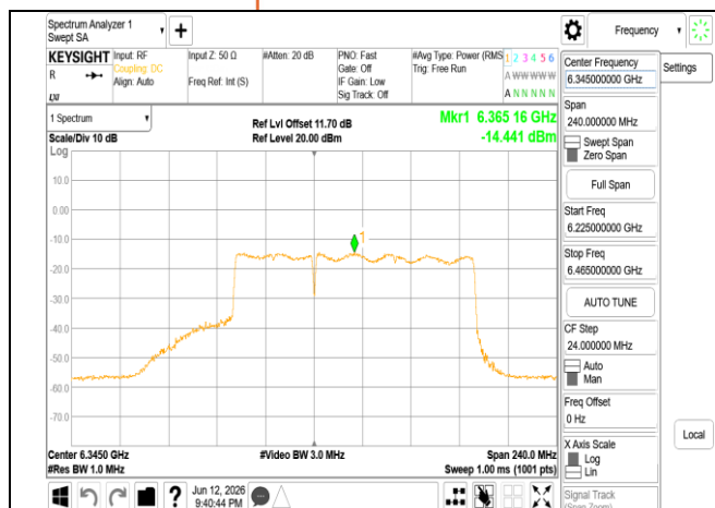
802.11be_160MHz_Chain1_6345MHz_996+484_MRU1
