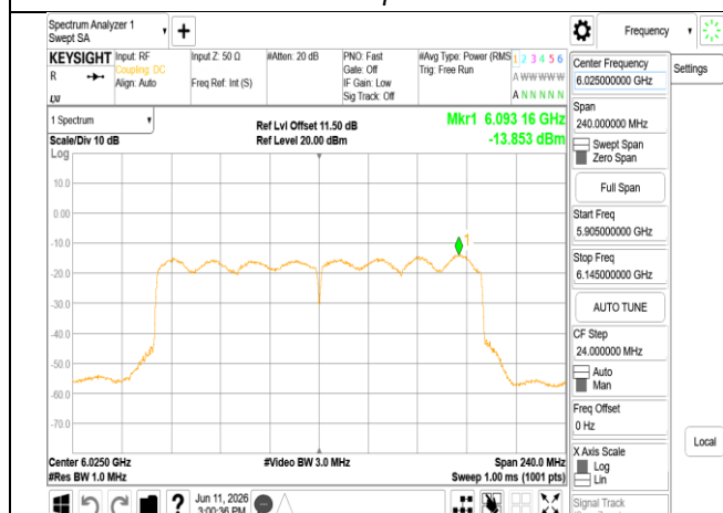
802.11be_160MHz_Chain1_6025MHz
