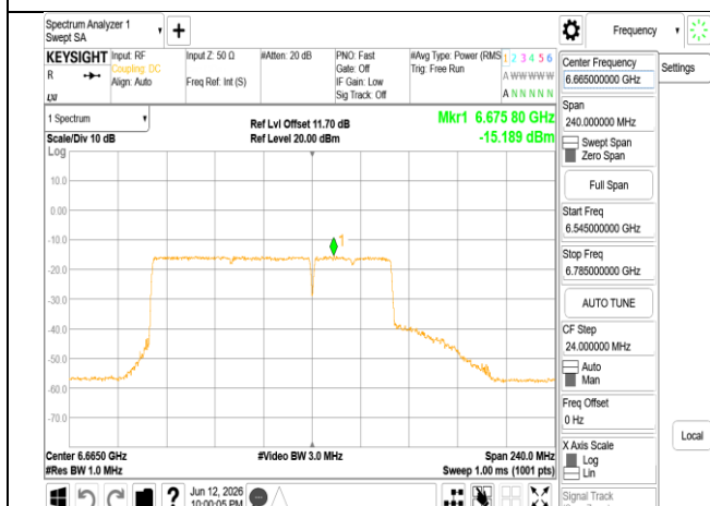
802.11be_160MHz_Chain1_6665MHz_996+484_MRU4
