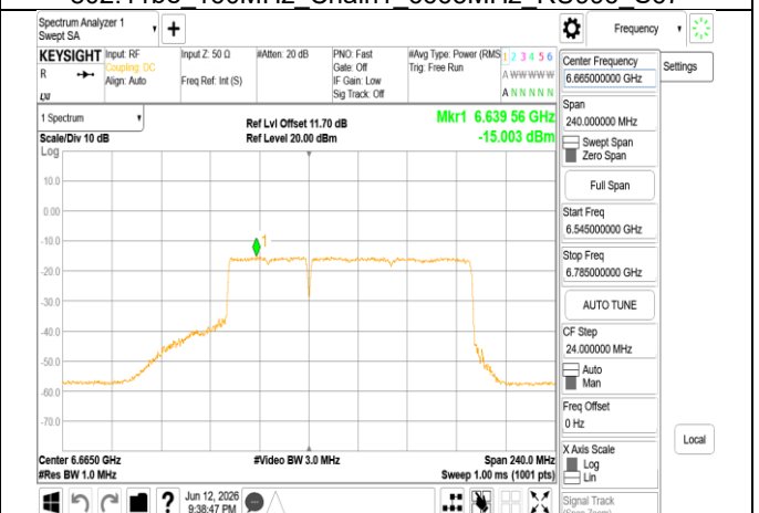
802.11be_160MHz_Chain1_6665MHz_996+484_MRU1
