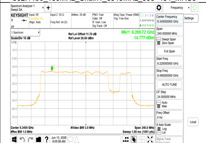
802.11be_160MHz_Chain1_6345MHz_996+484+242_MRU
