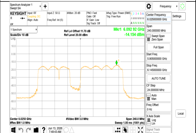
802.11be_160MHz_Chain1_6025MHz_996+484+242_MRU
