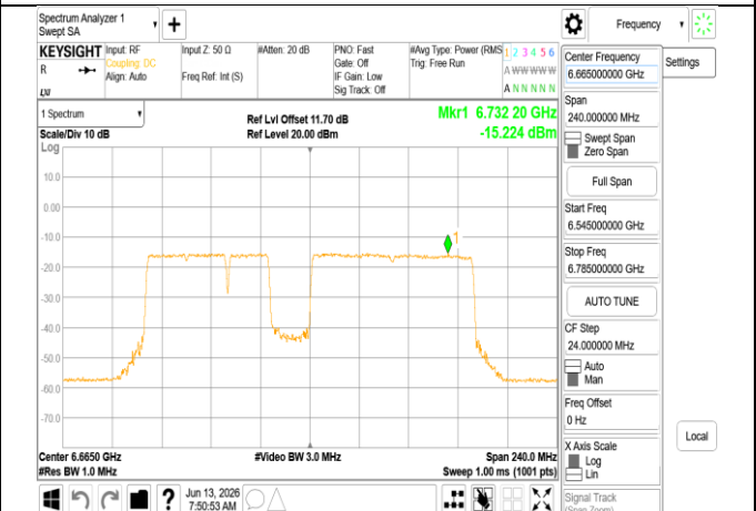
802.11be_160MHz_Chain1_6665MHz_996+484+242_MRU
