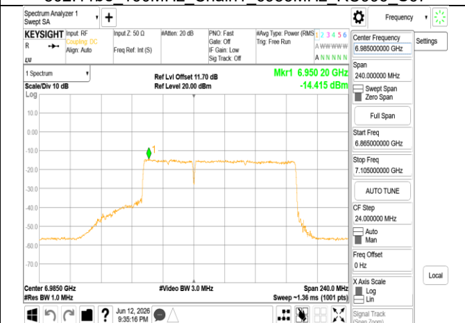
802.11be_160MHz_Chain1_6985MHz_996+484_MRU1
