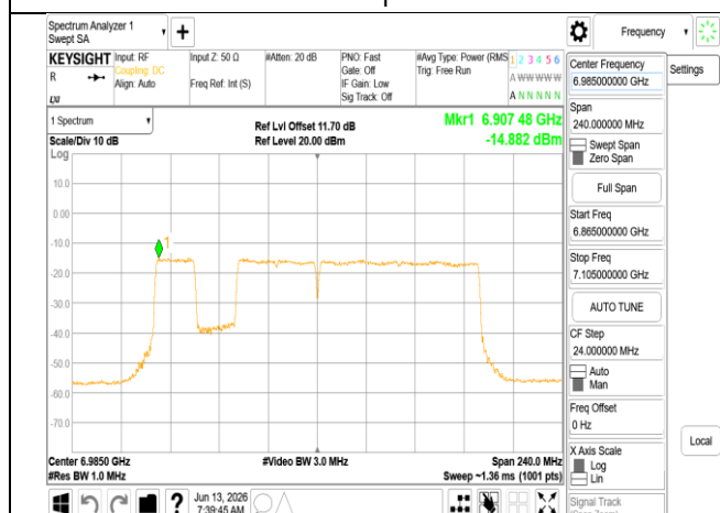
802.11be_160MHz_Chain1_6985MHz_996+484+242_MRU
