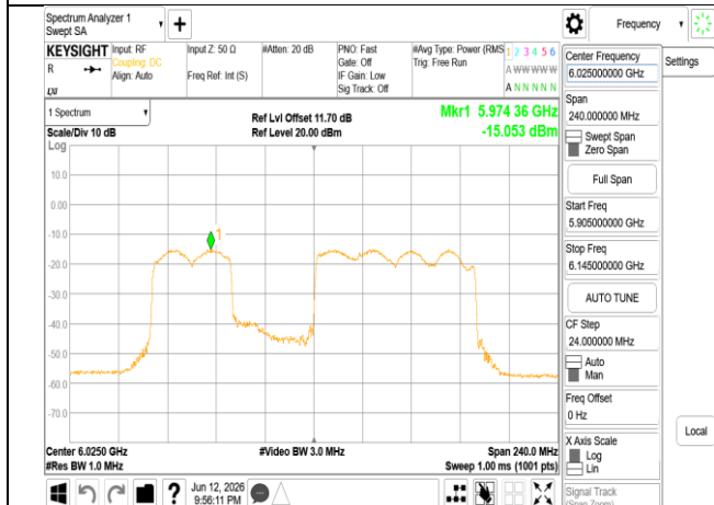
802.11be_160MHz_Chain1_6025MHz_996+484_MRU2
