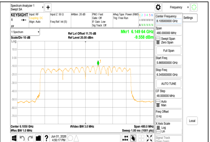
802.11be 320MHz Chain1 6105MHz RU996x4
