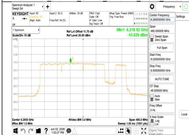
802.11be 320MHz Chain0 6265MHz 3x996+484 MRU7
