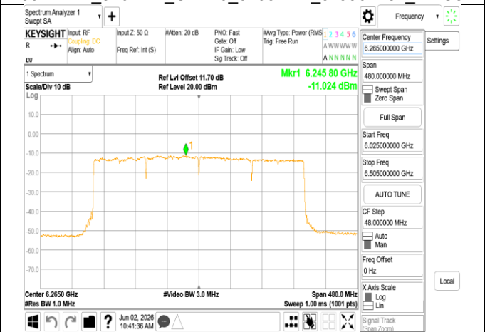
802.11be 320MHz Chain0 6265MHz RU996x4
