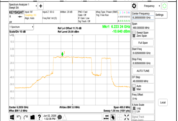
802.11be 320MHz Chain0 6265MHz 2x996+484 MRU11
