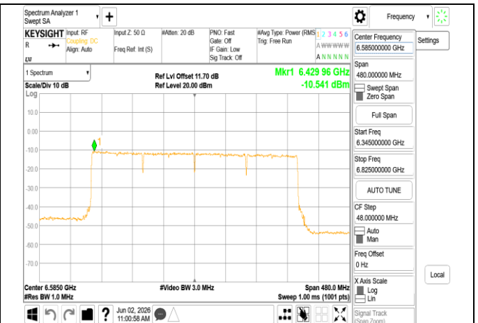
802.11be 320MHz Chain0 6585MHz RU996x4
