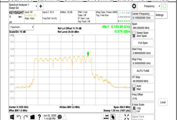
802.11be 320MHz Chain1 6105MHz 3x996 MRU4
