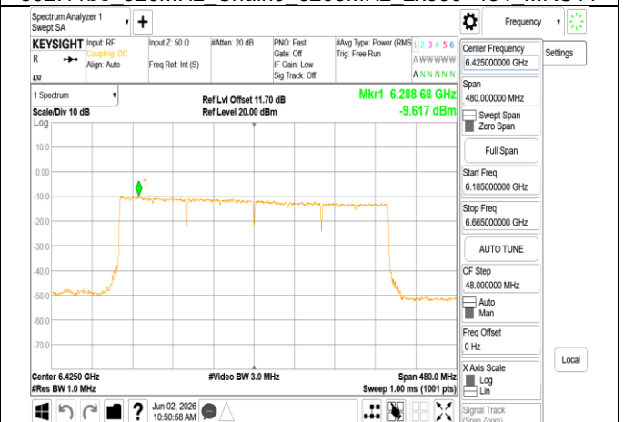
802.11be 320MHz Chain0 6425MHz RU996x4
