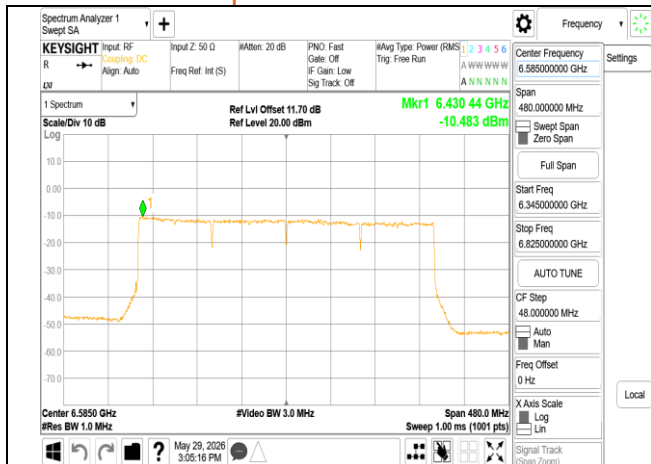
802.11be 320MHz Chain0 6585MHz
