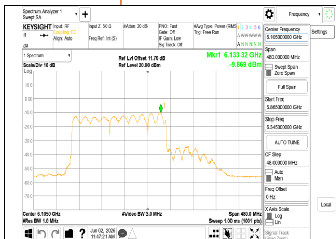
802.11be 320MHz Chain1 6105MHz 2x996+484 MRU6
