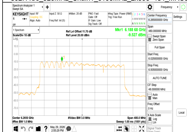
802.11be 320MHz Chain1 6265MHz
