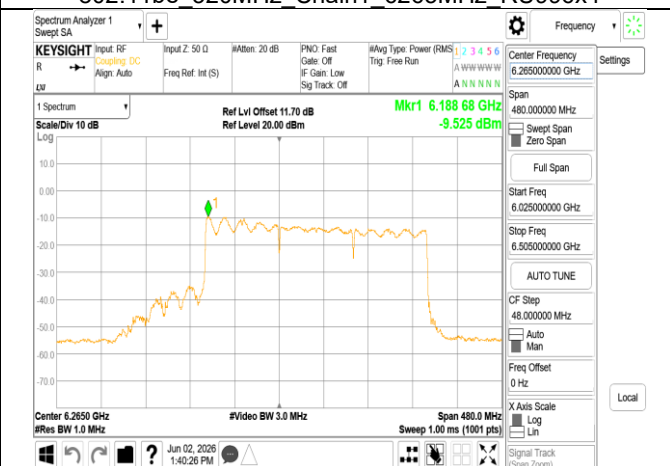
802.11be 320MHz Chain1 6265MHz 3x996 MRU1
