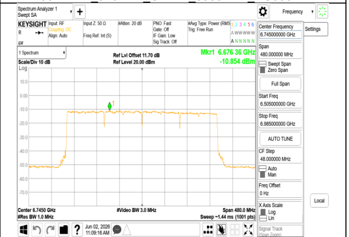
802.11be 320MHz Chain1 6745MHz RU996x4
