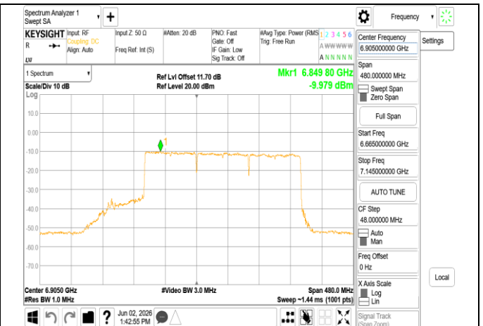
802.11be 320MHz Chain0 6905MHz 3x996 MRU1
