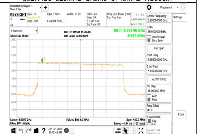
802.11be 320MHz Chain0 6905MHz RU996x4
