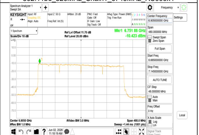
802.11be 320MHz Chain1 6905MHz RU996x4
