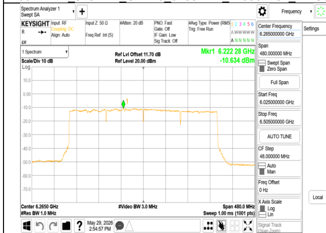
802.11be 320MHz Chain0 6265MHz
