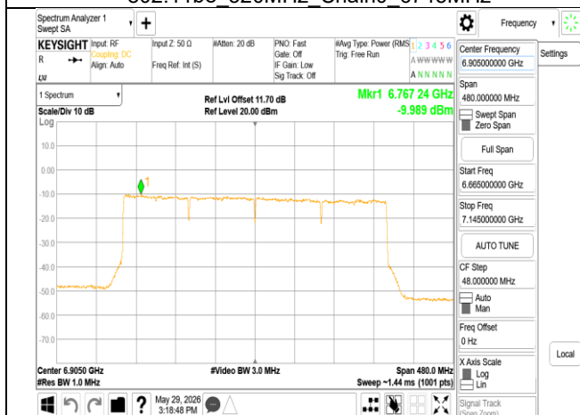
802.11be 320MHz Chain0 6905MHz
