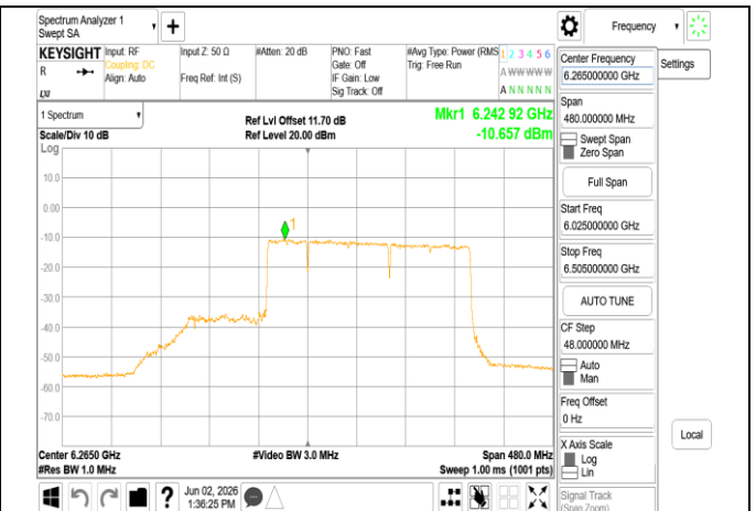
802.11be 320MHz Chain0 6265MHz 2x996+484 MRU7
