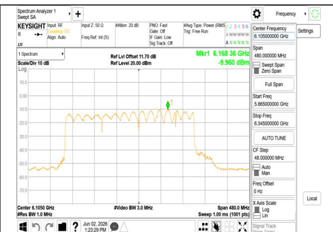
802.11be 320MHz Chain1 6105MHz 3x996+484 MRU8
