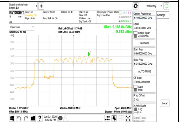
802.11be 320MHz Chain1 6105MHz 3x996+484 MRU2
