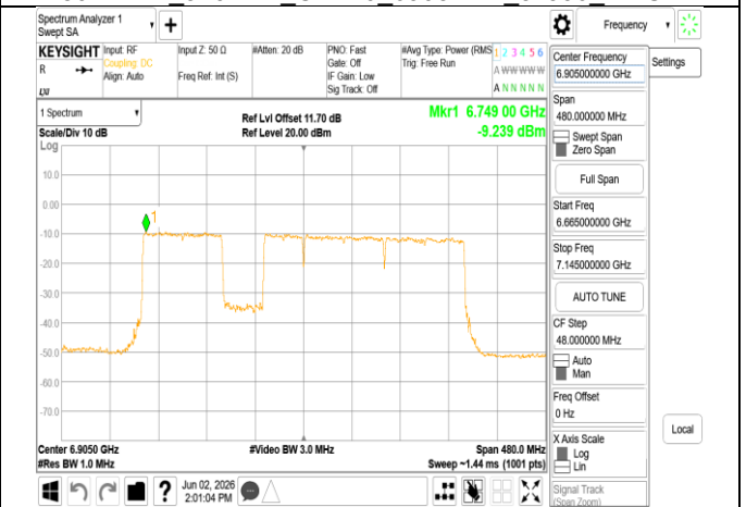
802.11be 320MHz Chain0 6905MHz 3x996+484 MRU3
