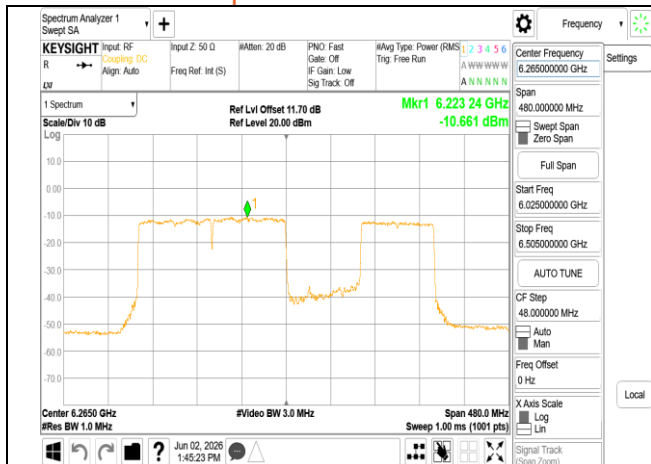
802.11be 320MHz Chain0 6265MHz 3x996 MRU3
