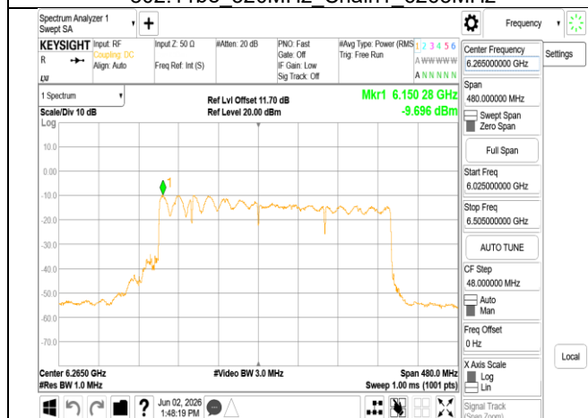
802.11be 320MHz Chain1 6265MHz 3x996+484 MRU1
