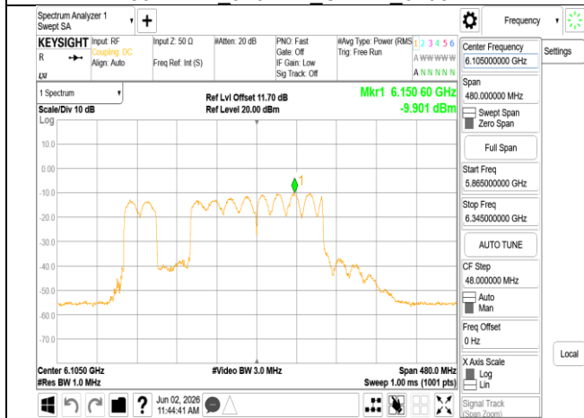
802.11be 320MHz Chain1 6105MHz 2x996+484 MRU2
