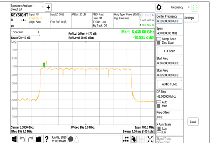
802.11be 320MHz Chain1 6585MHz RU996x4
