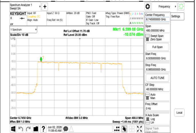
802.11be 320MHz Chain0 6745MHz RU996x4
