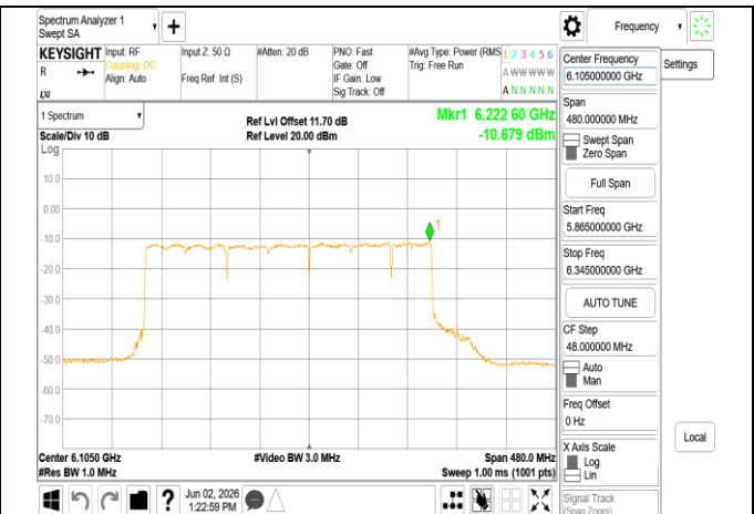
802.11be 320MHz Chain0 6105MHz 3x996+484 MRU8
