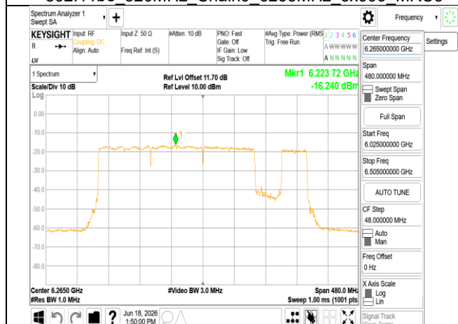
802.11be 320MHz Chain0 6265MHz 3x996+484 MRU7
