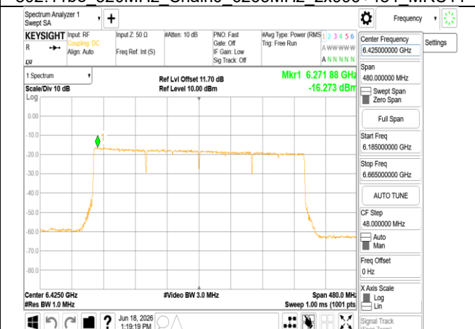
802.11be 320MHz Chain0 6425MHz RU996x4
