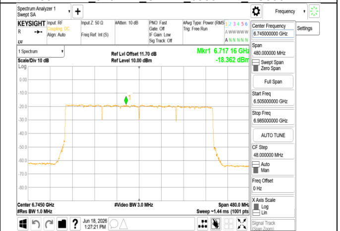
802.11be 320MHz_Chain1_6745MHz_RU996x4
