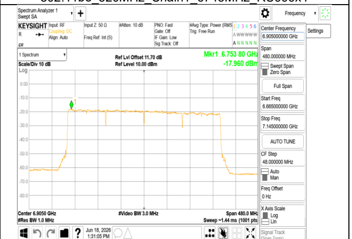
802.11be 320MHz_Chain1_6905MHz_RU996x4
