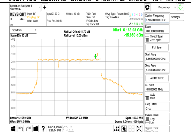
802.11be 320MHz Chain0 6105MHz 3x996 MRU4
