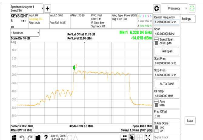
802.11be 320MHz Chain1 6265MHz 2x996+484 MRU7
