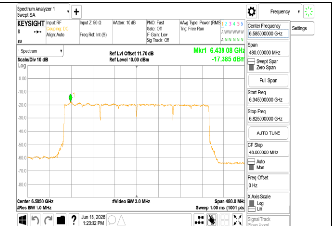
802.11be 320MHz_Chain1_6585MHz_RU996x4
