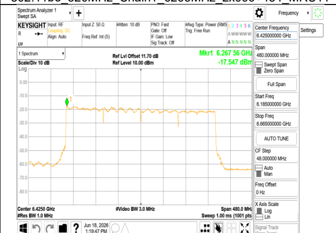
802.11be 320MHz Chain1 6425MHz RU996x4
