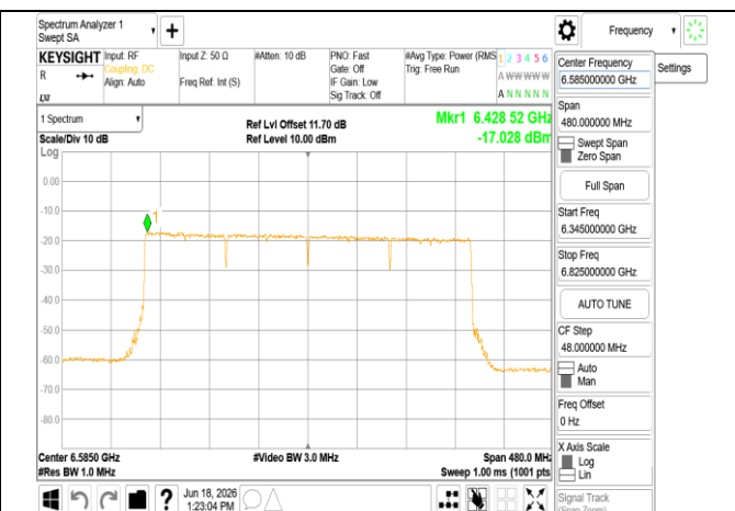
802.11be 320MHz Chain0 6585MHz RU996x4
