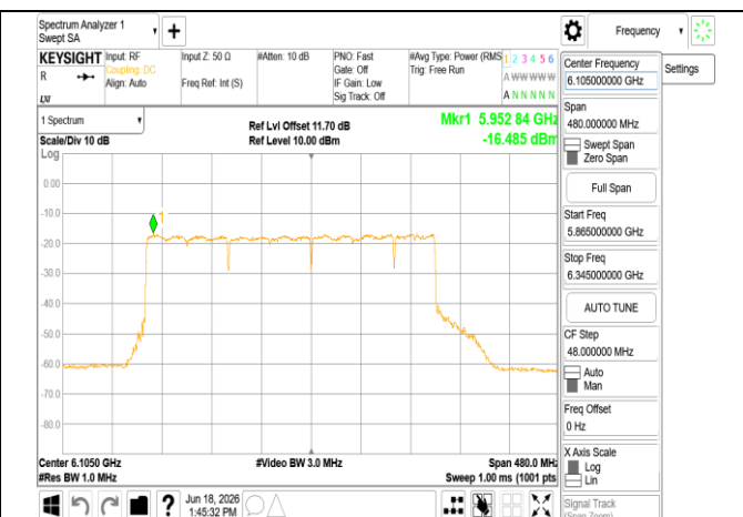
802.11be 320MHz Chain0 6105MHz 3x996+484 MRU8
