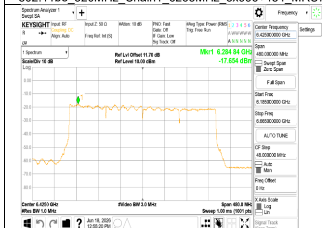
802.11be 320MHz Chain1 6425MHz
