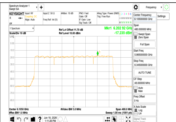
802.11be 320MHz Chain0 6105MHz RU996x4
