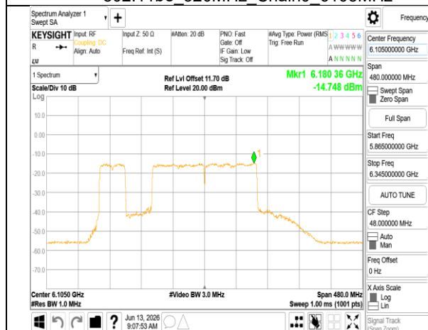
802.11be 320MHz Chain0 6105MHz 2x996+484 MRU2
