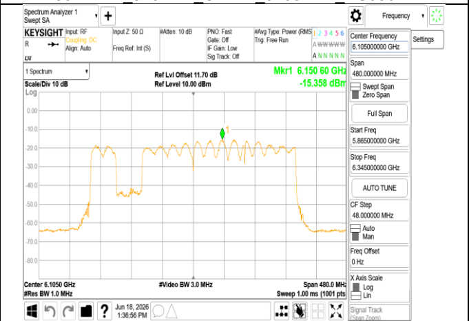
802.11be 320MHz Chain1 6105MHz 3x996+484 MRU2
