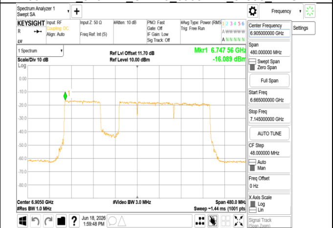
802.11be 320MHz Chain0 6905MHz 3x996+484 MRU3
