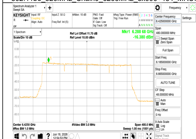
802.11be 320MHz Chain0 6425MHz
