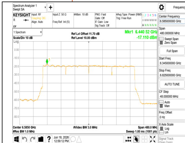
802.11be 320MHz_Chain1_6585MHz
