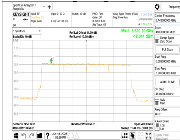
802.11be 320MHz_Chain1_6745MHz
