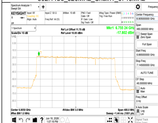
802.11be 320MHz_Chain1_6905MHz
