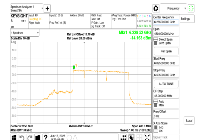
802.11be 320MHz Chain0 6265MHz 2x996+484 MRU7
