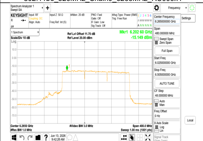
802.11be 320MHz Chain0 6265MHz 3x996 MRU1
