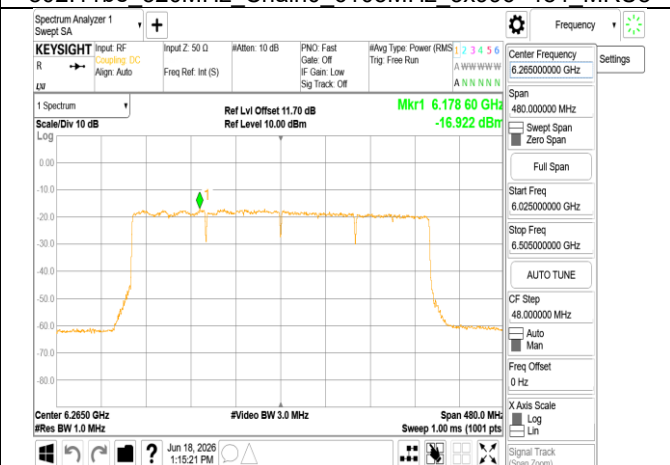
802.11be 320MHz Chain0 6265MHz RU996x4
