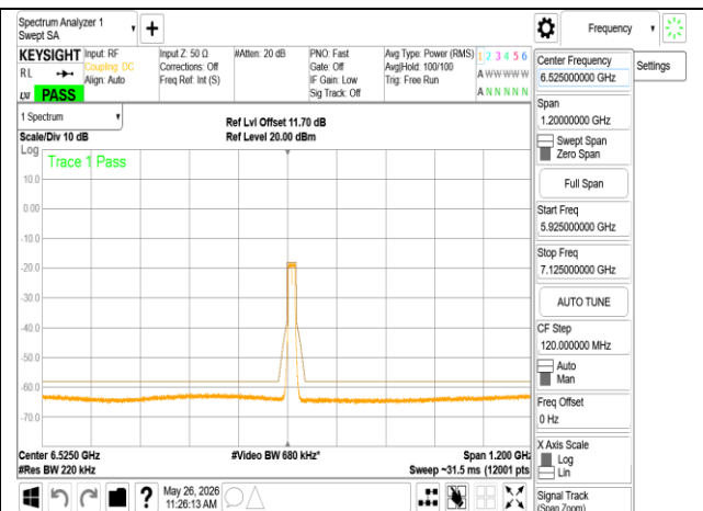
802.11a_20MHz_Chain1_6535MHz
