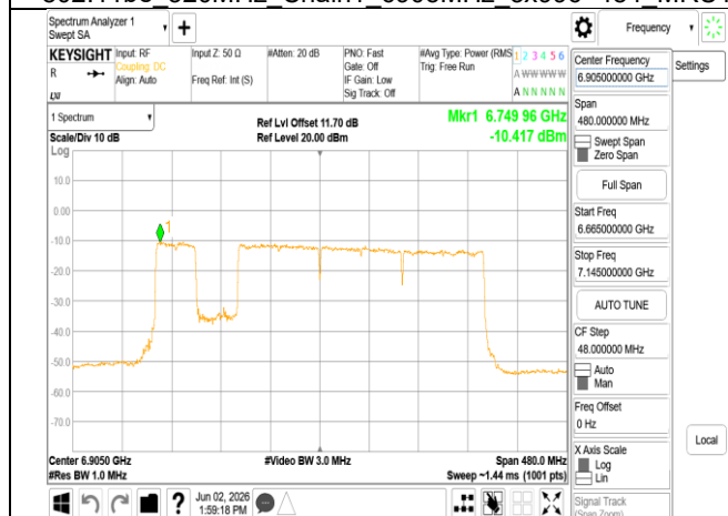
802.11be 320MHz Chain1 6905MHz 3x996+484 MRU2
