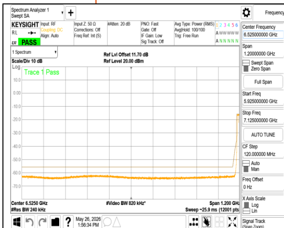
802.11a 20MHz Chain0 7115MHz
