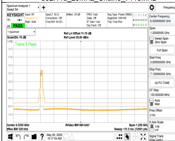
802.11a 20MHz Chain1 6175MHz
