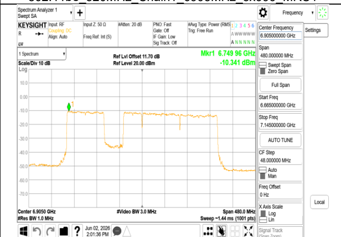
802.11be 320MHz Chain1 6905MHz 3x996+484 MRU3
