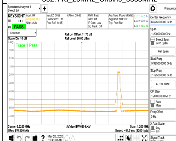
802.11a_20MHz_Chain0_6855MHz
