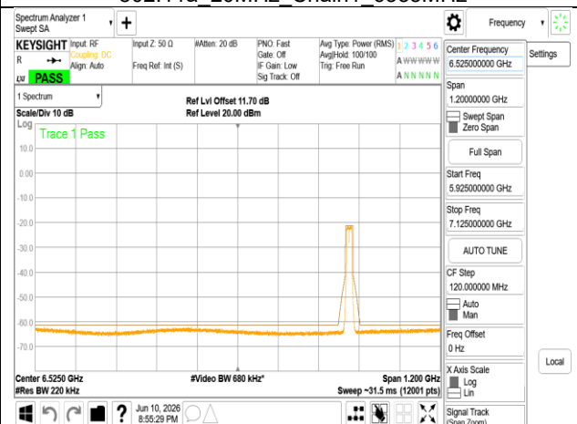
802.11a_20MHz_Chain1_6855MHz
