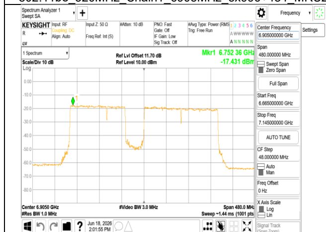
802.11be 320MHz Chain1 6905MHz 3x996+484 MRU4
