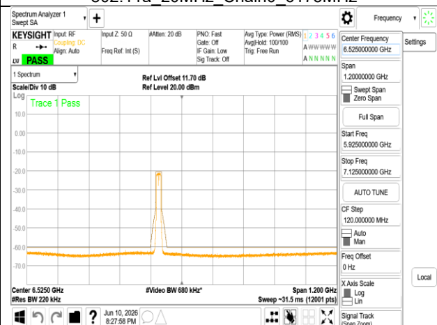
802.11a_20MHz_Chain0_6435MHz
