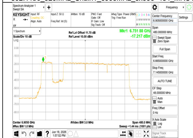
802.11be 320MHz Chain1 6905MHz 3x996+484 MRU2
