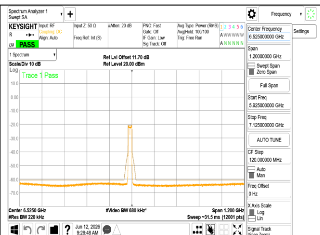
802.11ax_20MHz_Chain0_6515MHz RU242
