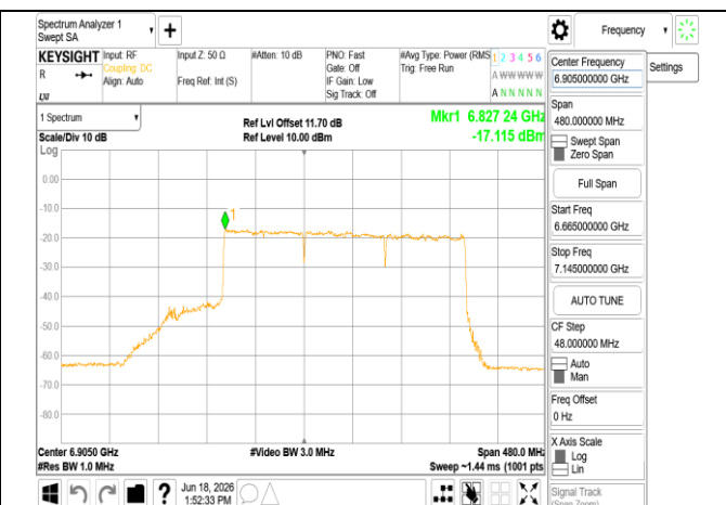
802.11be 320MHz Chain1 6905MHz 3x996 MRU1
