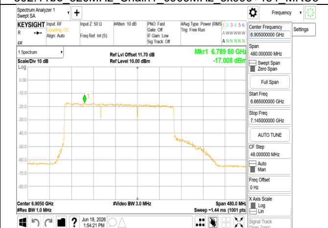
802.11be 320MHz Chain1 6905MHz 3x996 MRU4
