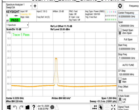
802.11ax_20MHz_Chain0_6435MHz
