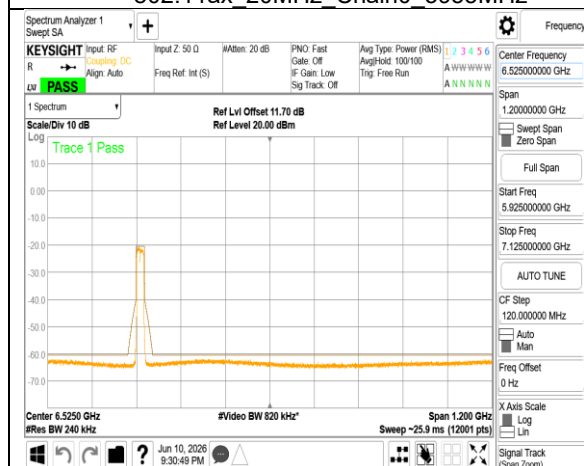
802.11ax_20MHz_Chain0_6175MHz
