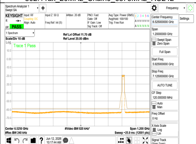
802.11ax_20MHz_Chain0_6895MHz RU242
