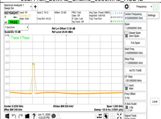
802.11ax_20MHz_Chain0_6175MHz RU242
