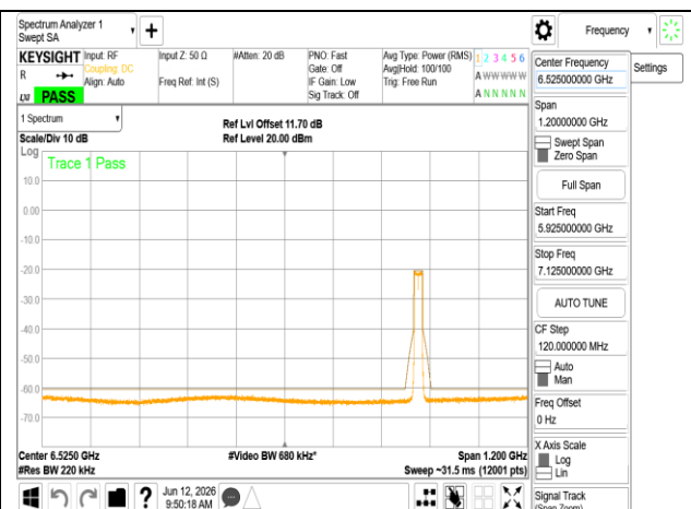
802.11ax_20MHz_Chain0_6855MHz RU242
