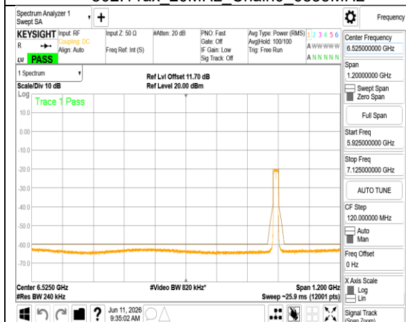
802.11ax_20MHz_Chain0_6875MHz
