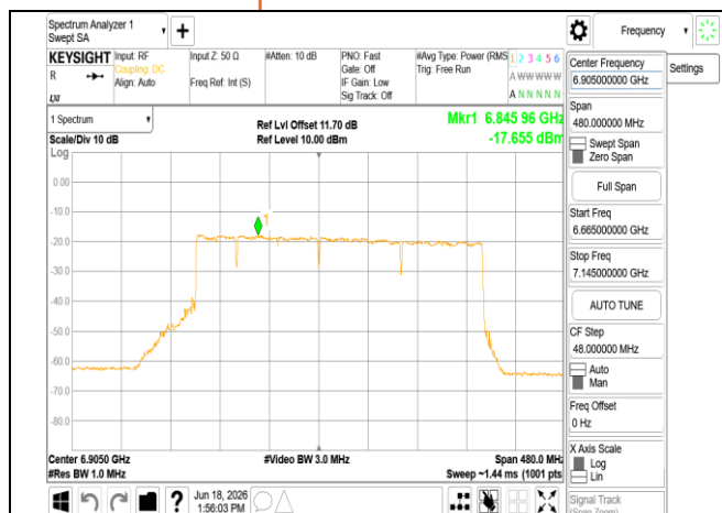
802.11be 320MHz Chain1 6905MHz 3x996+484 MRU1
