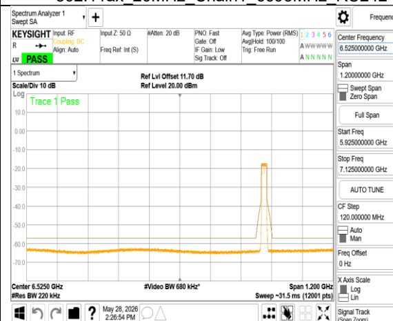
802.11ax_20MHz_Chain1_6855MHz RU242
