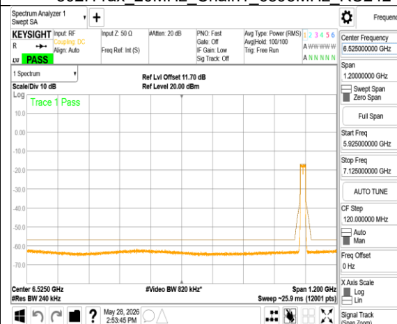
802.11ax_20MHz_Chain1_6995MHz RU242
