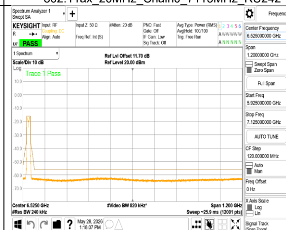
802.11ax_20MHz_Chain1_5955MHz RU242
