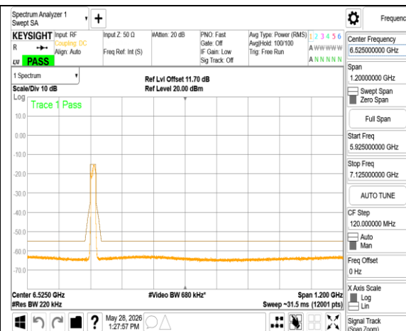
802.11ax_20MHz_Chain1_6175MHz RU242
