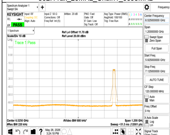
802.11ax_20MHz_Chain1_6855MHz
