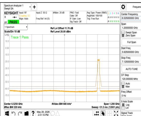
802.11ax_20MHz_Chain1_6895MHz RU242
