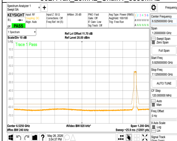
802.11ax_20MHz_Chain1_6995MHz
