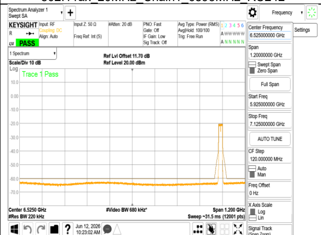
802.11ax_20MHz_Chain1_6995MHz RU242
