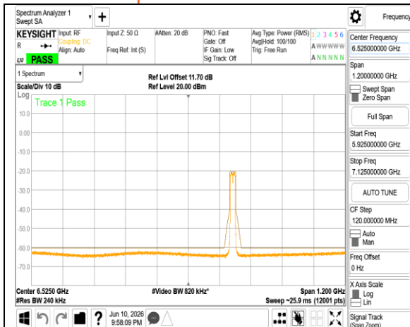
802.11ax_20MHz_Chain1_6695MHz
