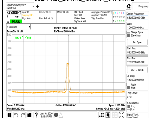
802.11ax_20MHz_Chain1_6515MHz
