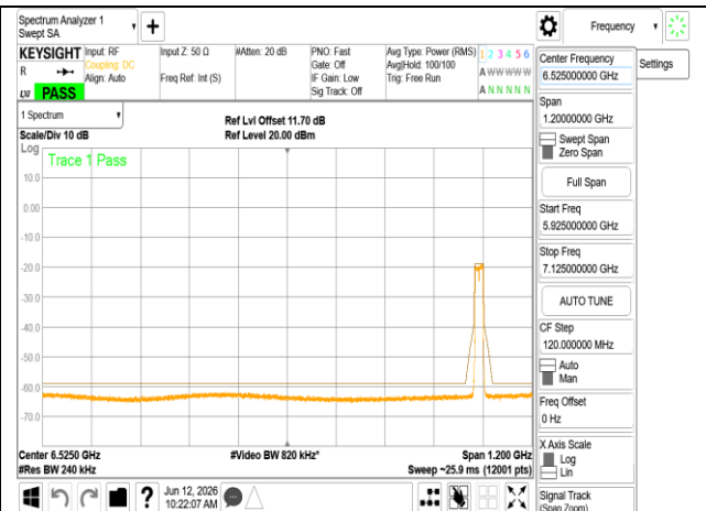
802.11ax_20MHz_Chain0_6995MHz RU242
