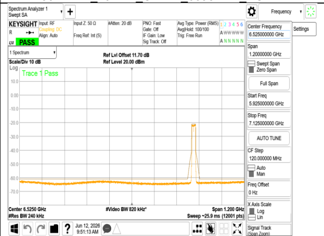
802.11ax_20MHz_Chain1_6855MHz RU242
