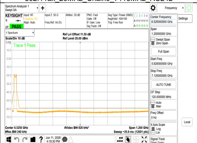
802.11ax_20MHz_Chain1_5955MHz RU242
