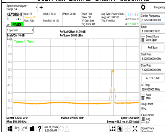
802.11ax_20MHz_Chain1_6875MHz
