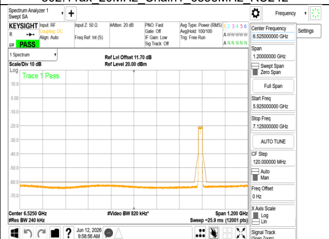
802.11ax_20MHz_Chain1_6875MHz RU242
