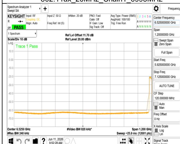
802.11ax_20MHz_Chain1_7115MHz
