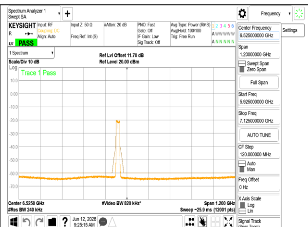
802.11ax_20MHz_Chain1_6475MHz RU242
