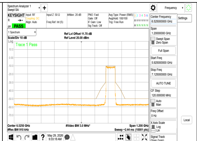
802.11ax_80MHz_Chain1_6785MHz RU996
