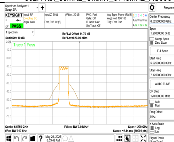
802.11ax_80MHz_Chain1_6385MHz RU996
