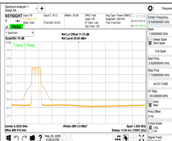
802.11ax_80MHz_Chain1_6145MHz RU996
