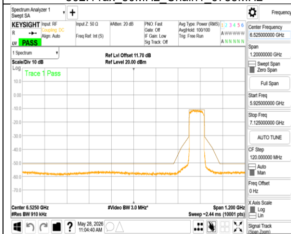
802.11ax_80MHz_Chain1_6865MHz
