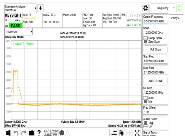
802.11be 40MHz Chain0 5965MHz RU484
