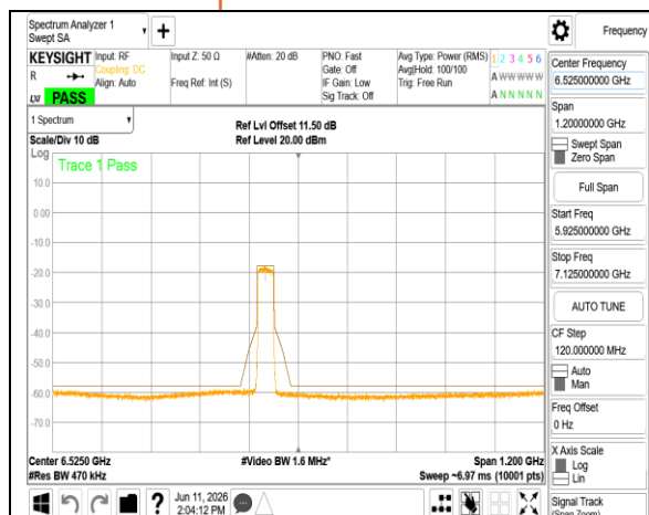
802.11be 40MHz Chain0 6445MHz
