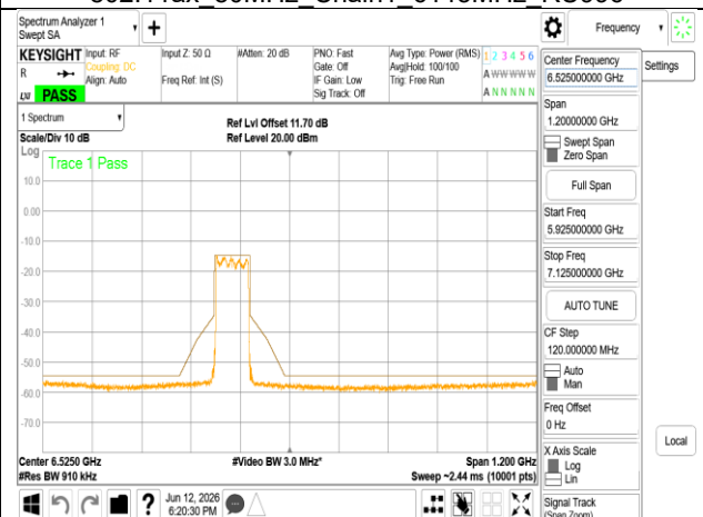
802.11ax_80MHz_Chain1_6385MHz RU996
