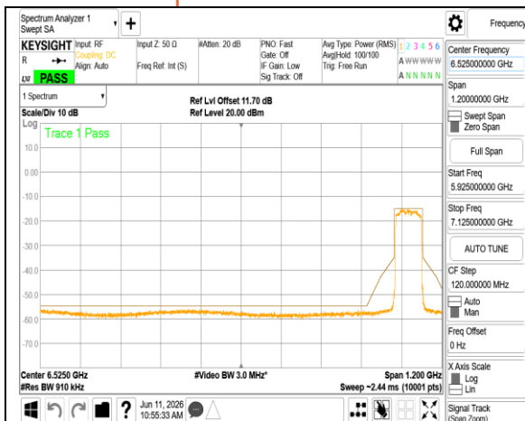
802.11ax_80MHz_Chain1_7025MHz
