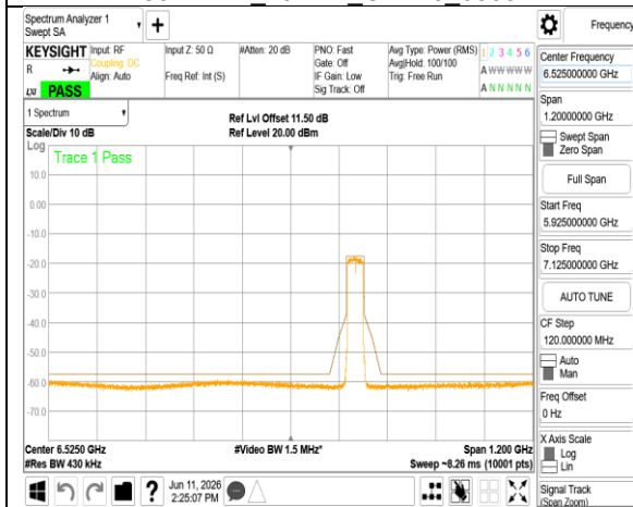
802.11be 40MHz Chain0 6685MHz
