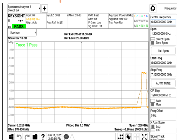
802.11be 40MHz Chain0 7085MHz
