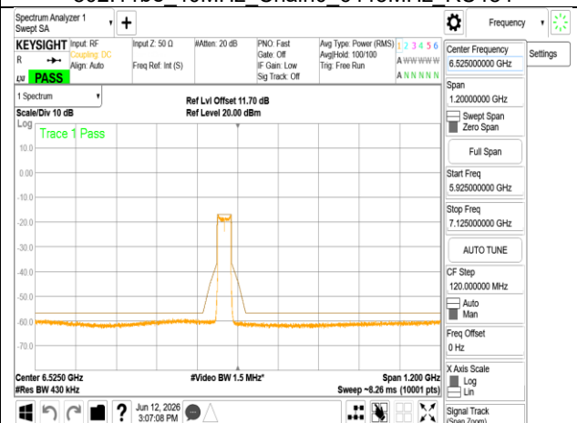
802.11be 40MHz Chain0 6485MHz RU484
