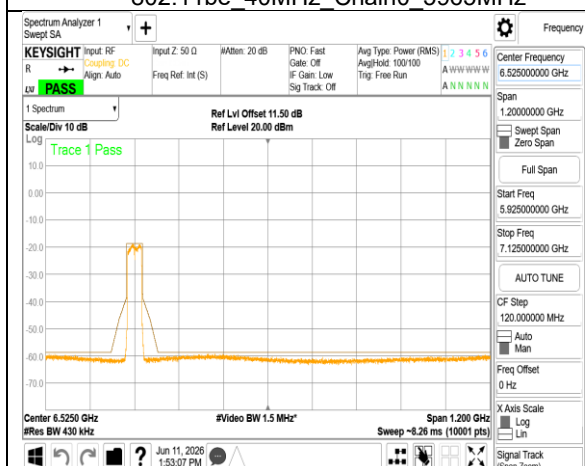
802.11be 40MHz Chain0 6165MHz
