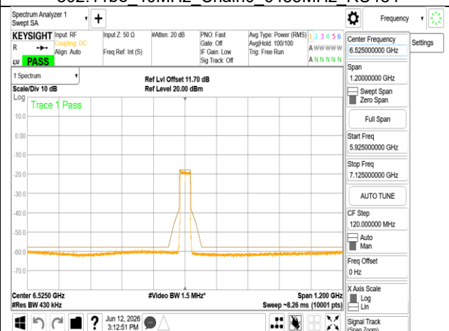
802.11be 40MHz Chain0 6525MHz RU484
