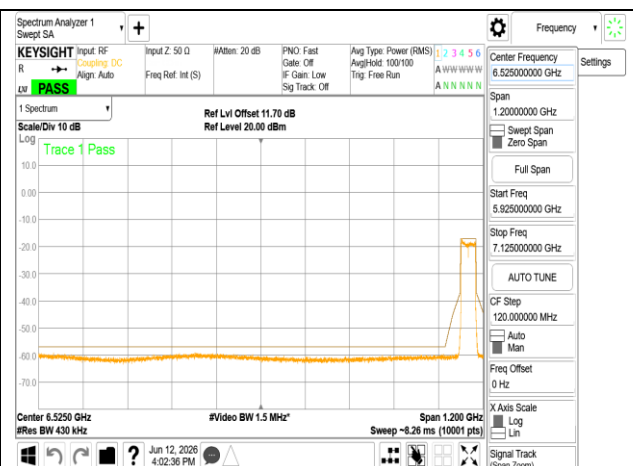
802.11be 40MHz Chain0 7085MHz RU484
