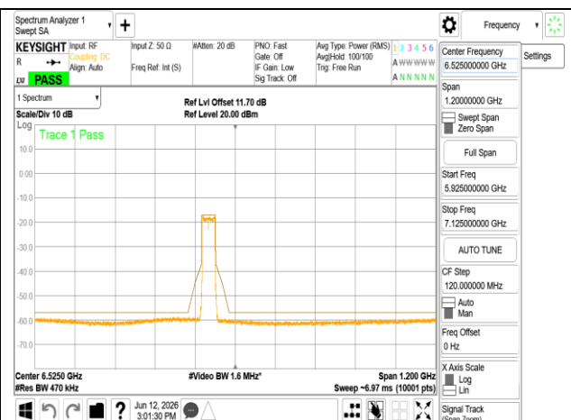
802.11be 40MHz Chain0 6445MHz RU484
