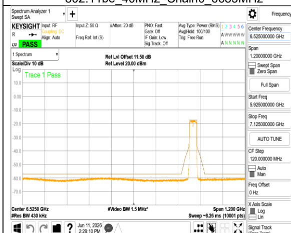
802.11be 40MHz Chain0 6845MHz
