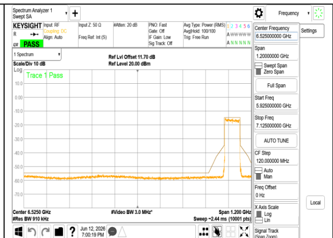
802.11ax_80MHz_Chain1_7025MHz RU996
