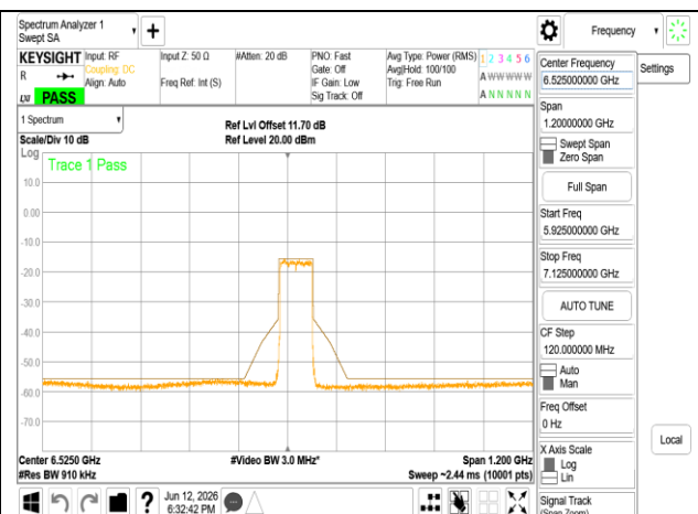
802.11ax 80MHz Chain1 6545MHz RU996
