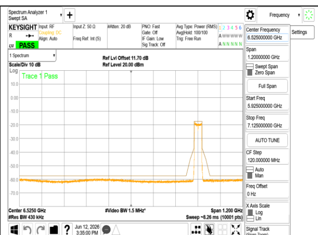
802.11be 40MHz Chain0 6885MHz RU484
