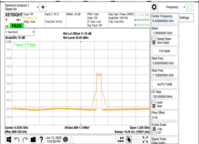
802.11be 40MHz Chain0 6685MHz RU484
