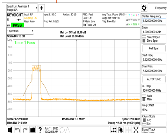
802.11ax_80MHz_Chain1_6145MHz
