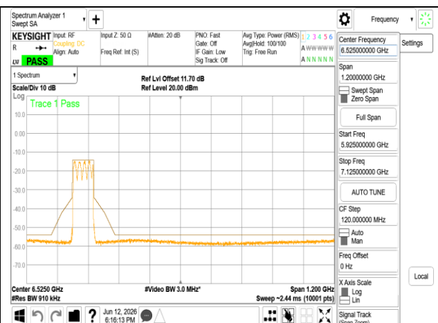
802.11ax_80MHz_Chain1_6145MHz RU996
