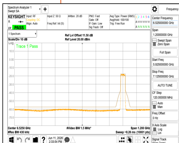
802.11be 40MHz Chain0 6885MHz
