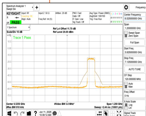
802.11ax_80MHz_Chain1_6785MHz
