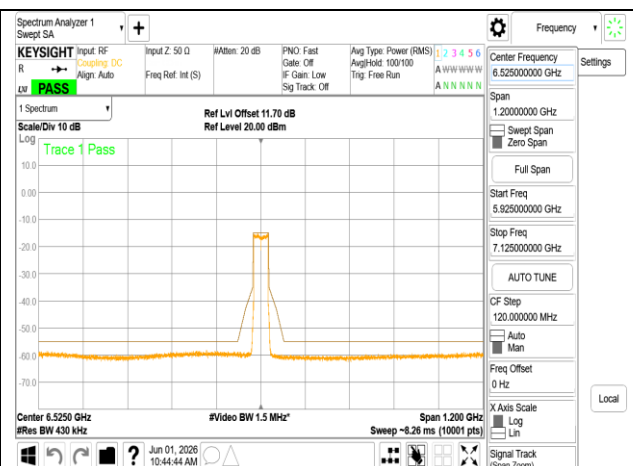
802.11be 40MHz Chain1 6525MHz RU484
