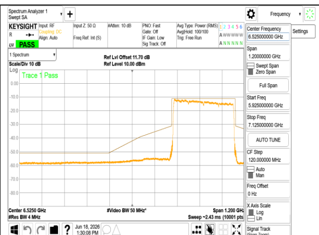
802.11be_320MHz_Chain1_6905MHz_RU996x4
