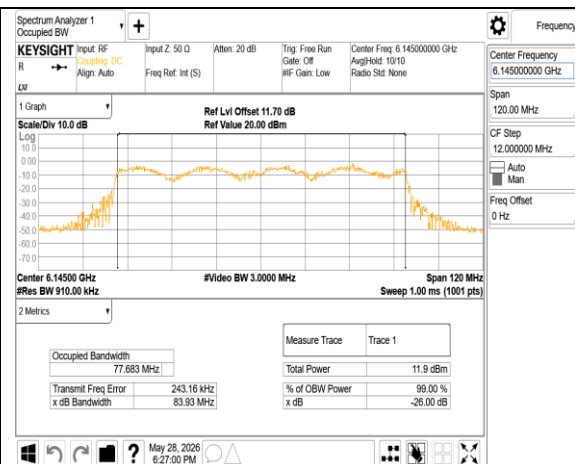
802.11ax_80MHz_Chain1_6145MHz RU996
