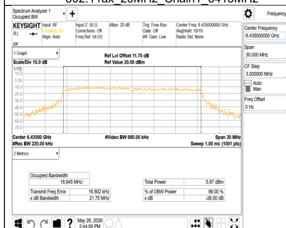
802.11ax_20MHz_Chain1_6435MHz
