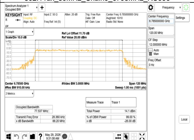
802.11ax 80MHz Chain0_6785MHz RU996
