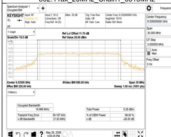
802.11ax_20MHz_Chain1_6535MHz
