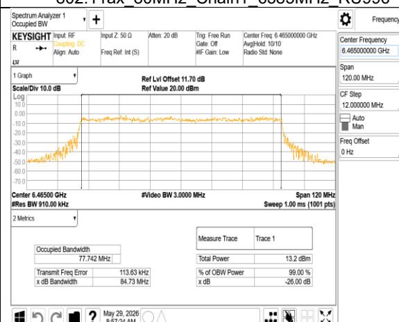
802.11ax_80MHz_Chain1_6465MHz RU996
