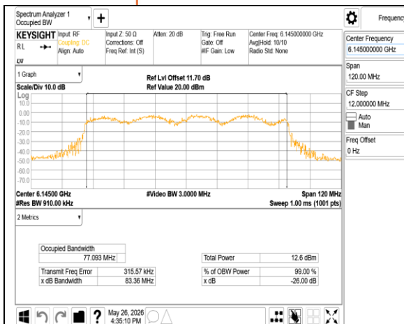
802.11ax_80MHz_Chain1_6145MHz
