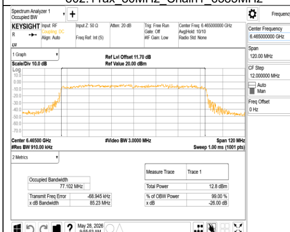
802.11ax_80MHz_Chain1_6465MHz
