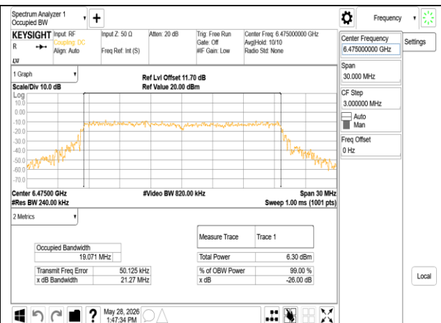
802.11ax_20MHz_Chain1_6475MHz RU242
