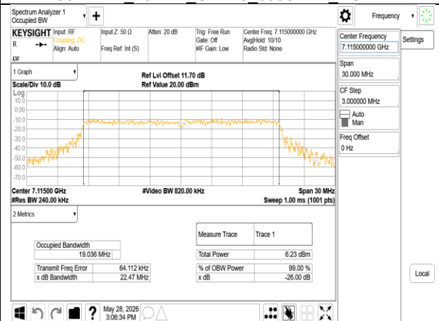
802.11ax 20MHz Chain0 7115MHz RU242
