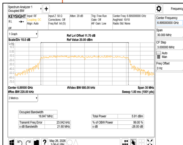
802.11ax_20MHz_Chain1_6895MHz
