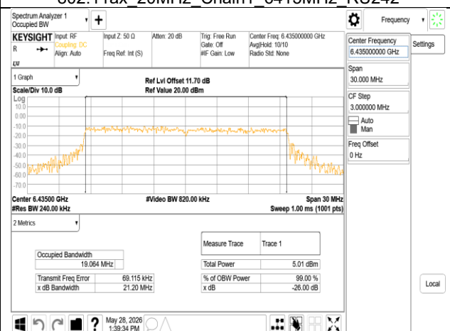
802.11ax_20MHz_Chain1_6435MHz RU242
