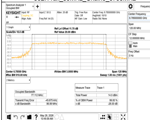
802.11ax 80MHz Chain0_6785MHz
