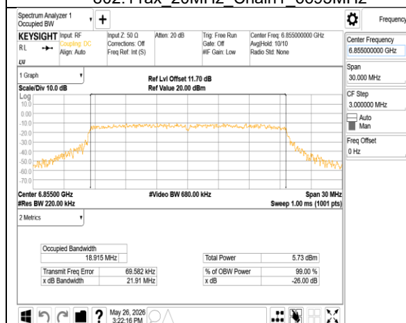
802.11ax 20MHz Chain1 6855MHz
