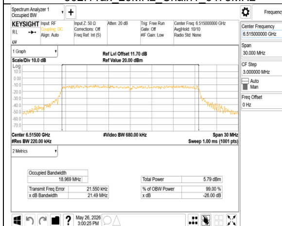
802.11ax_20MHz_Chain1_6515MHz
