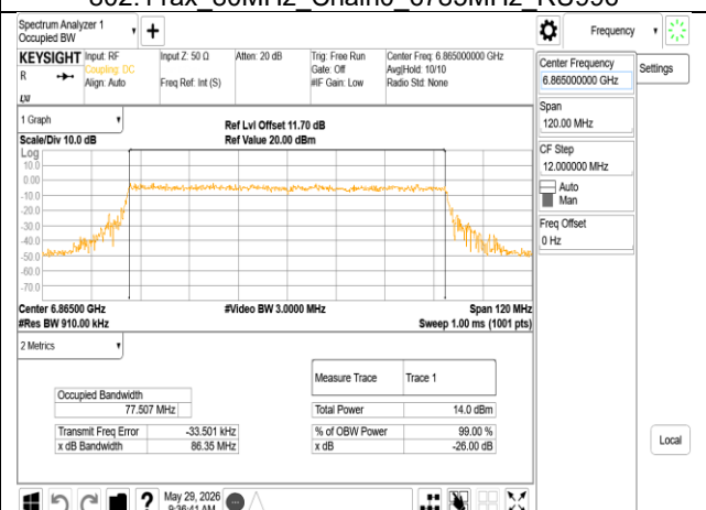
802.11ax 80MHz Chain0_6865MHz RU996
