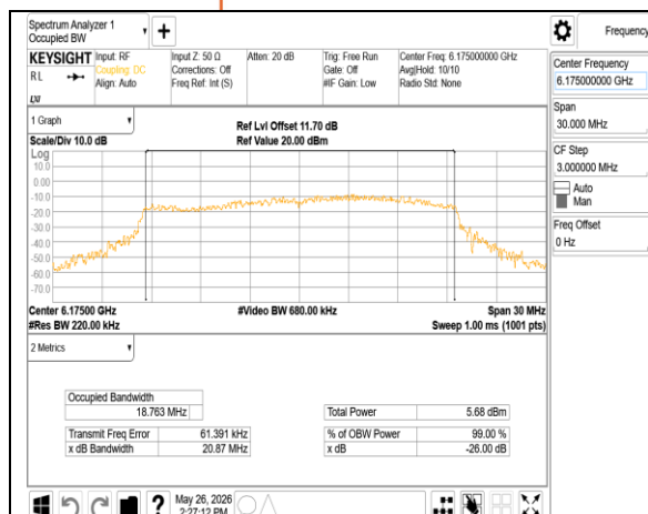
802.11ax_20MHz_Chain1_6175MHz
