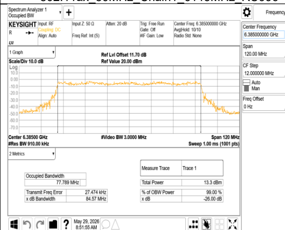
802.11ax_80MHz_Chain1_6385MHz RU996
