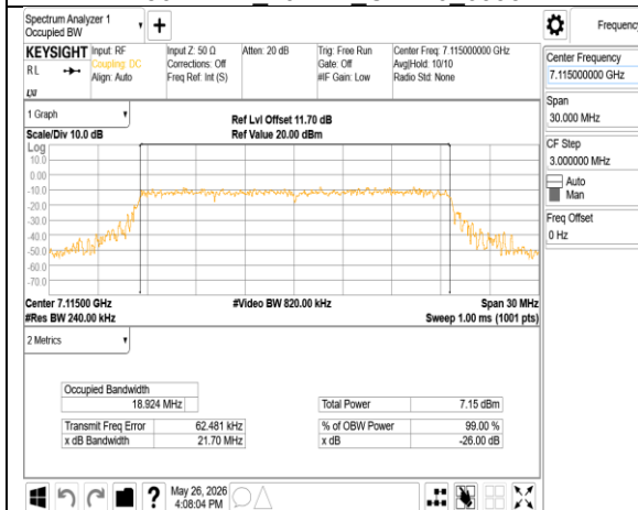
802.11ax 20MHz Chain0 7115MHz
