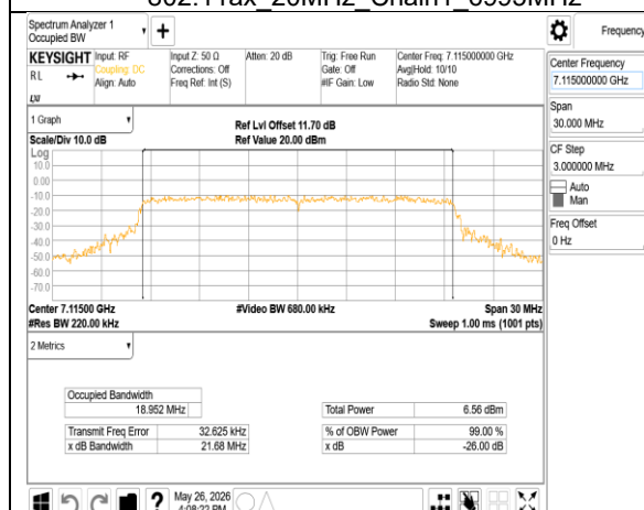
802.11ax_20MHz_Chain1_7115MHz
