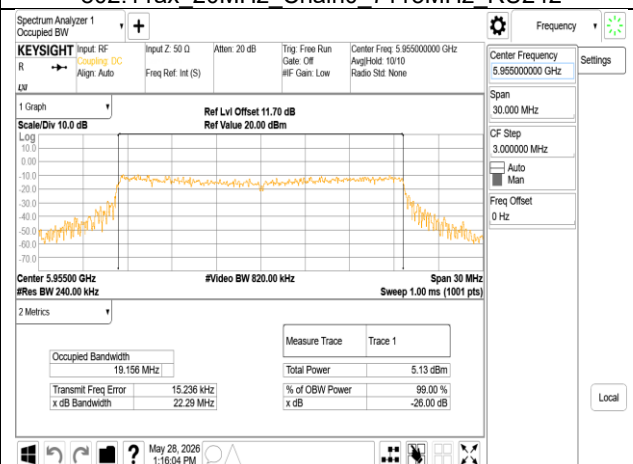
802.11ax 20MHz Chain1 5955MHz RU242
