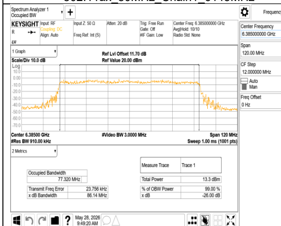
802.11ax_80MHz_Chain1_6385MHz
