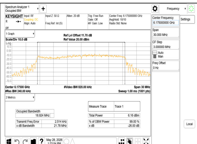
802.11ax_20MHz_Chain1_6175MHz RU242
