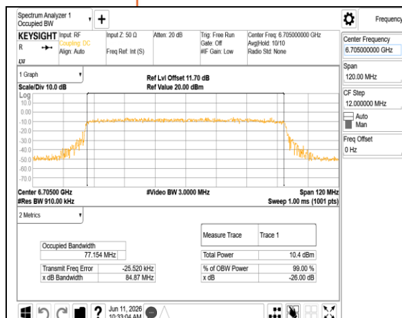
802.11ax_80MHz_Chain0_6705MHz
