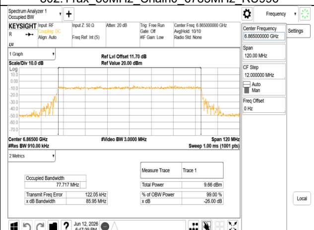
802.11ax_80MHz_Chain0_6865MHz RU996
