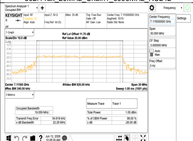
802.11ax_20MHz_Chain1_7115MHz RU242
