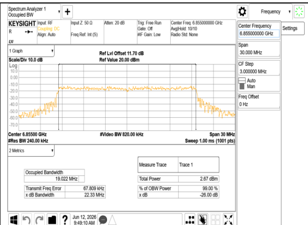
802.11ax_20MHz_Chain0_6855MHz RU242
