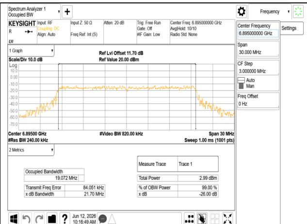
802.11ax_20MHz_Chain1_6895MHz RU242
