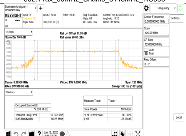
802.11ax_80MHz_Chain0_6385MHz RU996
