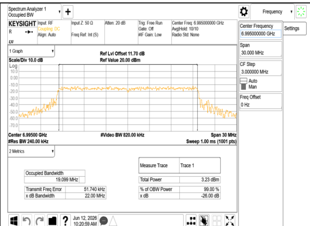
802.11ax_20MHz_Chain0_6995MHz RU242
