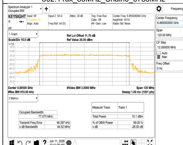
802.11ax_80MHz_Chain0_6865MHz
