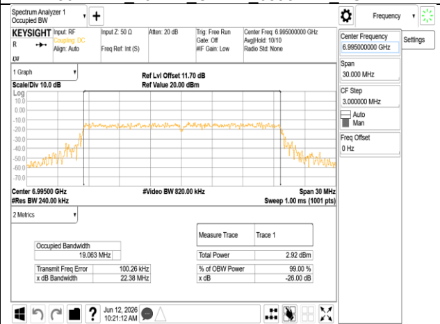
802.11ax_20MHz_Chain1_6995MHz RU242
