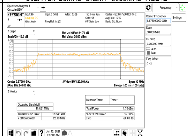
802.11ax 20MHz Chain1 6875MHz RU242
