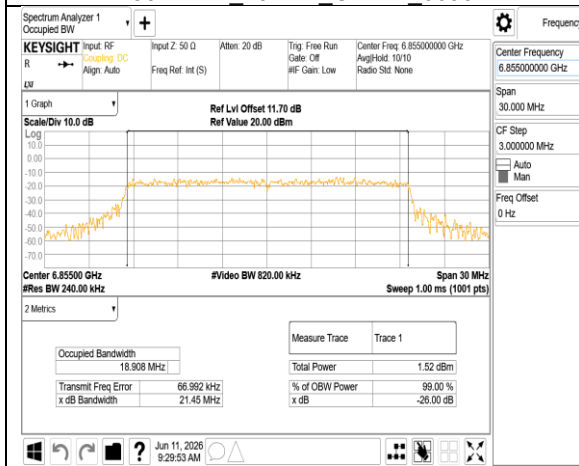
802.11ax 20MHz Chain1 6855MHz
