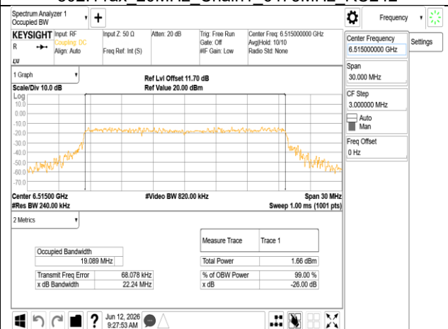
802.11ax 20MHz Chain1 6515MHz RU242
