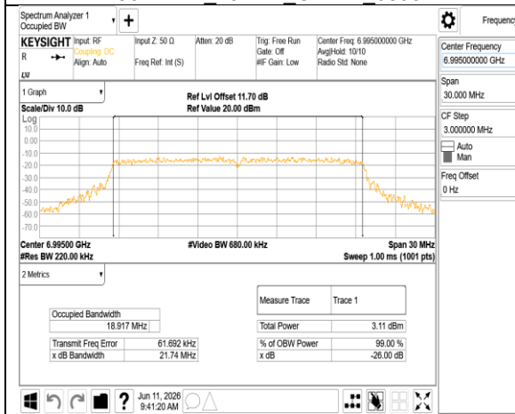
802.11ax_20MHz_Chain1_6995MHz
