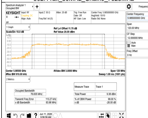
802.11ax 80MHz Chain1 5985MHz
