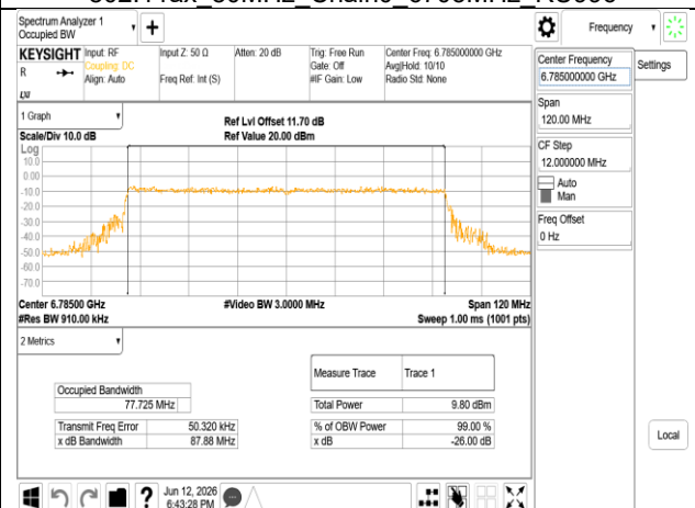
802.11ax_80MHz_Chain0_6785MHz RU996
