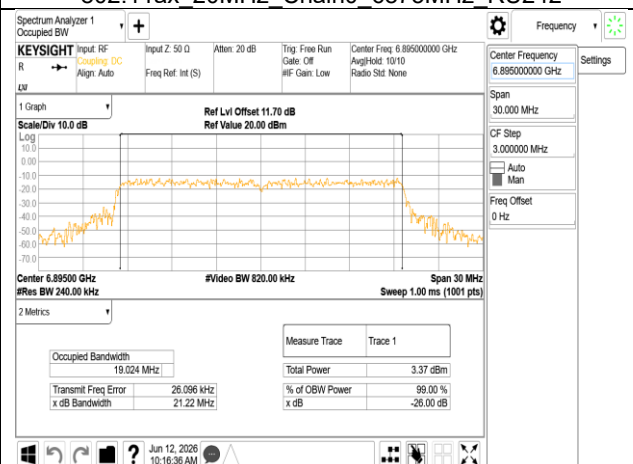
802.11ax_20MHz_Chain0_6895MHz RU242
