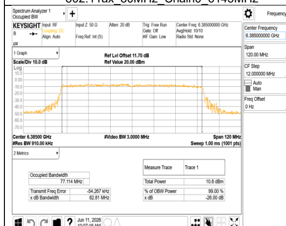
802.11ax_80MHz_Chain0_6385MHz
