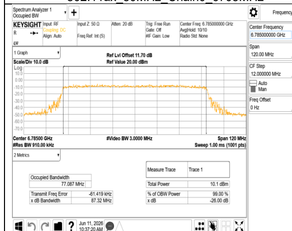
802.11ax_80MHz_Chain0_6785MHz
