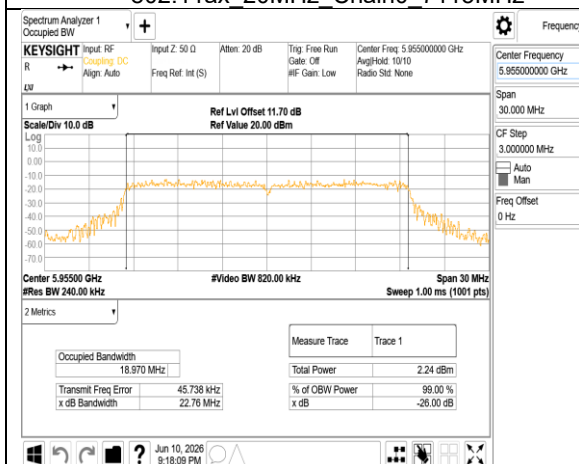
802.11ax_20MHz_Chain1_5955MHz
