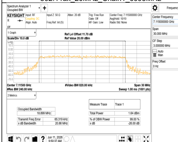
802.11ax_20MHz_Chain1_7115MHz
