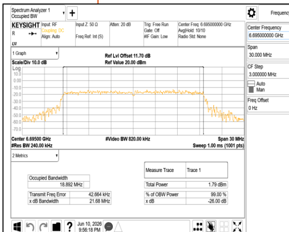
802.11ax 20MHz Chain1 6695MHz
