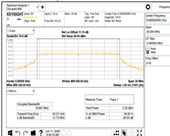
802.11ax_20MHz_Chain1_6895MHz
