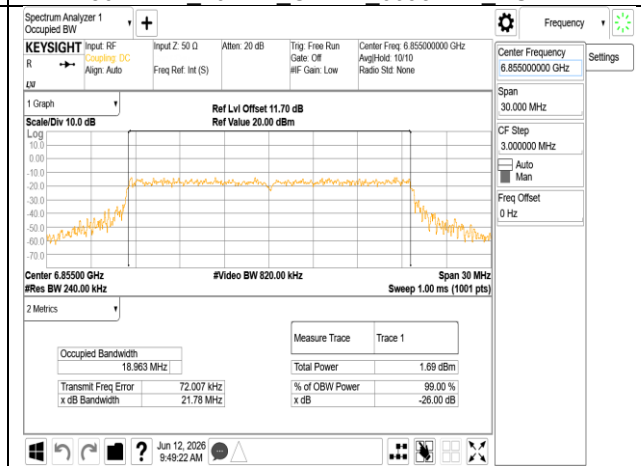
802.11ax 20MHz Chain1 6855MHz RU242
