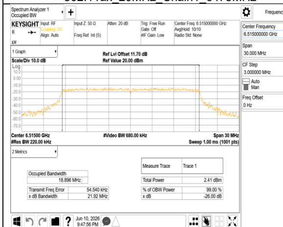
802.11ax 20MHz Chain1 6515MHz
