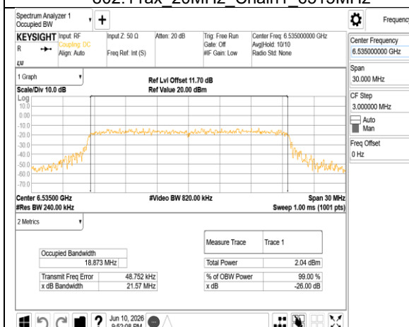
802.11ax 20MHz Chain1 6535MHz
